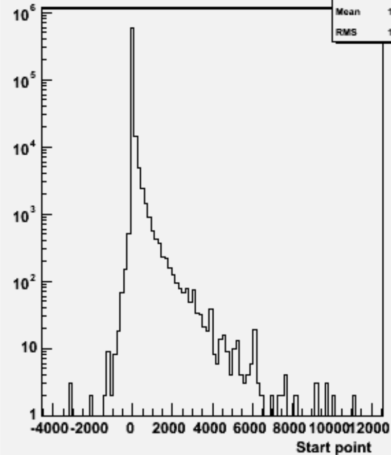
Start point Z : w103327 e1a_e1uubb_o
