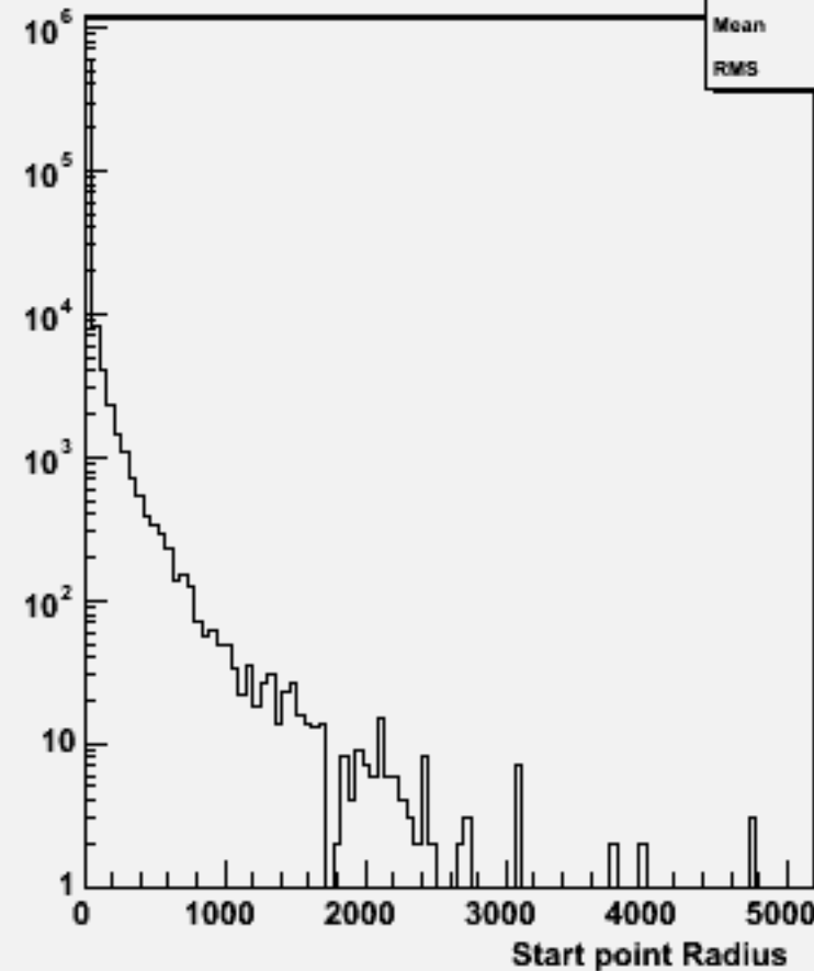
Start point R : w103327 e1a_e1uubb_o
