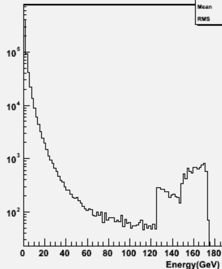
Start point R : w103327 e1a_e1uubb_o
