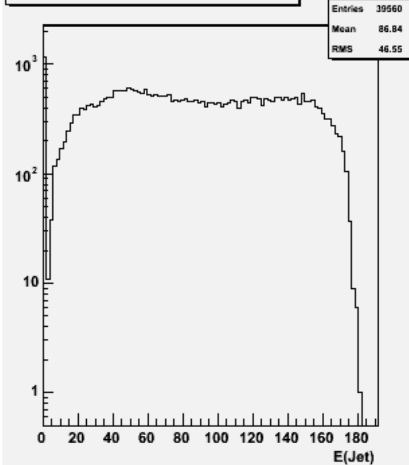
Jet energies(All jets)w103324 e1a_e1uuss_o
