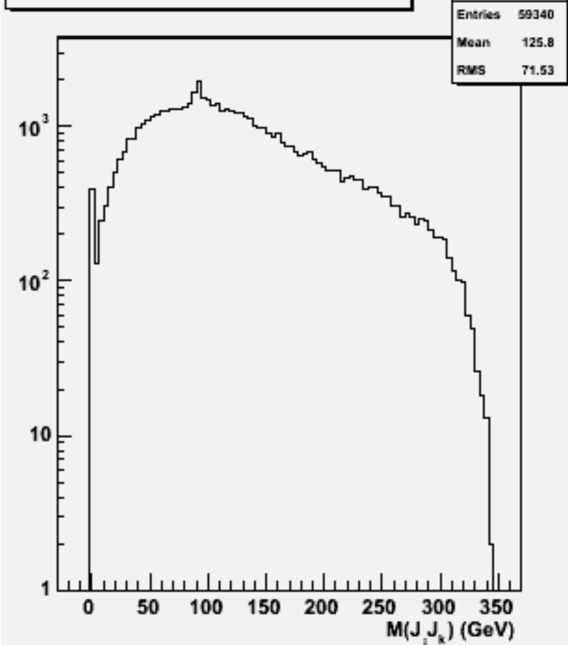
2jets mass(All comb)w103324 e1a_e1uuss_o
