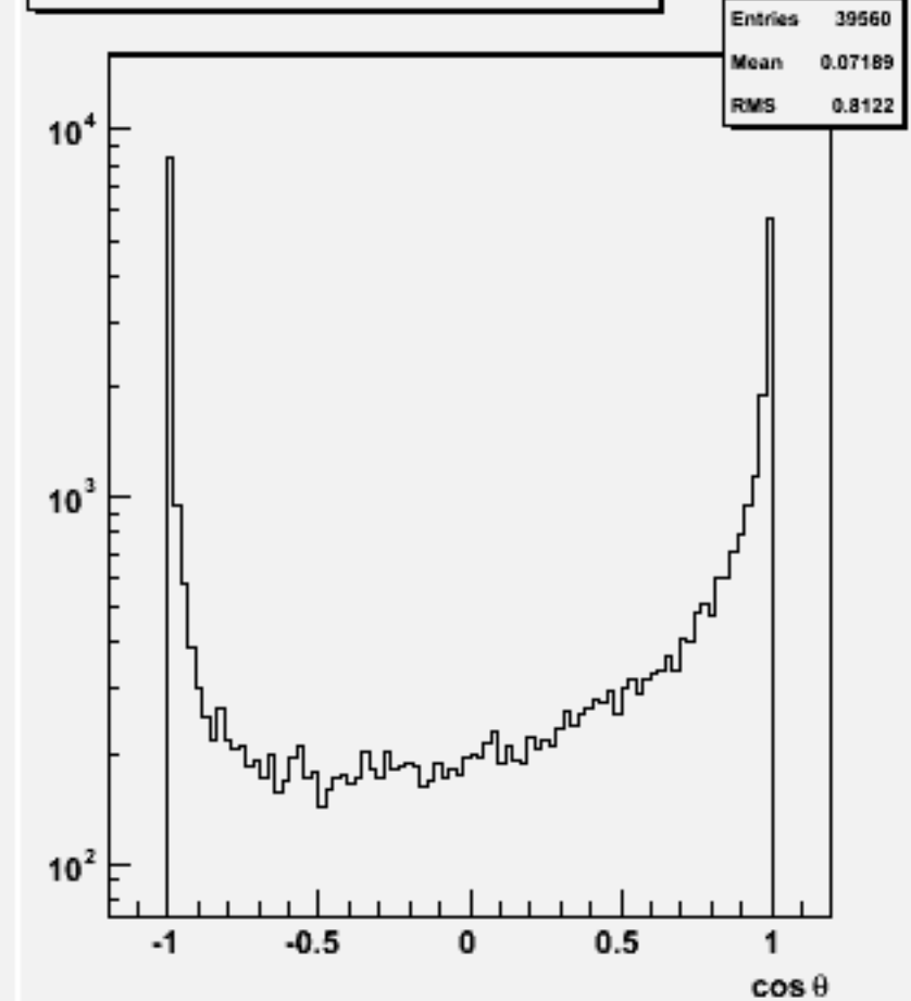
Jet cos \theta (All jets)w103324 e1a_e1uuss_o
