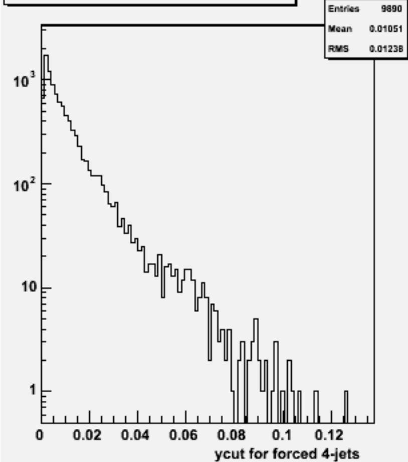
Ycut for 4-jets :w103324 e1a_e1uuss_o
