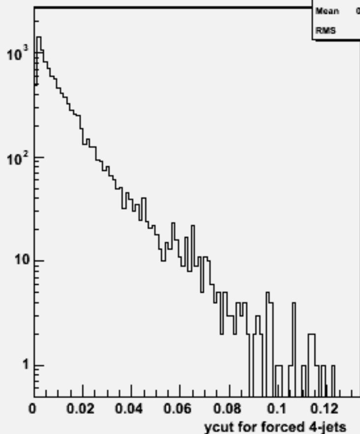
Ycut for 4-jets :w103322 e1a_e1uuss_o
