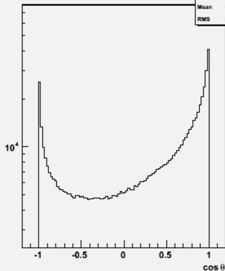
Particle cosθ : w103322 e1a_e1uuss_o
