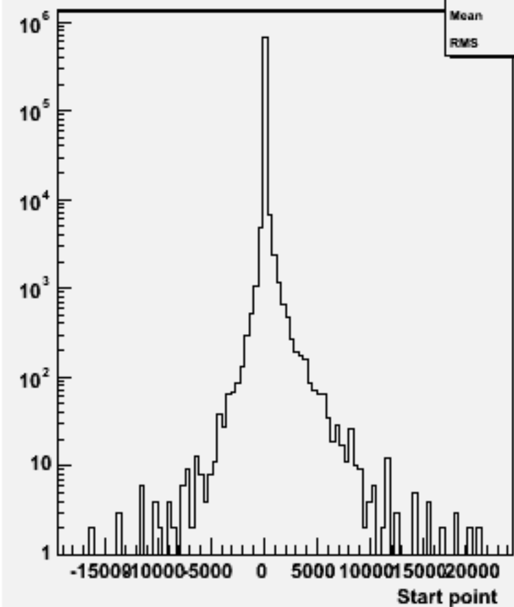
Start point Z : w103322 e1a_e1uuss_o
