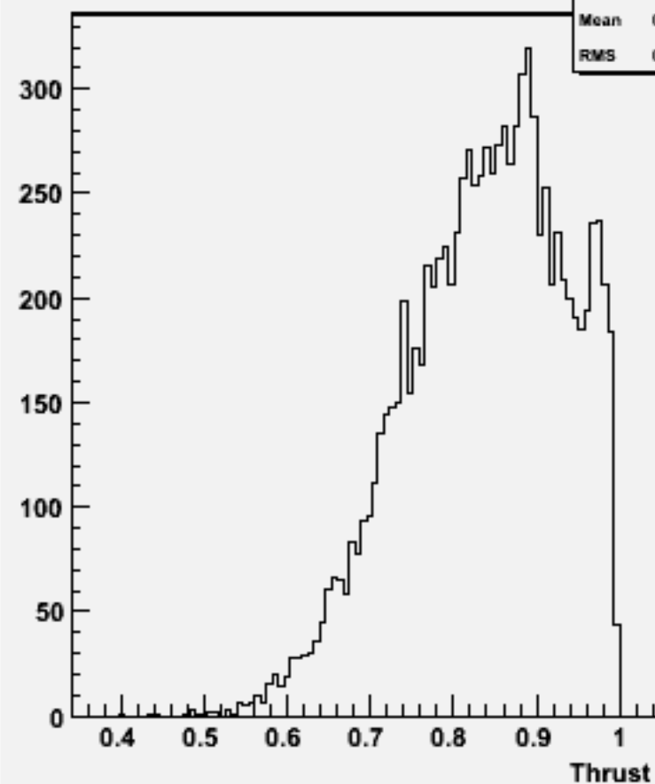
Thrust w103322 e1a_e1uuss_o
