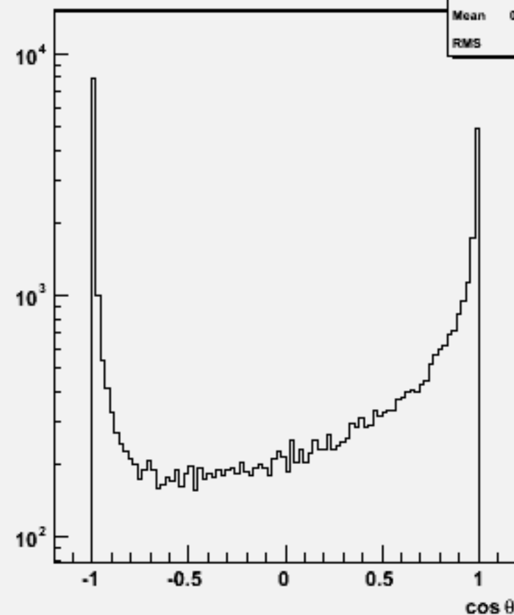
Jet cos \theta (All jets)w103322 e1a_e1uuss_o
