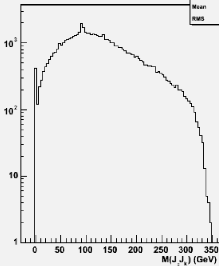
2jets mass(All comb)w103322 e1a_e1uuss_o
