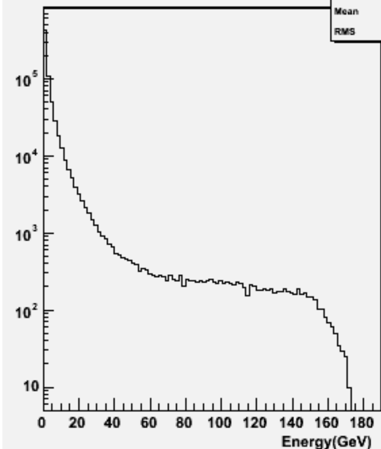
Start point R : w103322 e1a_e1uuss_o
