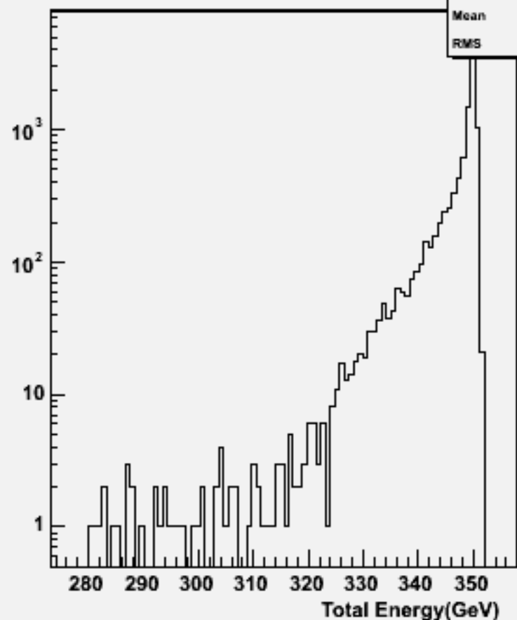
Pt Sum: w103322 e1a_e1uuss_o
