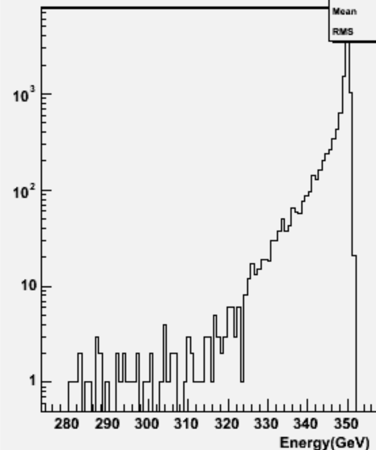
Thrust w103322 e1a_e1uuss_o
