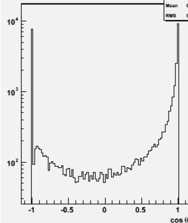
Jet cos \theta (All jets)w103319 e1a_e1uue3e3_o
