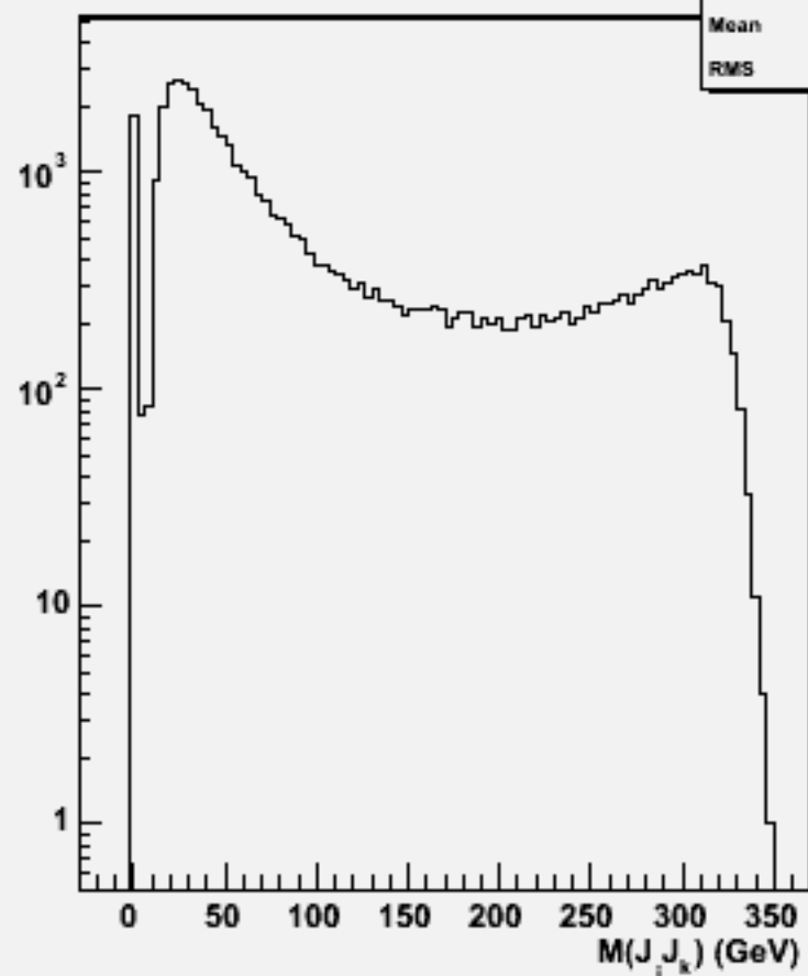
2jets mass(All comb)w103319 e1a_e1uue3e3_o
