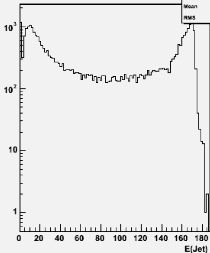
Jet energies(All jets)w103319 e1a_e1uue3e3_o
