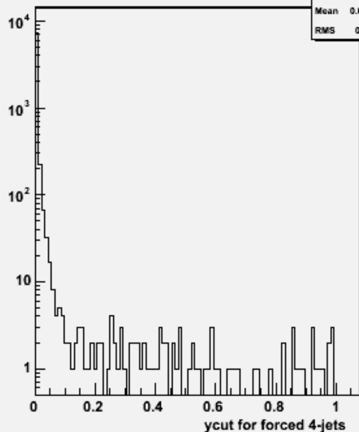
Ycut for 4-jets :w103319 e1a_e1uue3e3_o
