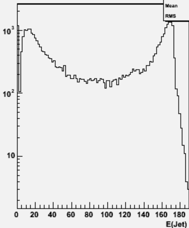
Jet energies(All jets)w103315 e1a_e1uue2e2_o
