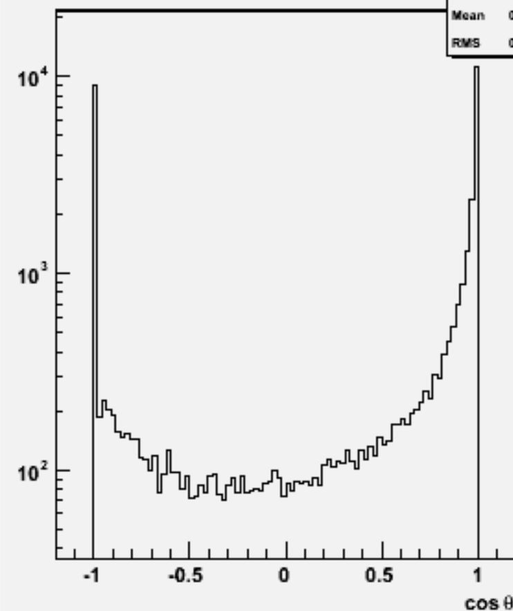
Jet cos \theta (All jets)w103315 e1a_e1uue2e2_o
