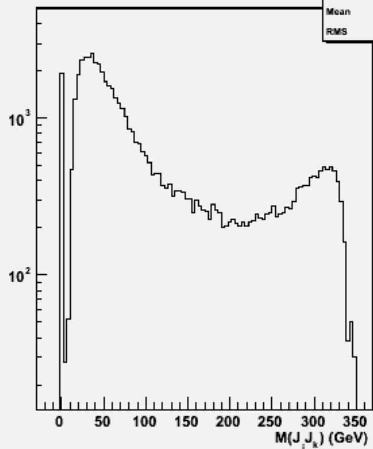
2jets mass(All comb)w103315 e1a_e1uue2e2_o
