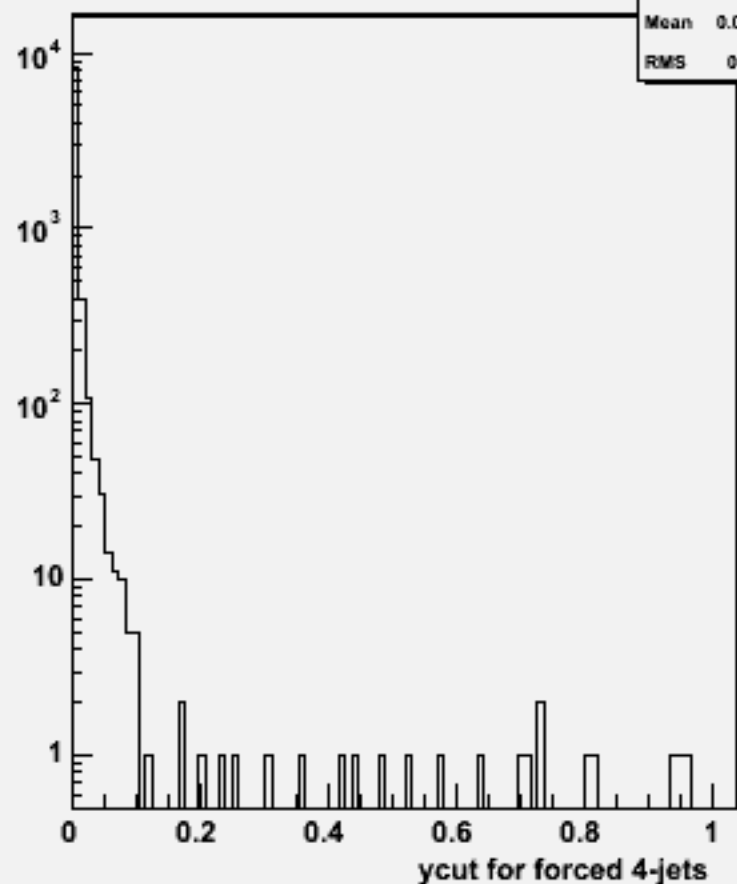
Ycut for 4-jets :w103315 e1a_e1uue2e2_o
