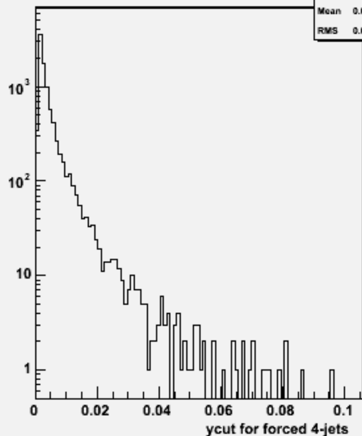
Ycut for 4-jets :w103314 e1a_e1uue2e2_o
