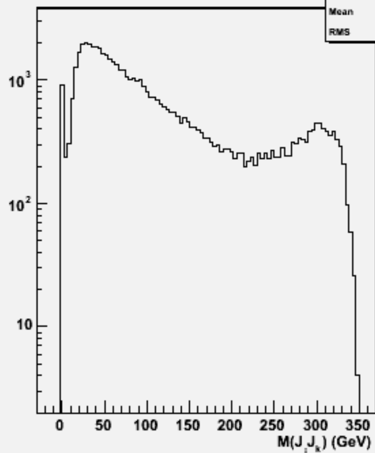
2jets mass(All comb)w103314 e1a_e1uue2e2_o
