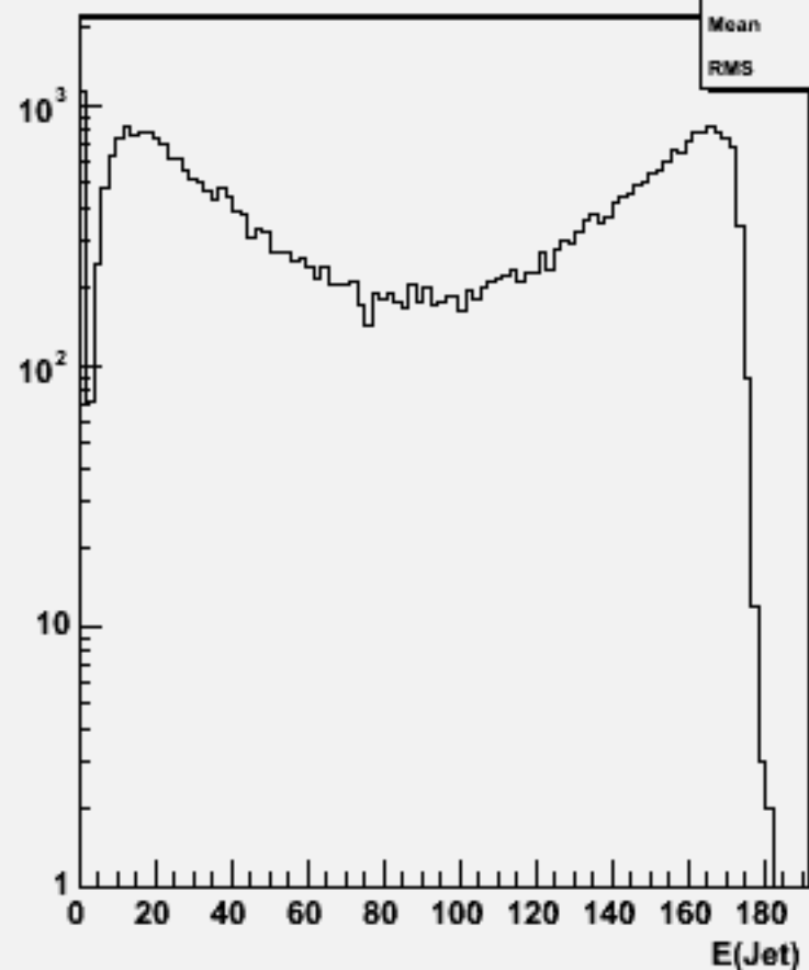
Jet energies(All jets)w103314 e1a_e1uue2e2_o
