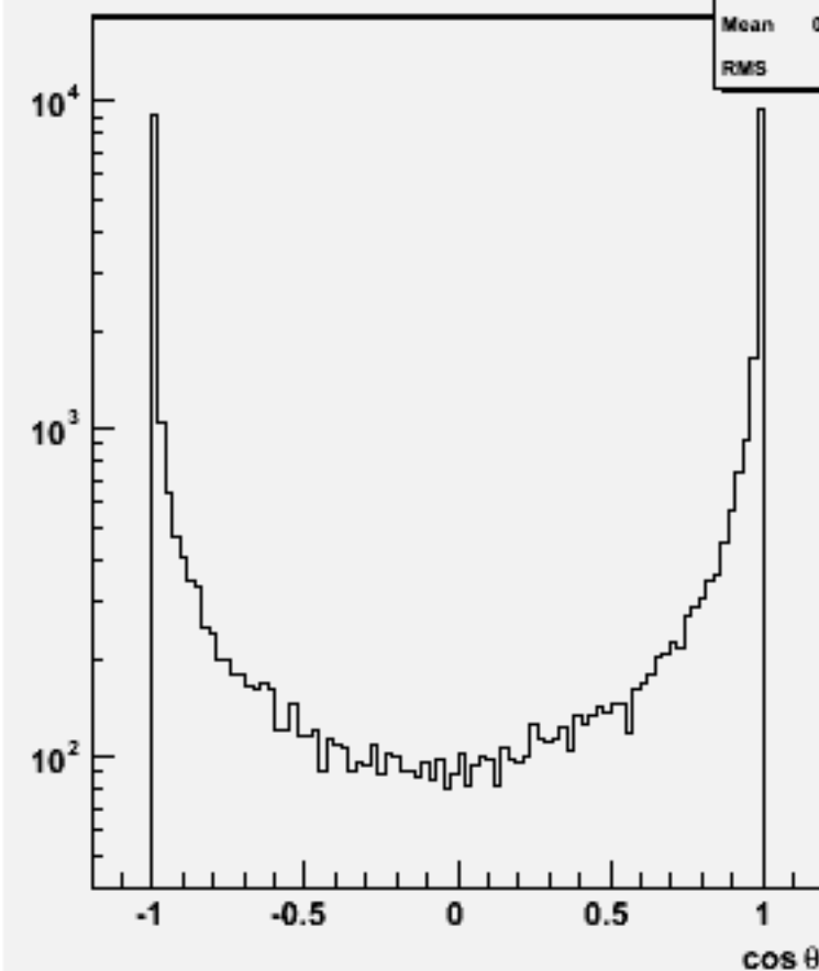
Jet cos \theta (All jets)w103314 e1a_e1uue2e2_o
