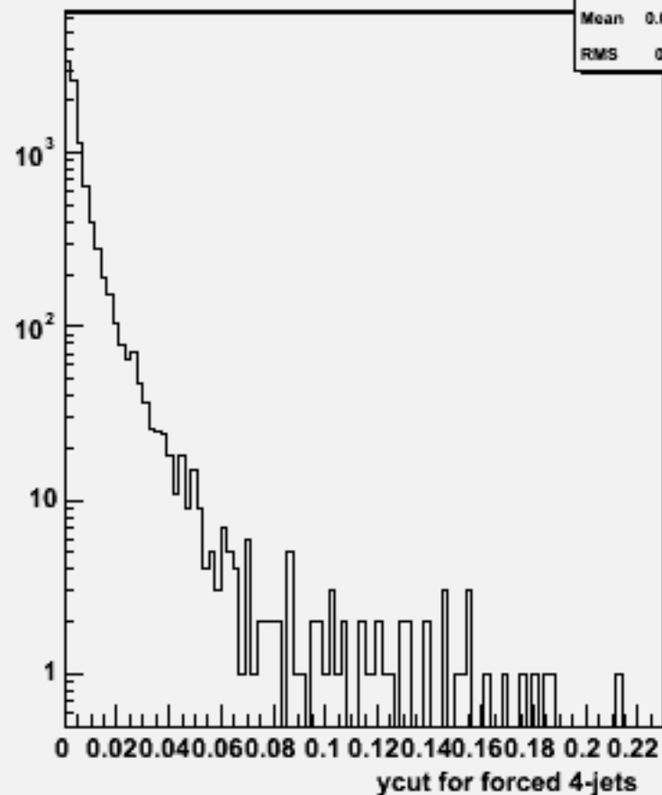
Ycut for 4-jets :w103304 e1a_e1n3n3ss_o
