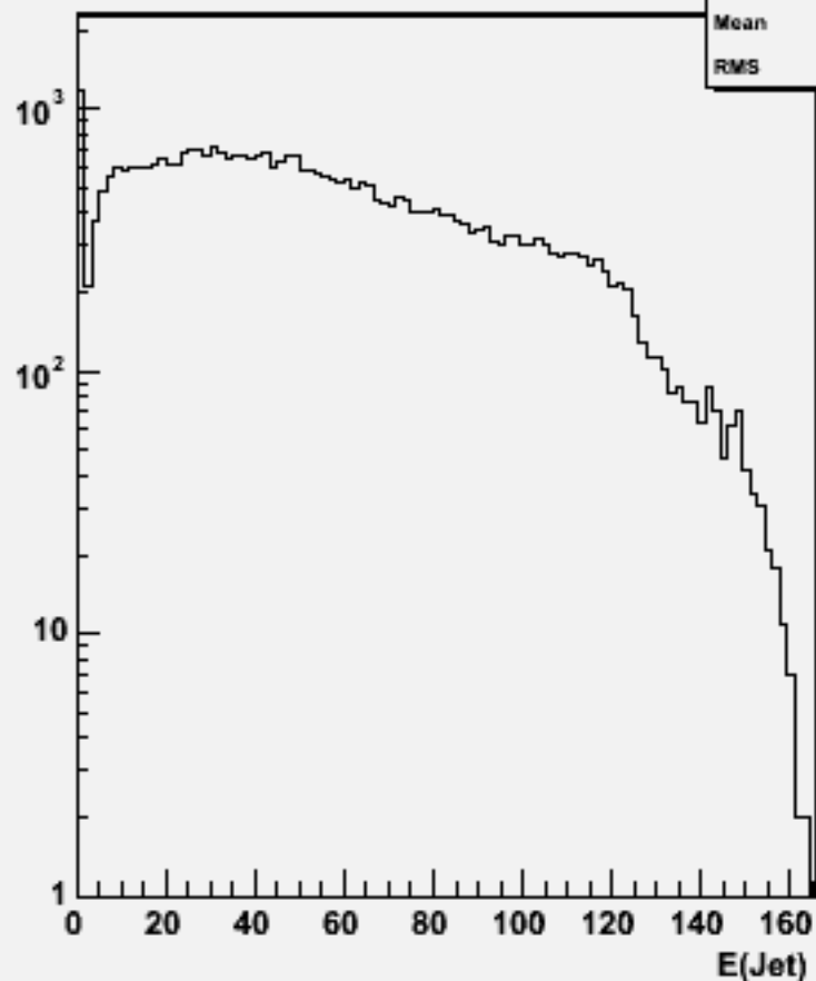
Jet energies(All jets)w103304 e1a_e1n3n3ss_o
