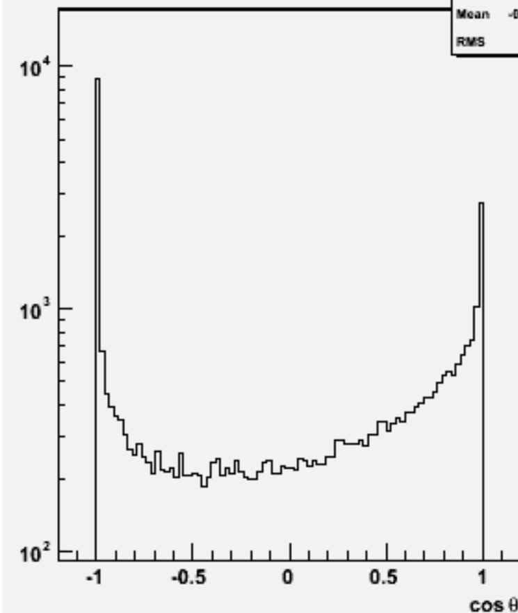
Jet cos \theta (All jets)w103304 e1a_e1n3n3ss_o
