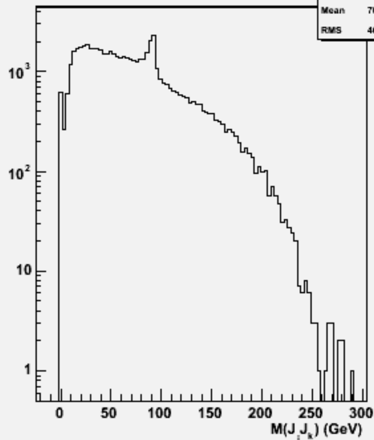
2jets mass(All comb)w103304 e1a_e1n3n3ss_o
