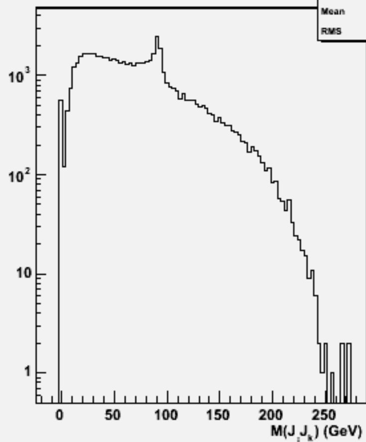
2jets mass(All comb)w103302 e1a_e1n3n3ss_o
