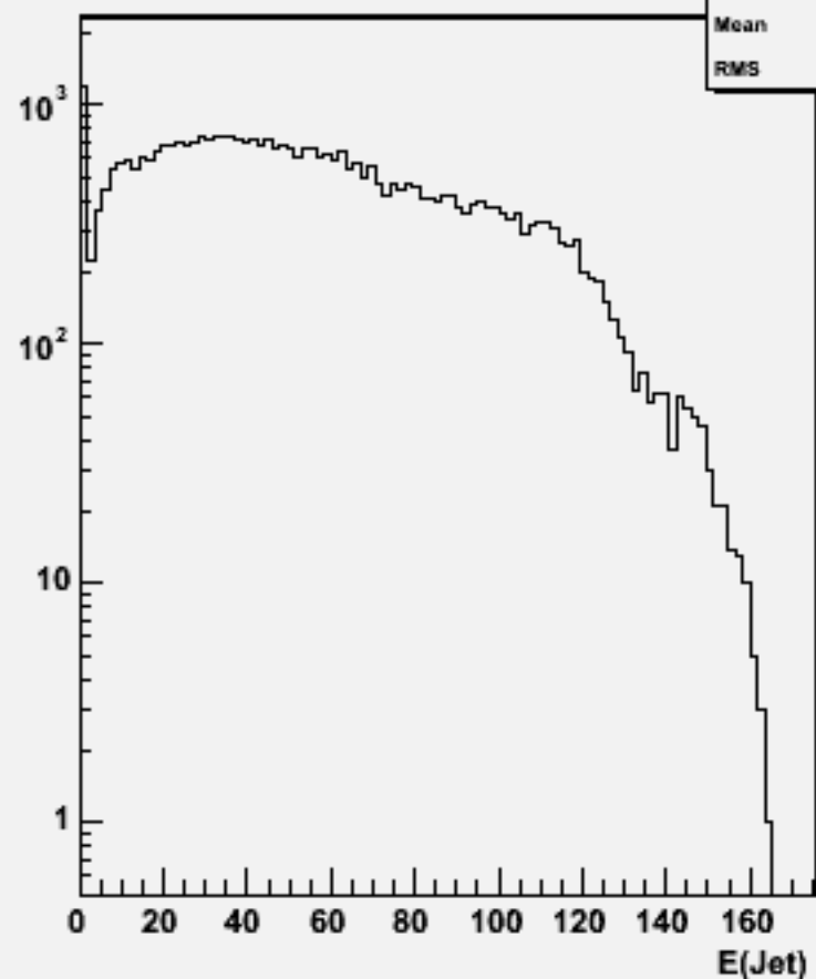
Jet energies(All jets)w103302 e1a_e1n3n3ss_o
