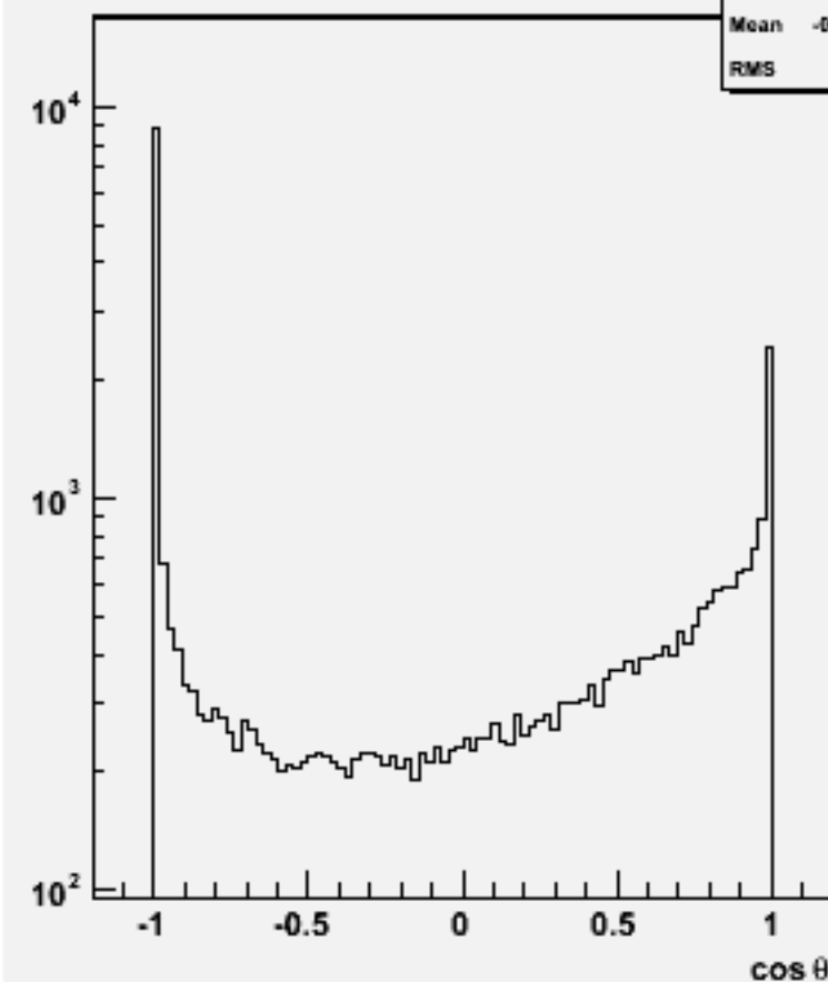
Jet cos \theta (All jets)w103302 e1a_e1n3n3ss_o
