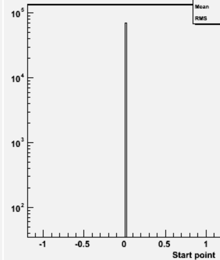
Start point Z : w103294 e1a_e1n3n3e2e2_o
