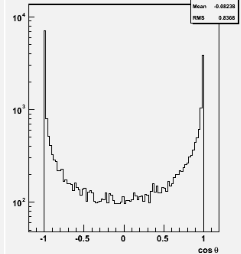
Jet cos \theta (All jets)w103294 e1a_e1n3n3e2e2_o
