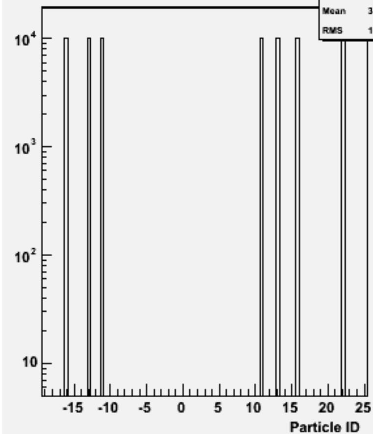
Particle ID : w103294 e1a_e1n3n3e2e2_o
