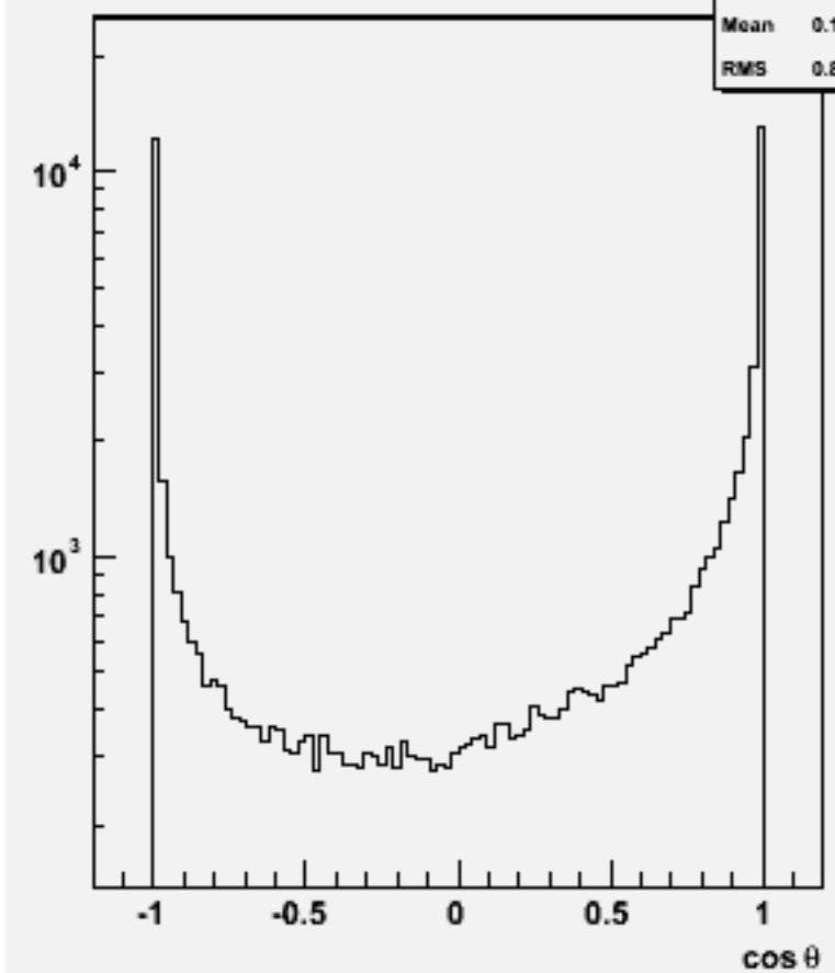
Particle cos \theta : w103294 e1a_e1n3n3e2e2_o
