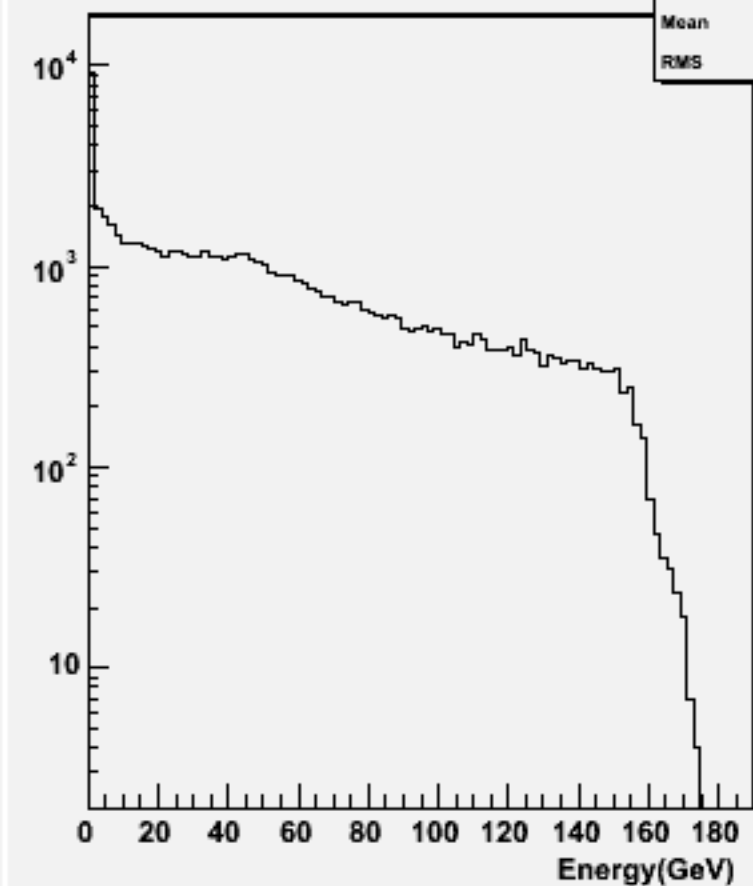
Particle Energy : w103294 e1a_e1n3n3e2e2_o
