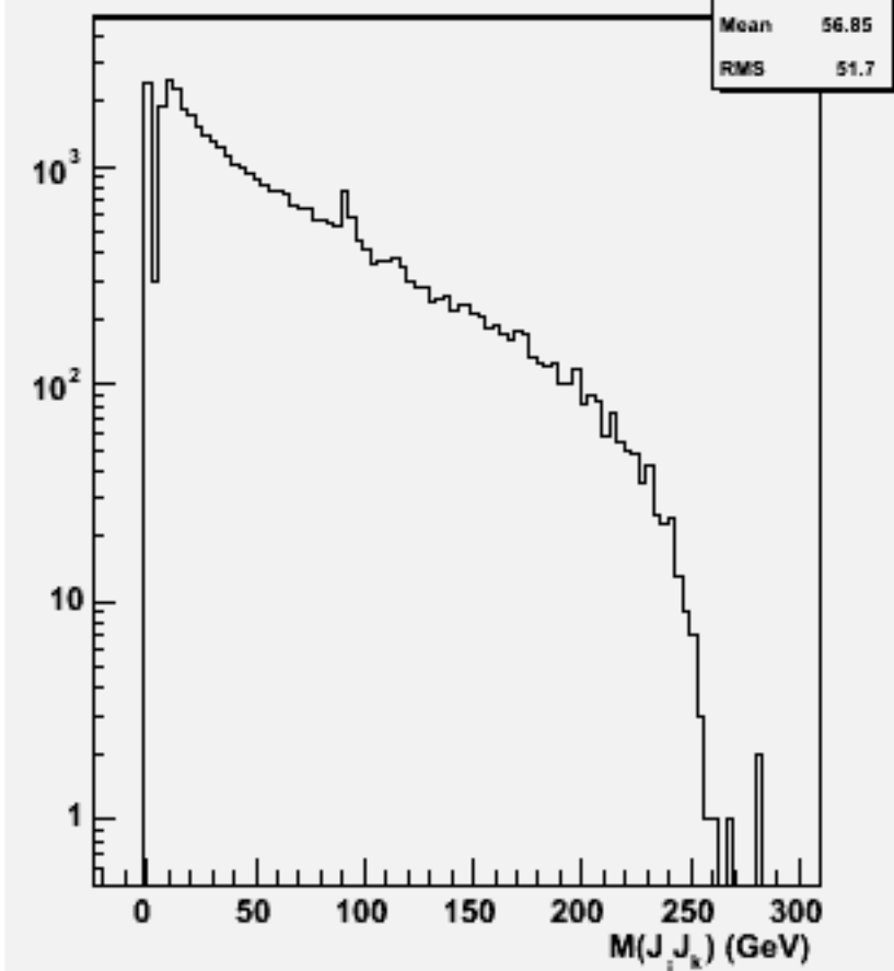
2jets mass(All comb)w103294 e1a_e1n3n3e2e2_o
