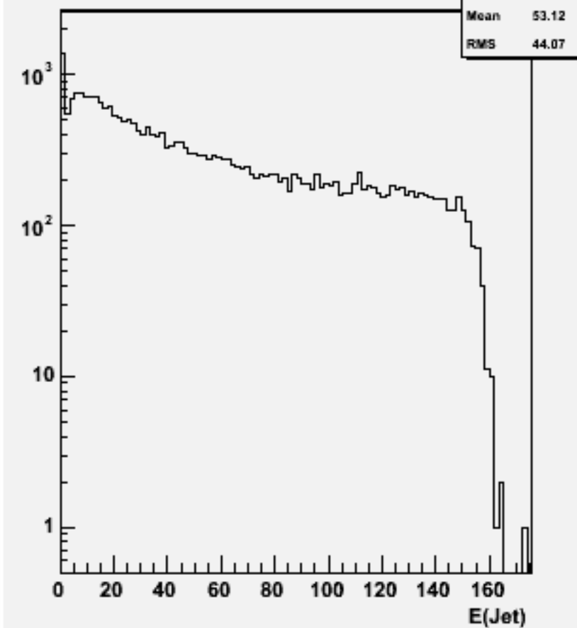
Jet energies(All jets)w103294 e1a_e1n3n3e2e2_o
