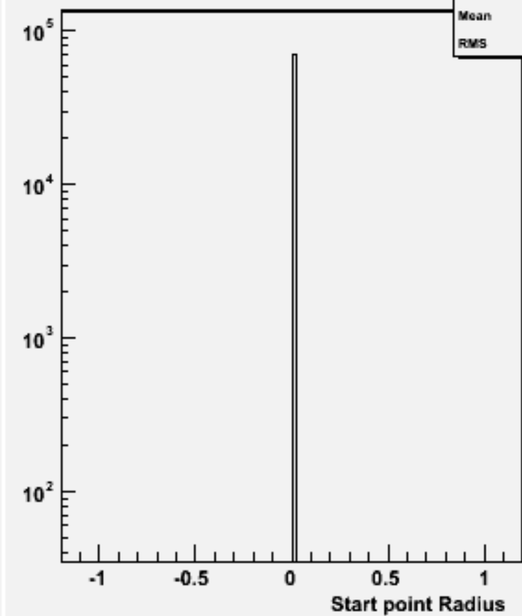
Start point R : w103294 e1a_e1n3n3e2e2_o
