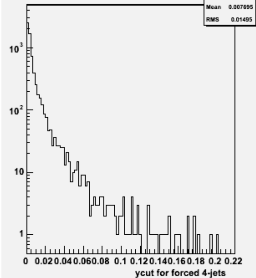
Ycut for 4-jets :w103294 e1a_e1n3n3e2e2_o
