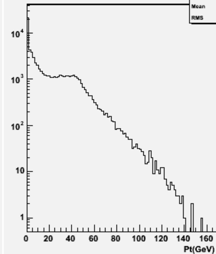
Particle Pt : w103294 e1a_e1n3n3e2e2_o
