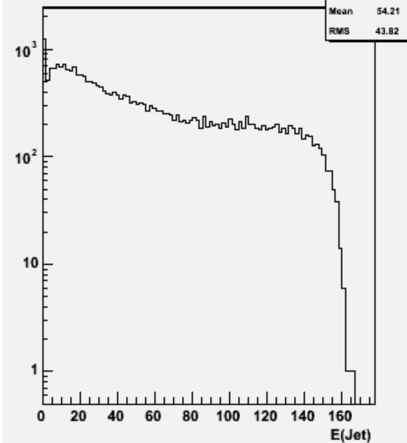
Jet energies(All jets)w103292 e1a_e1n3n3e1e1_o
