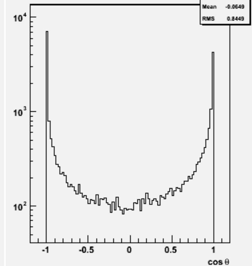
Jet cos \theta (All jets)w103292 e1a_e1n3n3e1e1_o
