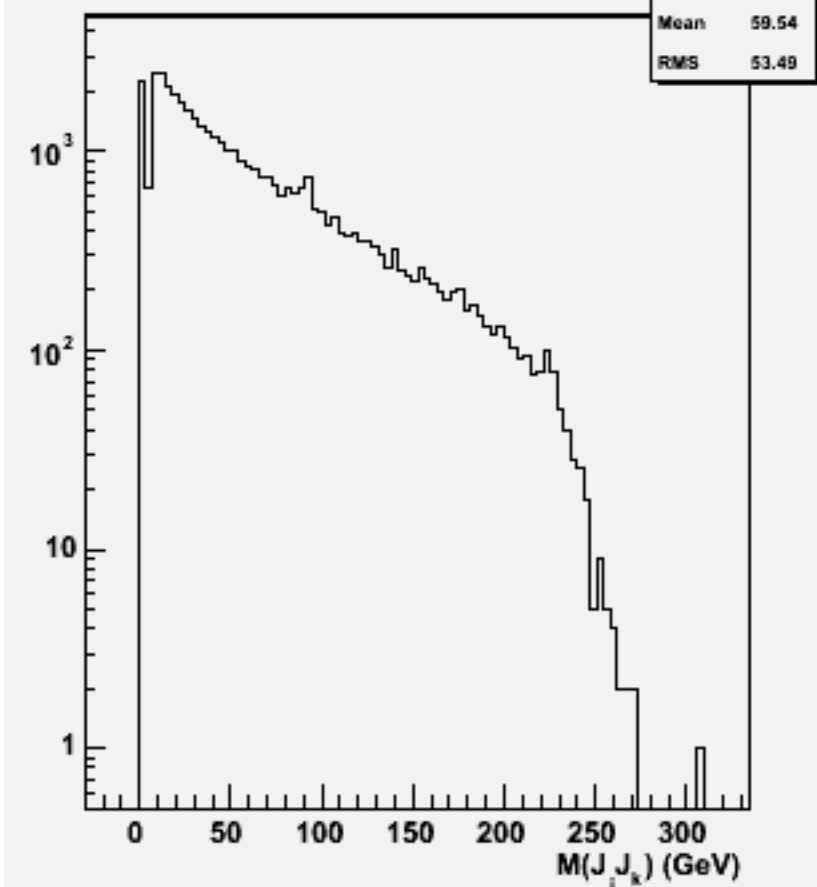
2jets mass(All comb)w103292 e1a_e1n3n3e1e1_o
