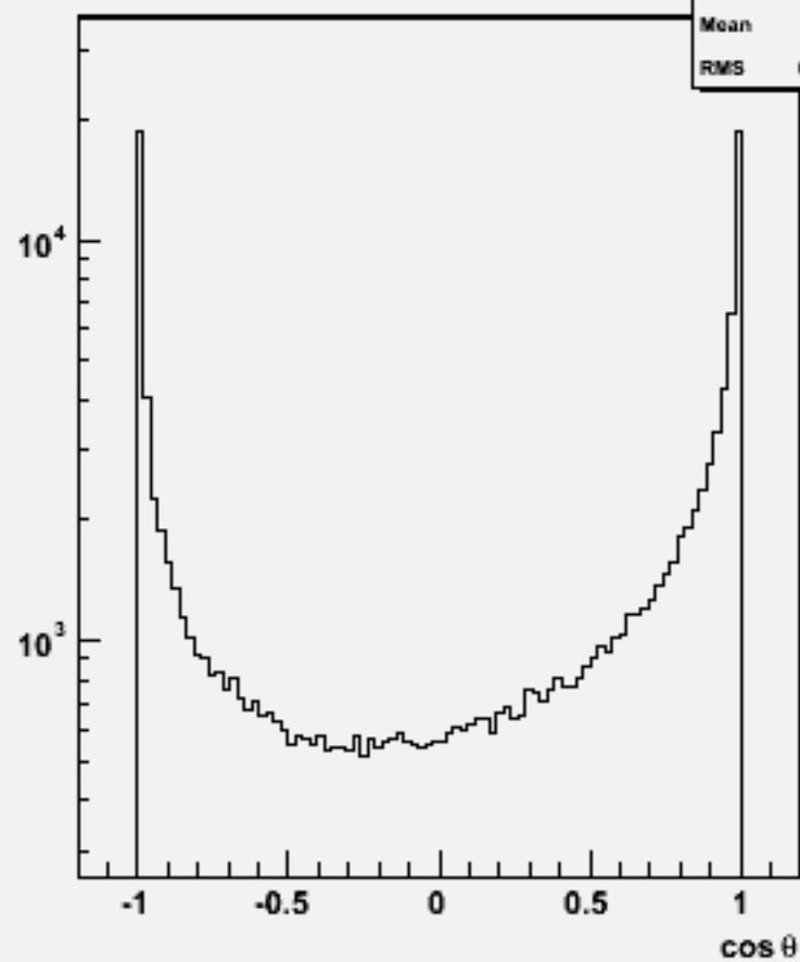
Particle cos \theta : w103276 e1a_e1n2n2e3e3_o
