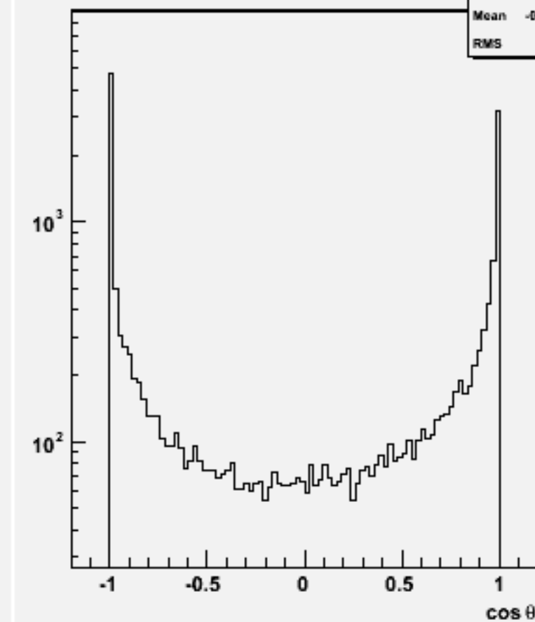
Jet cos \theta (All jets)w103276 e1a_e1n2n2e3e3_o
