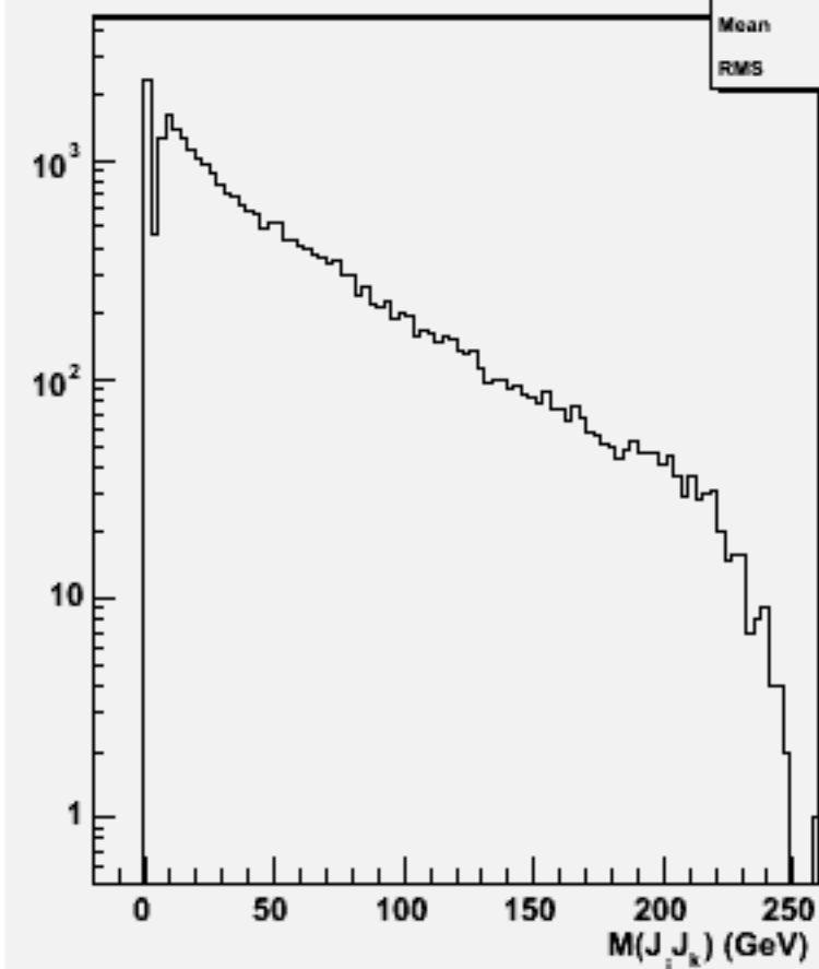
2jets mass(All comb)w103276 e1a_e1n2n2e3e3_o
