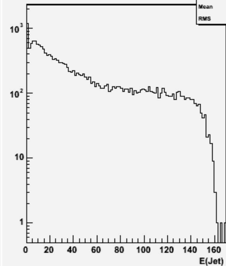
Jet energies(All jets)w103276 e1a_e1n2n2e3e3_o
