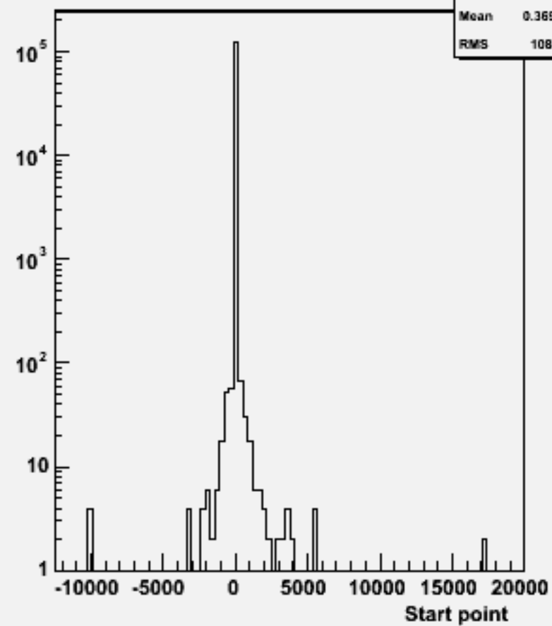
Start point Z : w103276 e1a_e1n2n2e3e3_o
