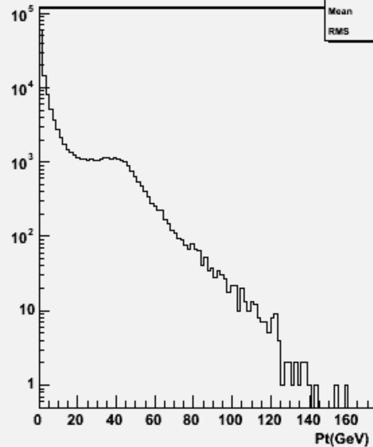
Start point Z : w103276 e1a_e1n2n2e3e3_o
