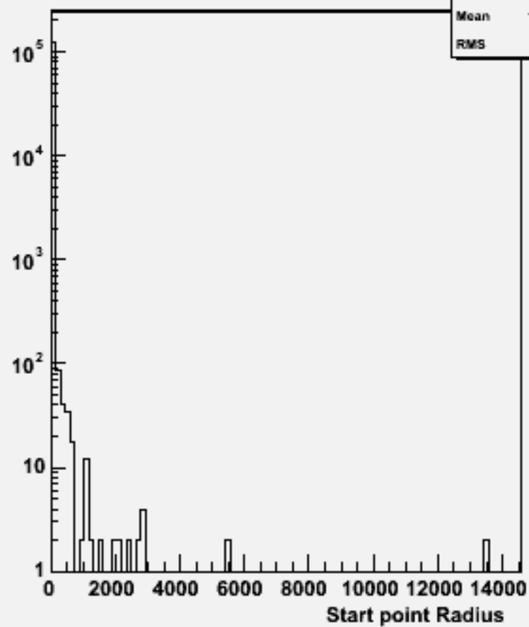
Start point R : w103276 e1a_e1n2n2e3e3_o
