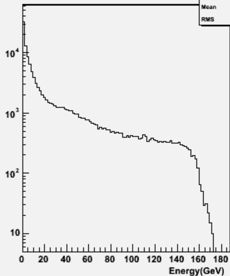
Start point R : w103276 e1a_e1n2n2e3e3_o
