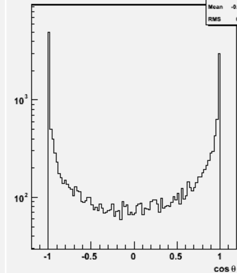
Jet cos \theta (All jets)w103274 e1a_e1n2n2e3e3_o
