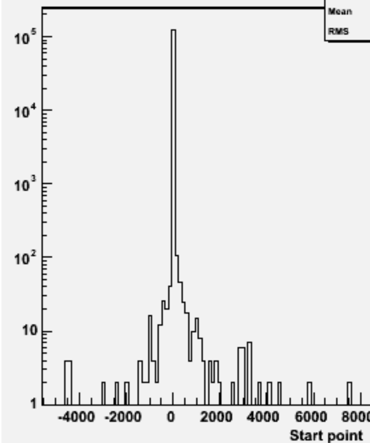
Start point Z : w103274 e1a_e1n2n2e3e3_o
