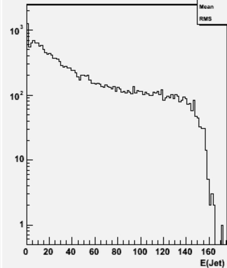
Jet energies(All jets)w103274 e1a_e1n2n2e3e3_o
