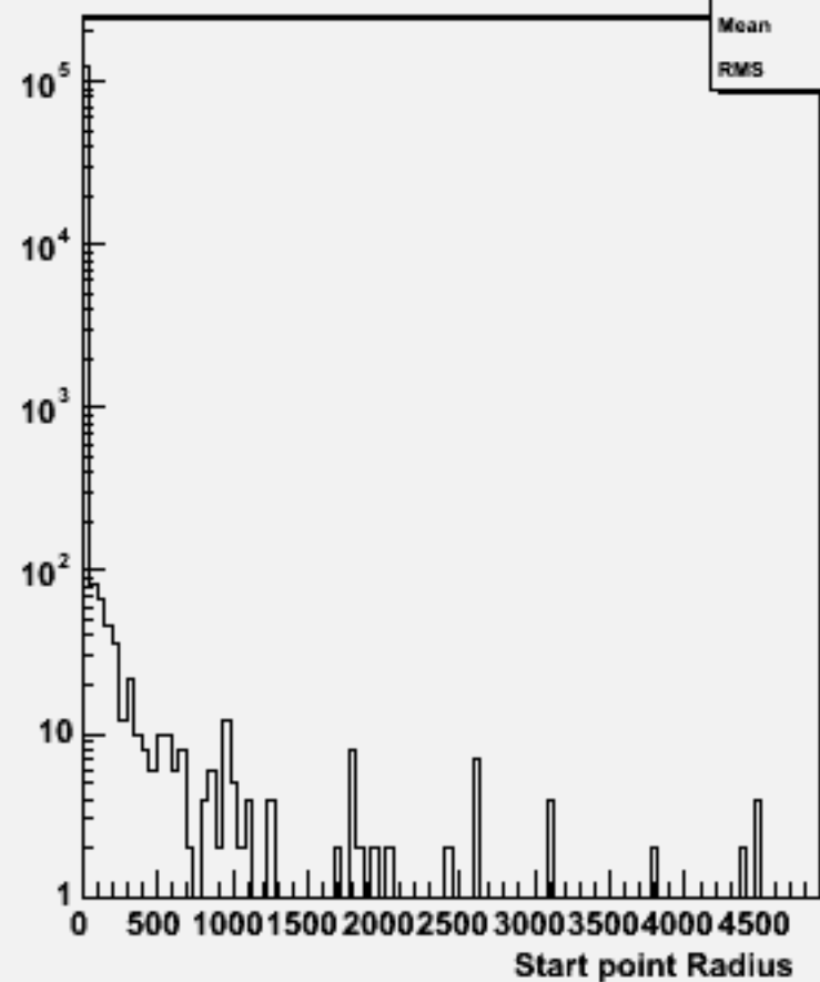
Start point R : w103274 e1a_e1n2n2e3e3_o
