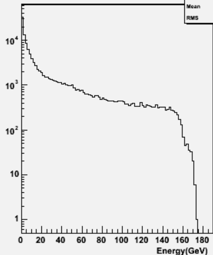
Start point R : w103274 e1a_e1n2n2e3e3_o
