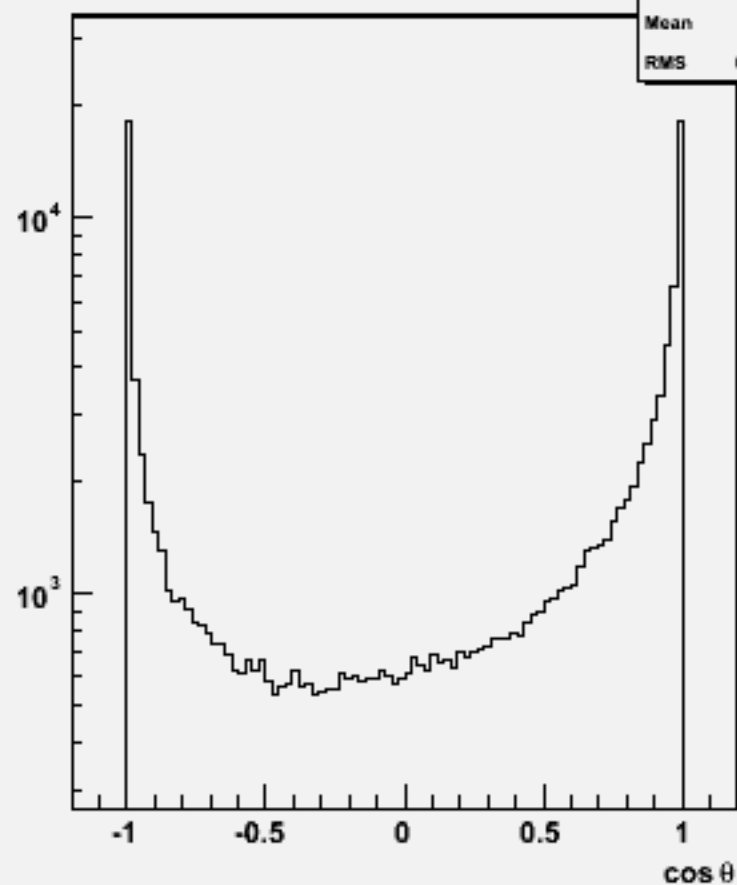
Particle cos \theta : w103274 e1a_e1n2n2e3e3_o
