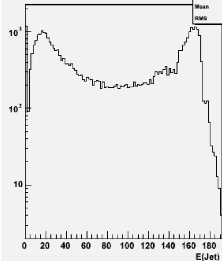
Jet energies(All jets)w103269 e1a_e1cccc_o
