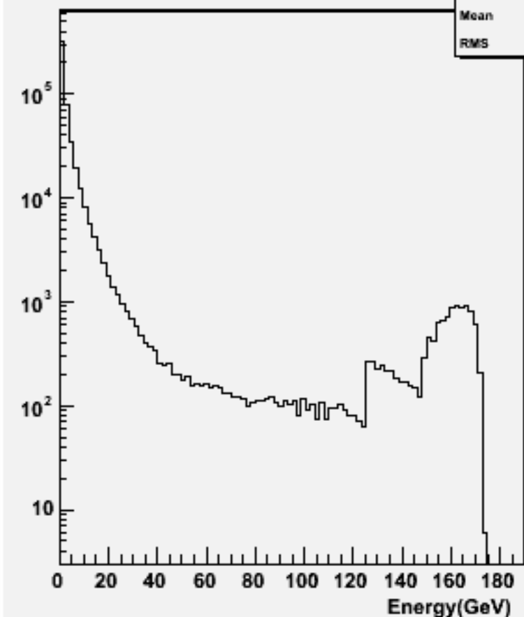
Start point R : w103269 e1a_e1cccc_o
