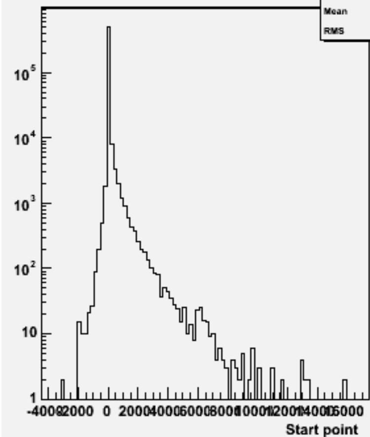
Start point Z : w103269 e1a_e1cccc_o
