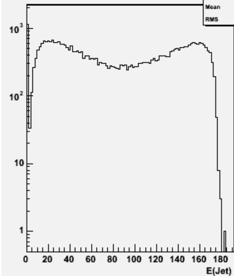
Jet energies(All jets)w103268 e1a_e1cccc_o
