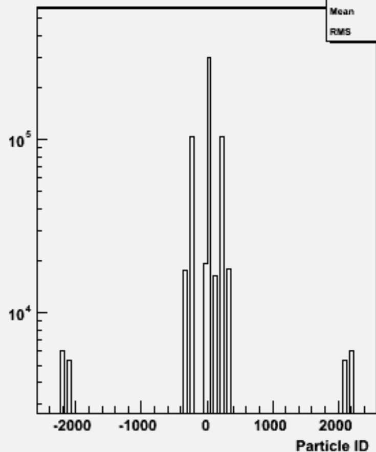
Particle ID : w103268 e1a_e1cccc_o
