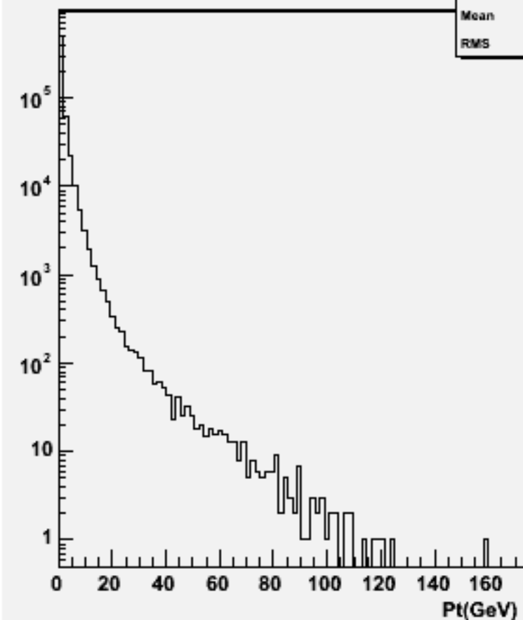
Particle Pt : w103268 e1a_e1cccc_o
