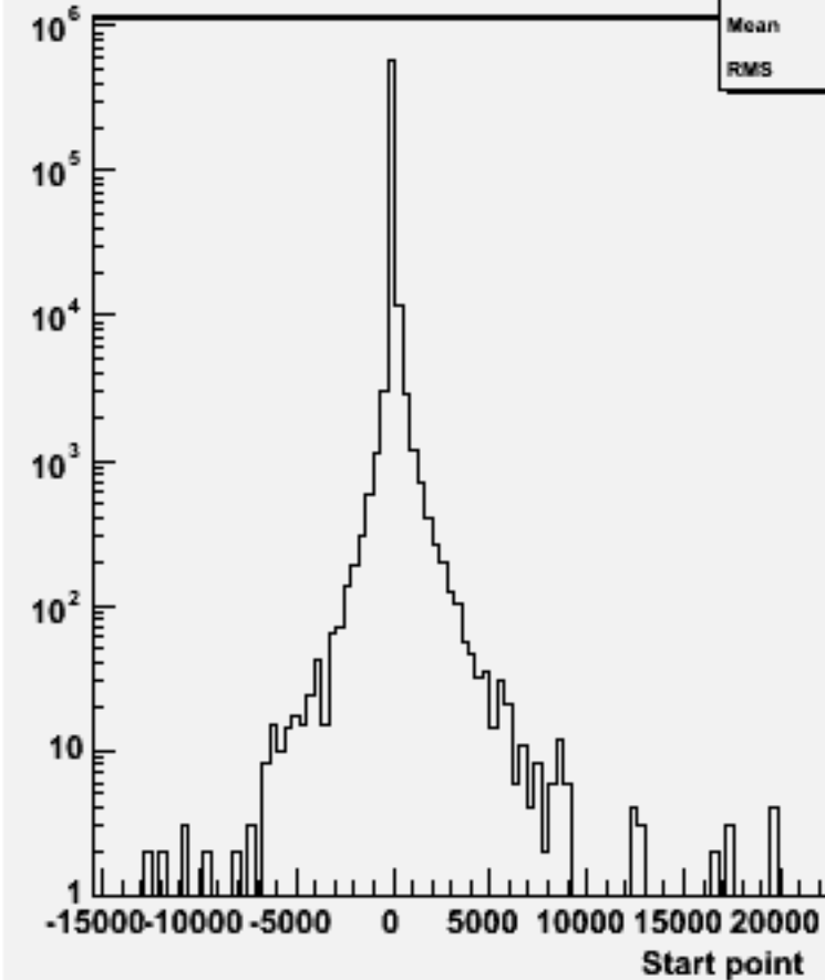
Start point Z : w103268 e1a_e1cccc_o
