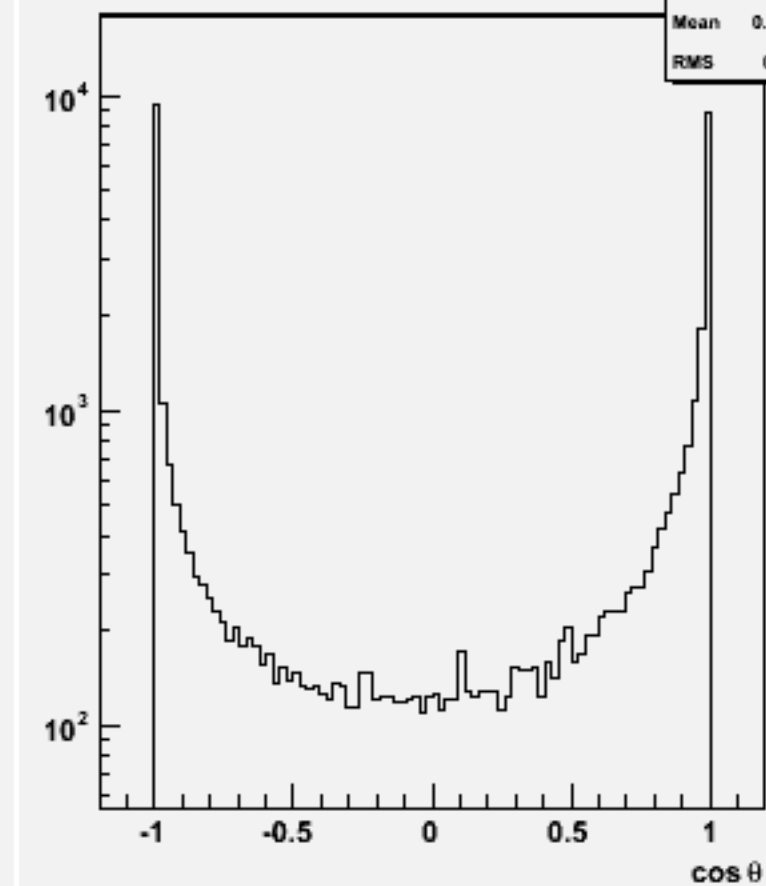
Jet cos \theta (All jets)w103268 e1a_e1cccc_o
