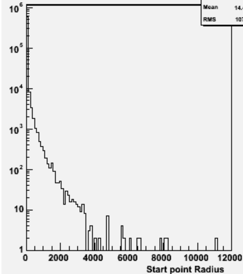
Start point R : w103268 e1a_e1cccc_o
