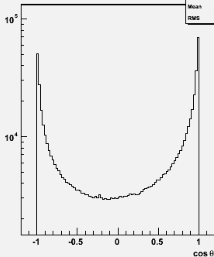
Particle cosθ : w103268 e1a_e1cccc_o
