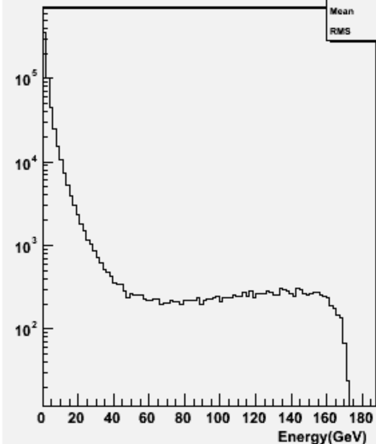
Particle Energy : w103268 e1a_e1cccc_o
