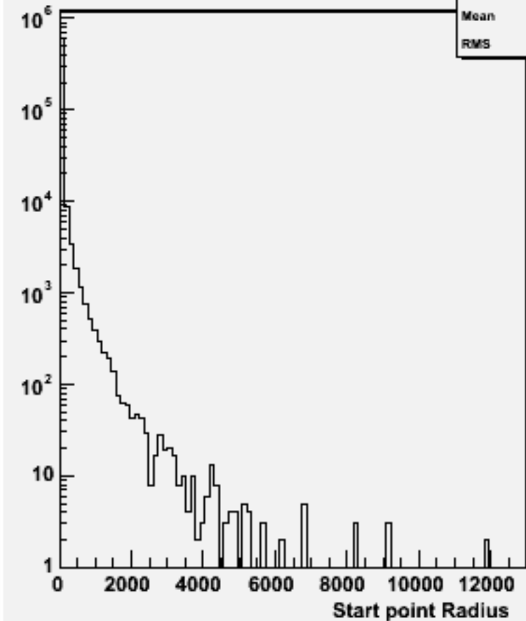
Start point R : w103266 e1a_e1cccc_o
