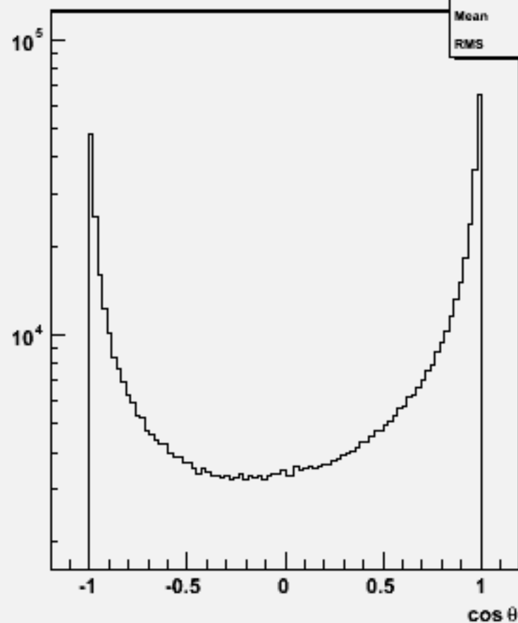
Particle cos \theta : w103266 e1a_e1cccc_o
