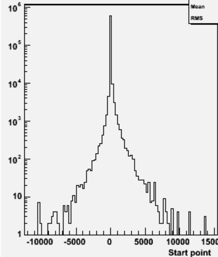
Start point Z : w103266 e1a_e1cccc_o
