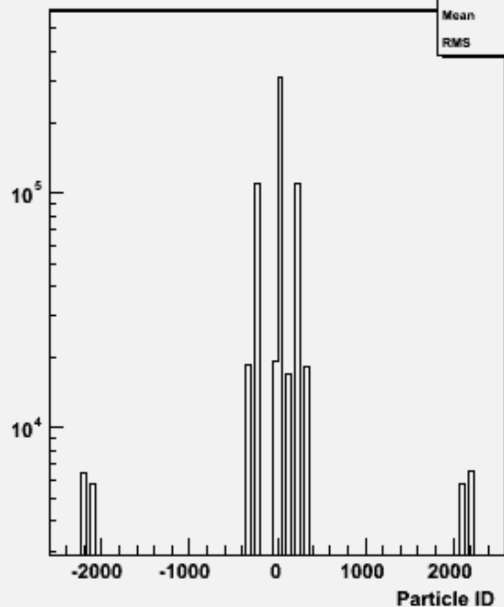
Particle ID : w103266 e1a_e1cccc_o
