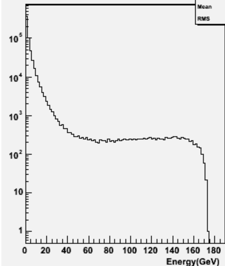
Particle Energy : w103266 e1a_e1cccc_o
