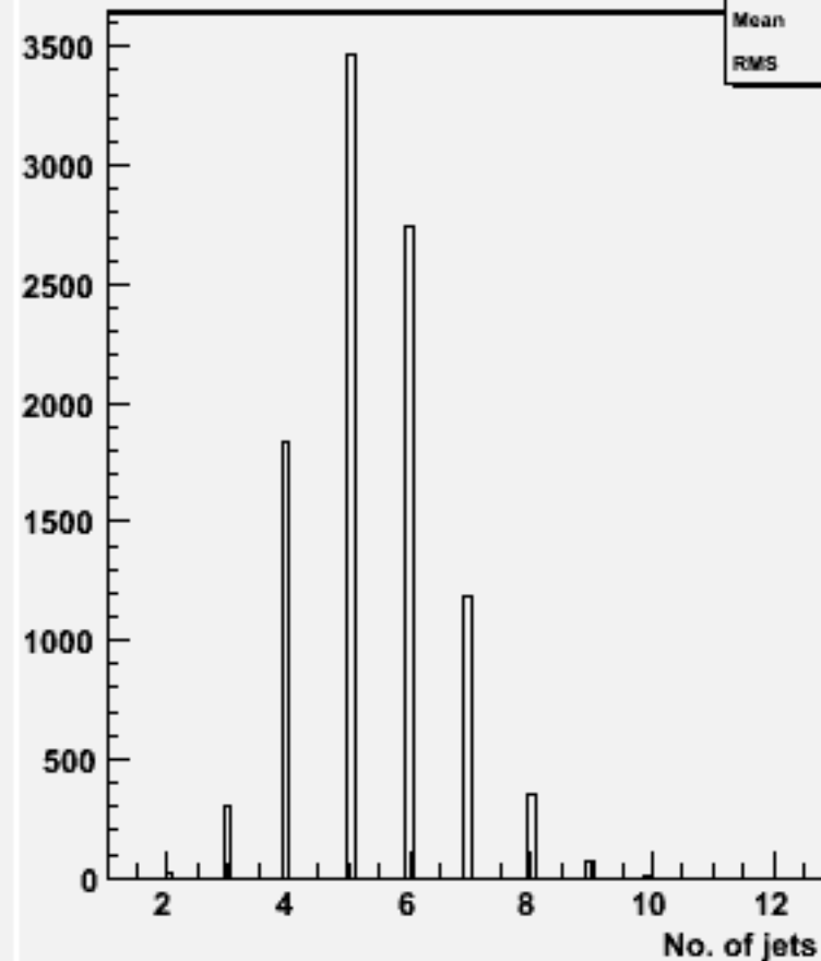
No. jets (ycut=0.001) : w103266 e1a_e1cccc_o
