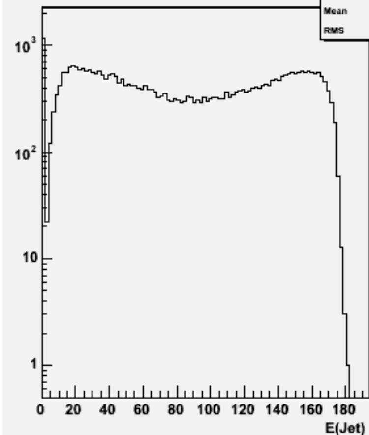
Jet energies(All jets)w103266 e1a_e1cccc_o
