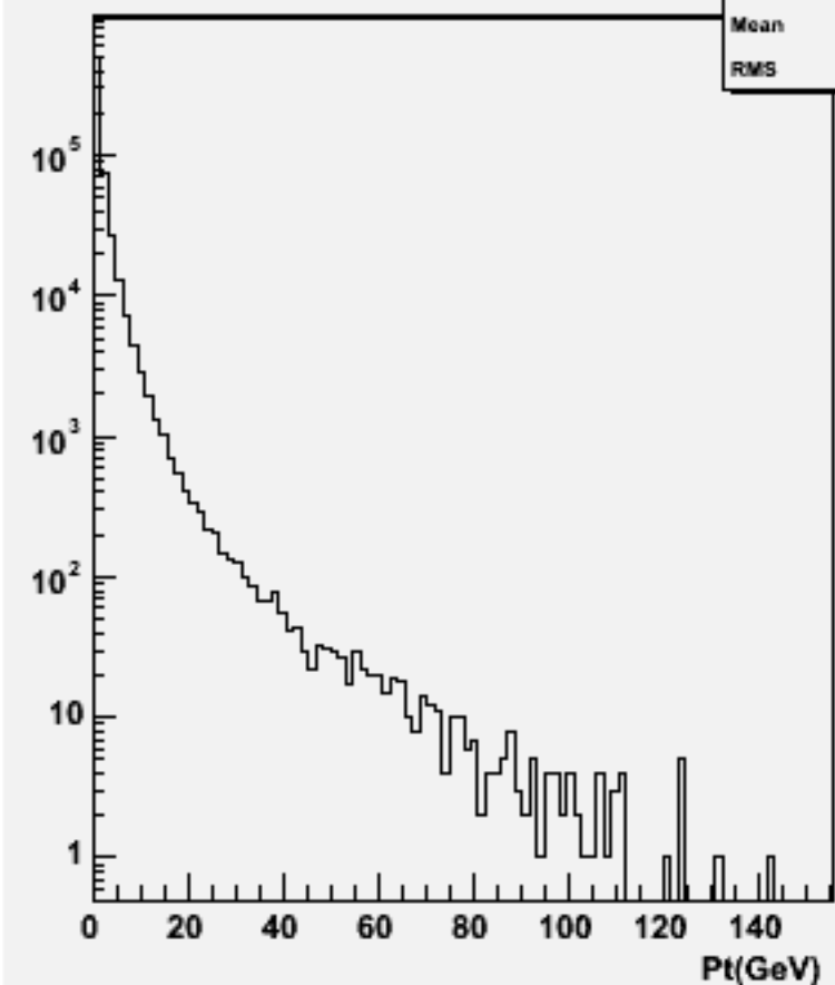
Particle Pt : w103266 e1a_e1cccc_o
