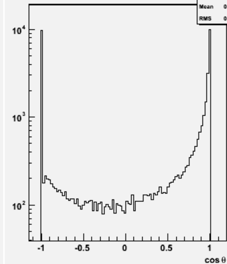
Jet cos \theta (All jets)w103265 e1a_e1uucc_o
