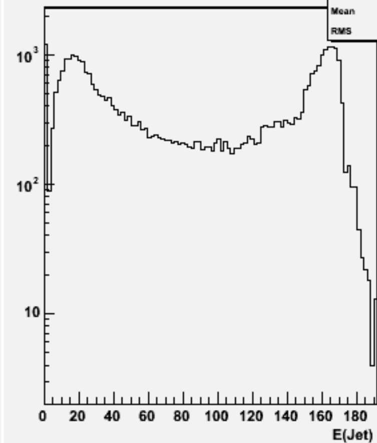
Jet energies(All jets)w103265 e1a_e1uucc_o
