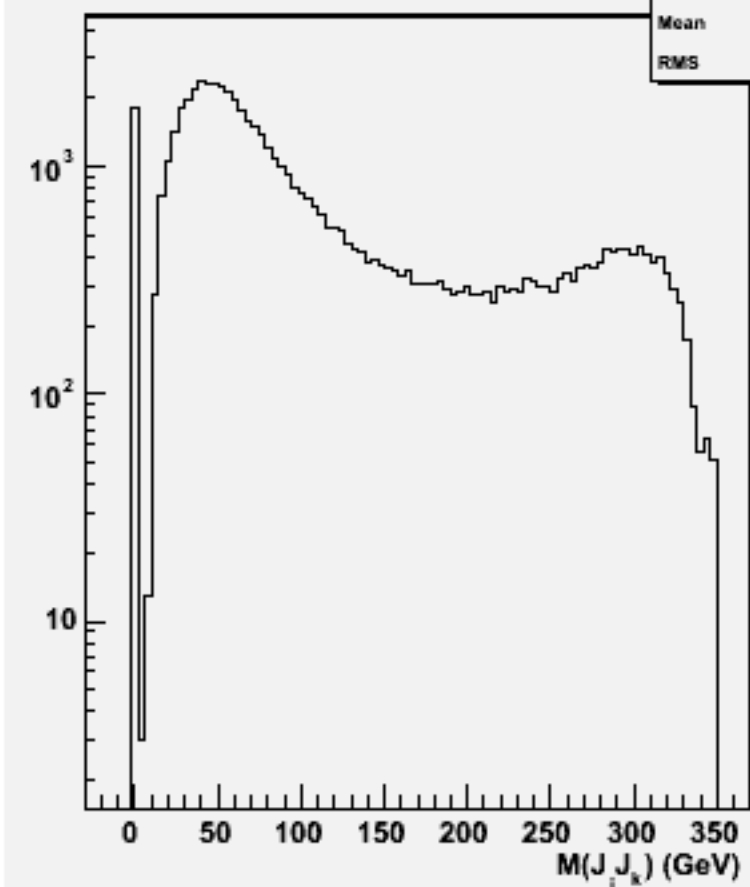
2jets mass(All comb)w103265 e1a_e1uucc_o
