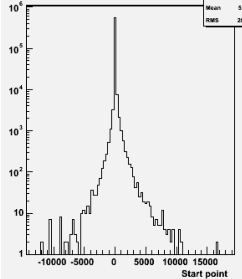
Start point Z : w103264 e1a_e1uucc_o
