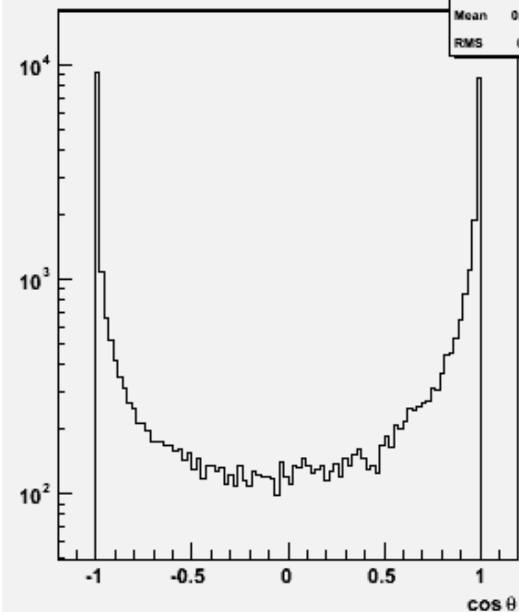
Jet cos \theta (All jets)w103264 e1a_e1uucc_o
