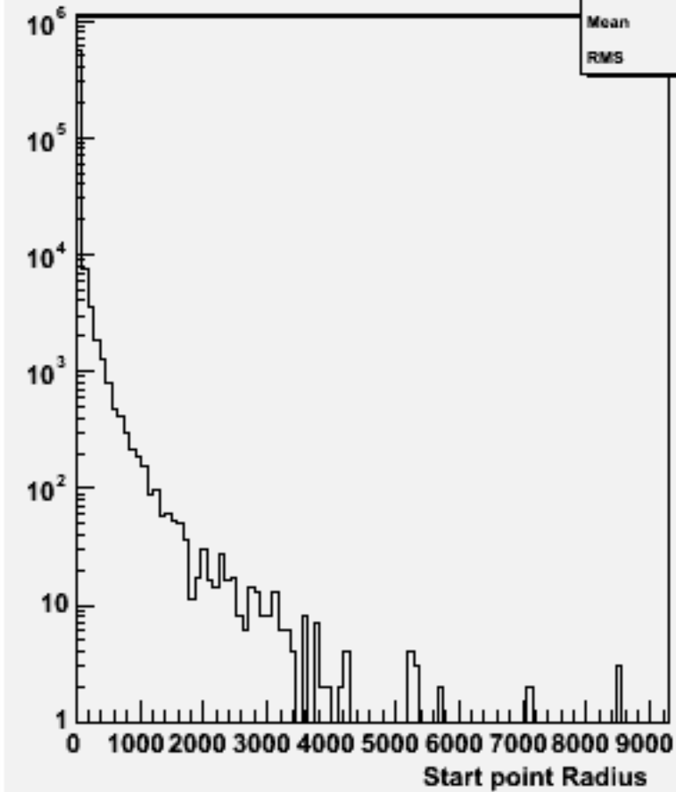
Start point R : w103264 e1a_e1uucc_o
