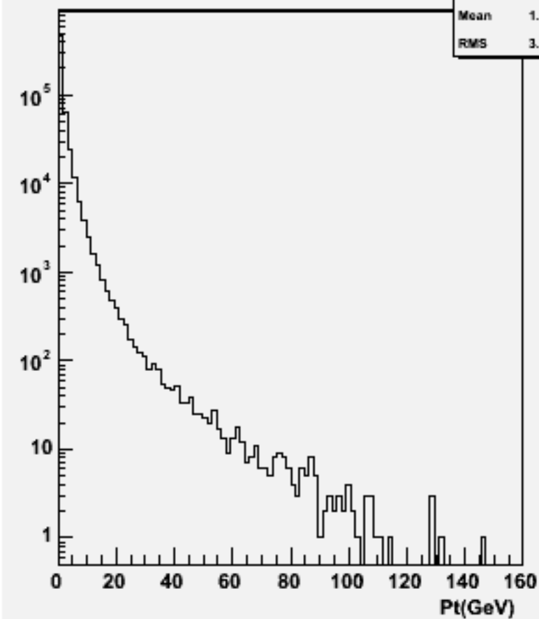
Particle Pt : w103264 e1a_e1uucc_o
