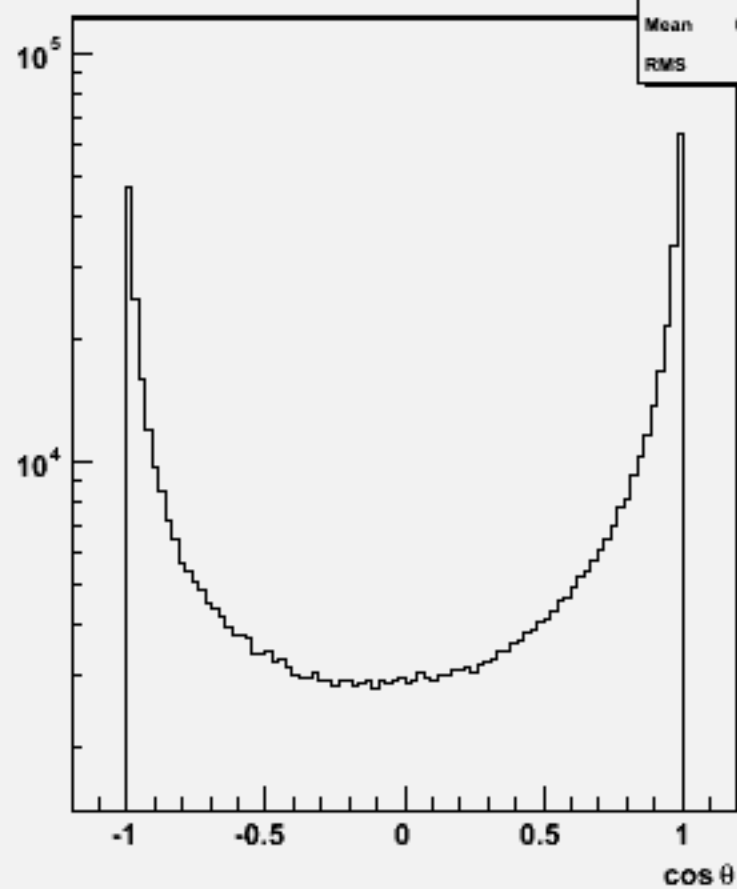
Particle cosθ : w103264 e1a_e1uucc_o
