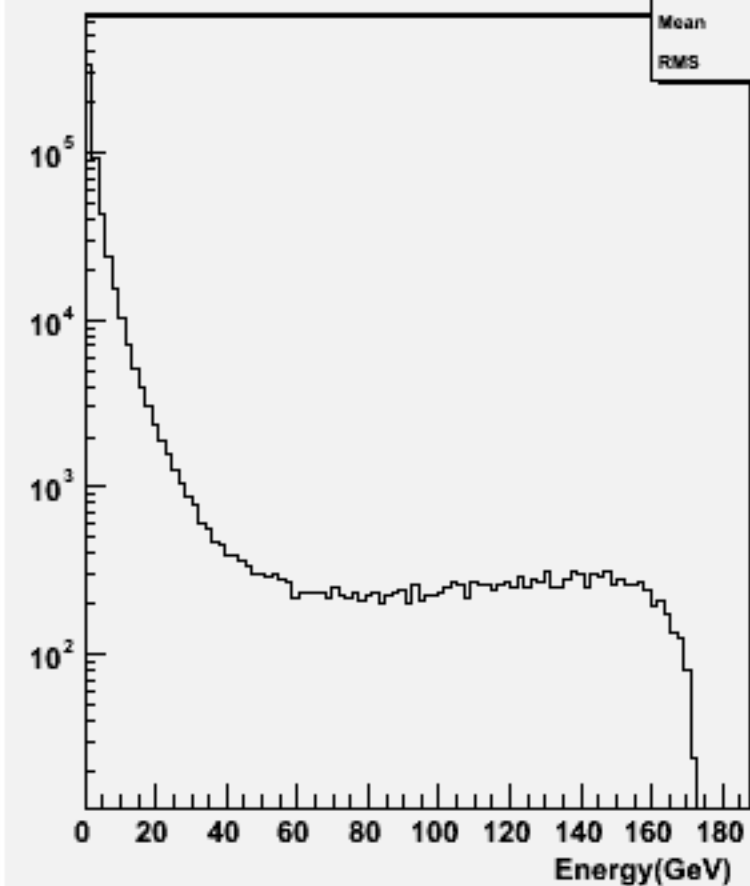
Particle Energy : w103264 e1a_e1uucc_o
