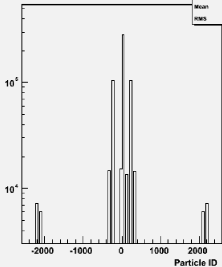
Particle ID : w103264 e1a_e1uucc_o
