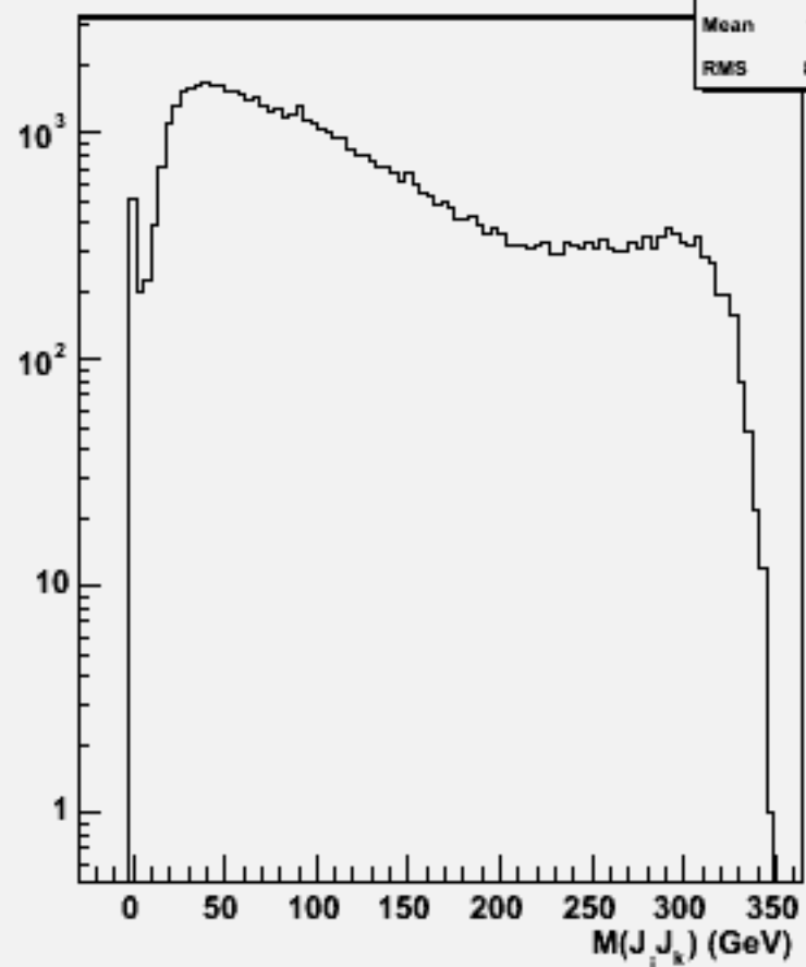
2jets mass(All comb)w103264 e1a_e1uucc_o
