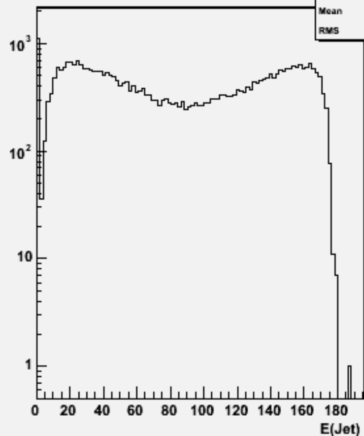
Jet energies(All jets)w103264 e1a_e1uucc_o
