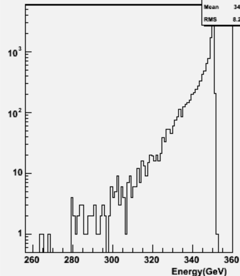
Thrust w103262 e1a_e1uucc_o
