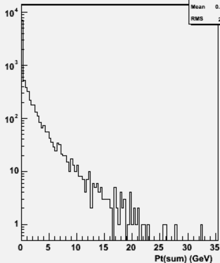
Pt Sum: w103262 e1a_e1uucc_o
