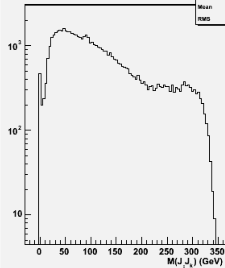
2jets mass(All comb)w103262 e1a_e1uucc_o
