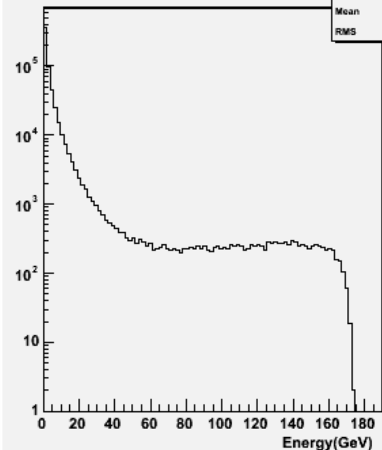
Particle Energy : w103262 e1a_e1uucc_o
