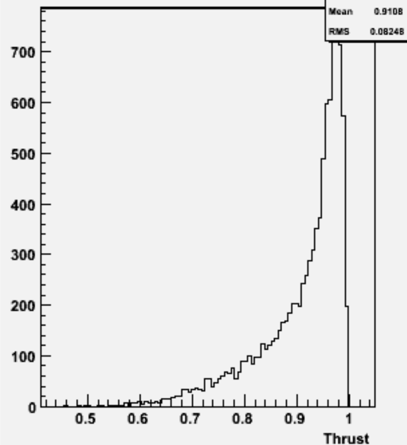
Thrust w103262 e1a_e1uucc_o
