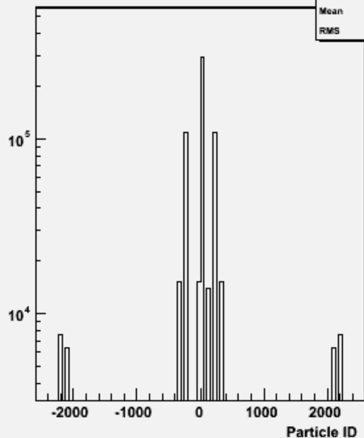
Particle ID : w103262 e1a_e1uucc_o
