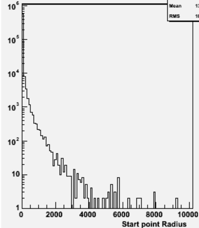
Start point R : w103262 e1a_e1uucc_o
