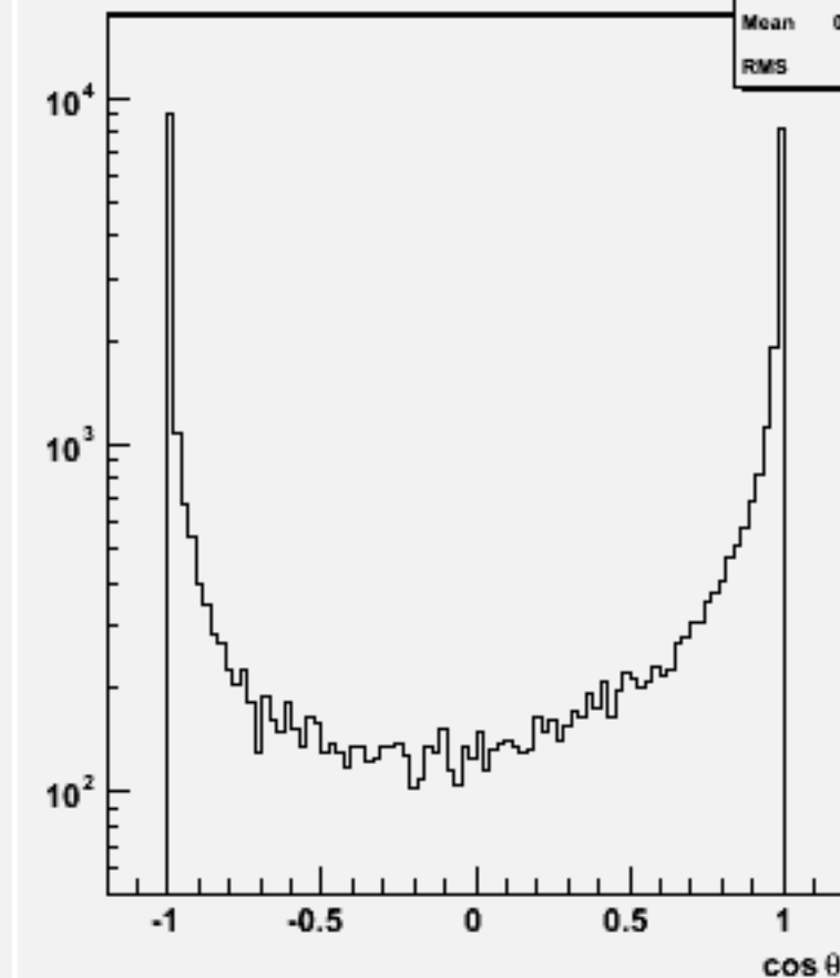
Jet cos \theta (All jets)w103262 e1a_e1uucc_o
