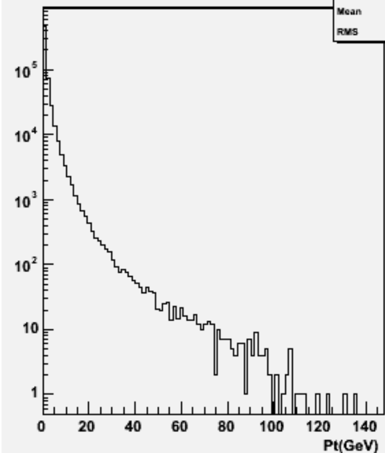
Particle Pt : w103262 e1a_e1uucc_o
