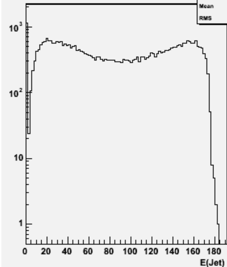
Jet energies(All jets)w103262 e1a_e1uucc_o
