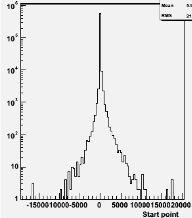
Start point Z : w103262 e1a_e1uucc_o
