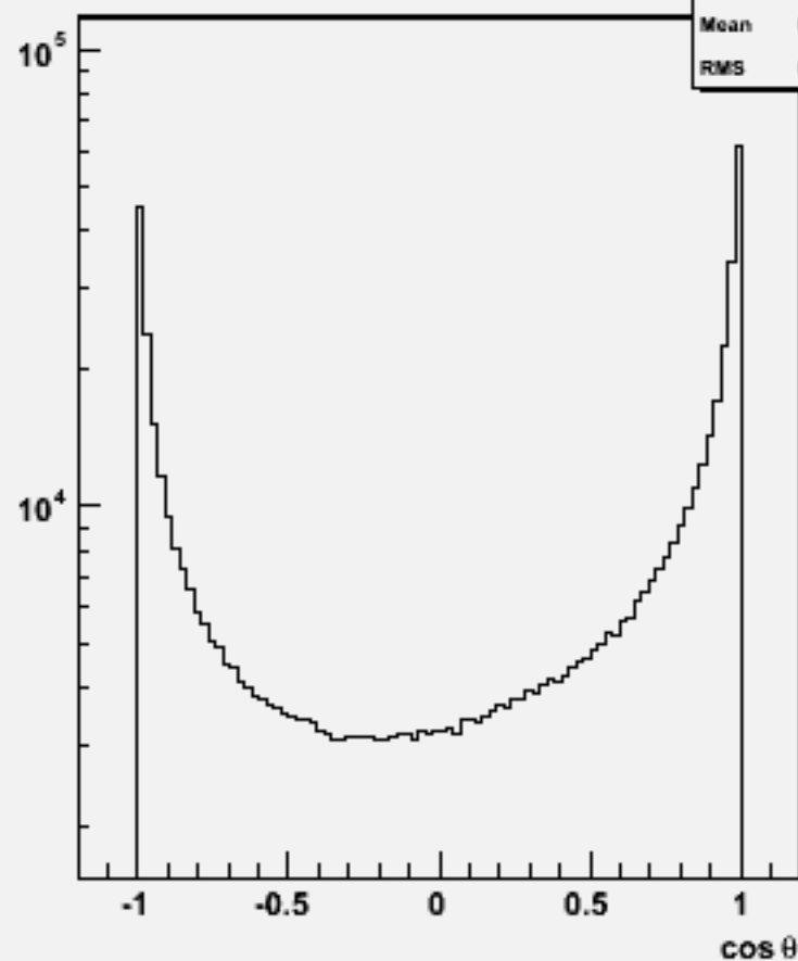
Particle cosθ : w103262 e1a_e1uucc_o
