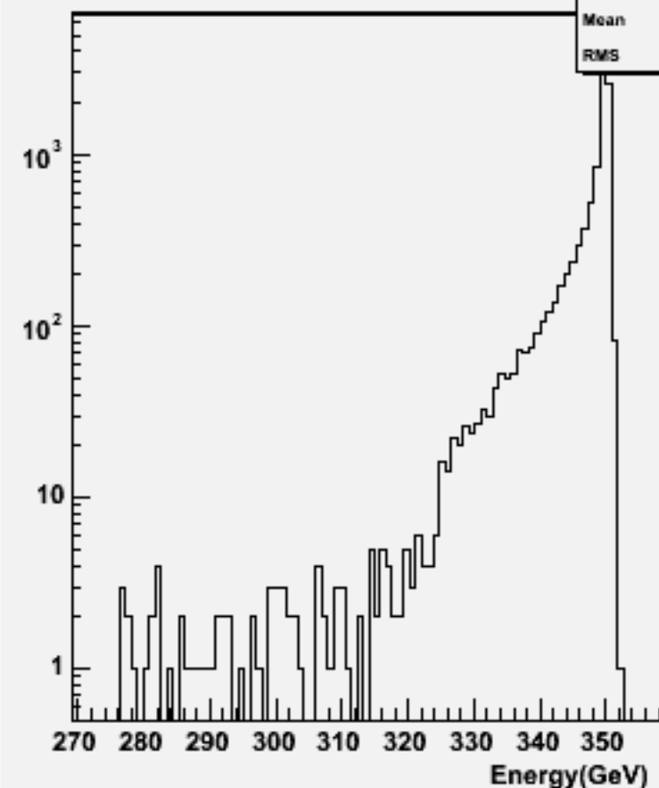
Thrust w103260 e1a_e1uuuu_o
