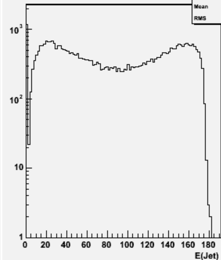
Jet energies(All jets)w103260 e1a_e1uuuu_o
