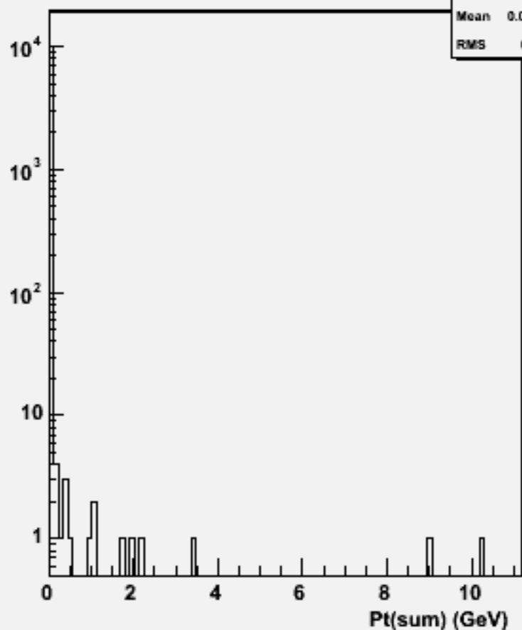
Pt Sum: w103260 e1a_e1uuuu_o
