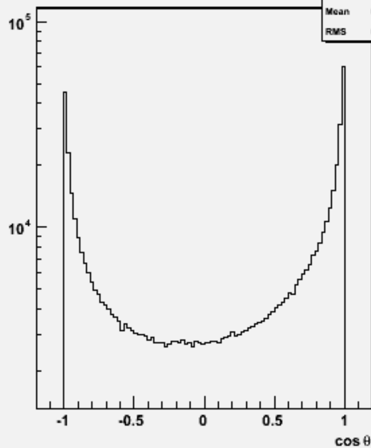
Particle cosθ : w103260 e1a_e1uuuu_o
