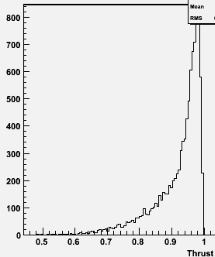
Thrust w103260 e1a_e1uuuu_o
