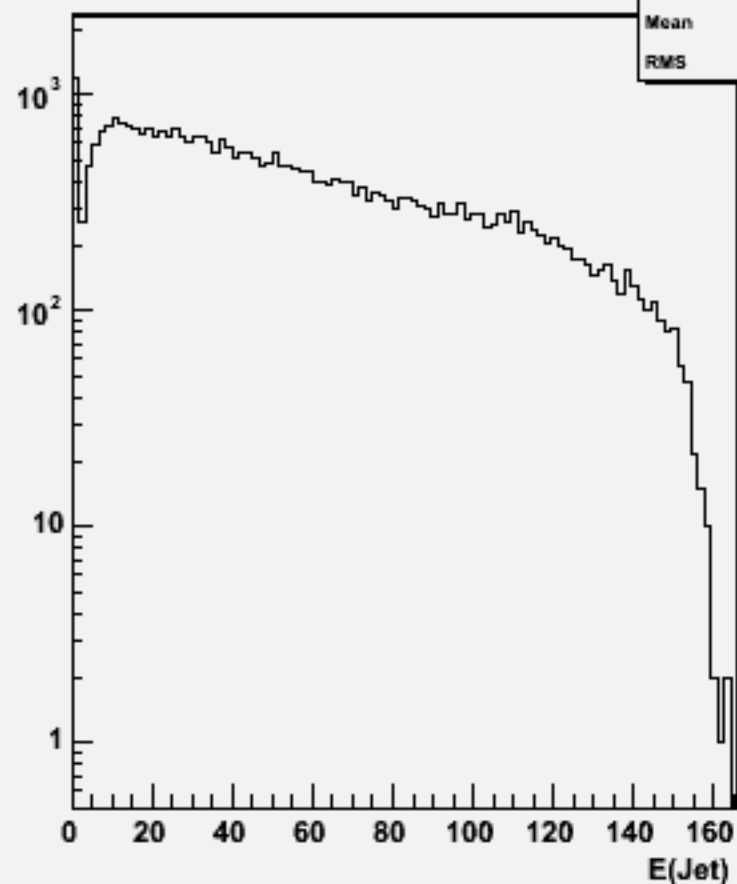
Jet energies(All jets)w103254 e1a_e1n3n3cc_o
