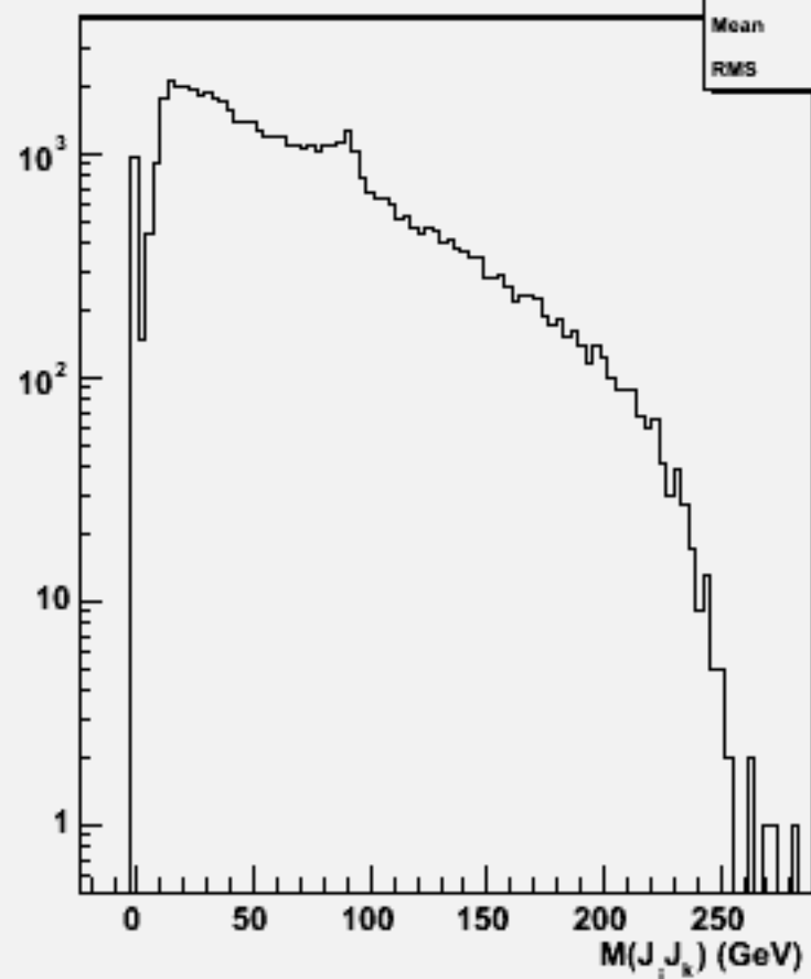
2jets mass(All comb)w103254 e1a_e1n3n3cc_o
