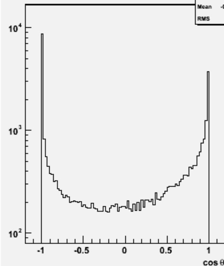
Jet cos \theta (All jets)w103254 e1a_e1n3n3cc_o
