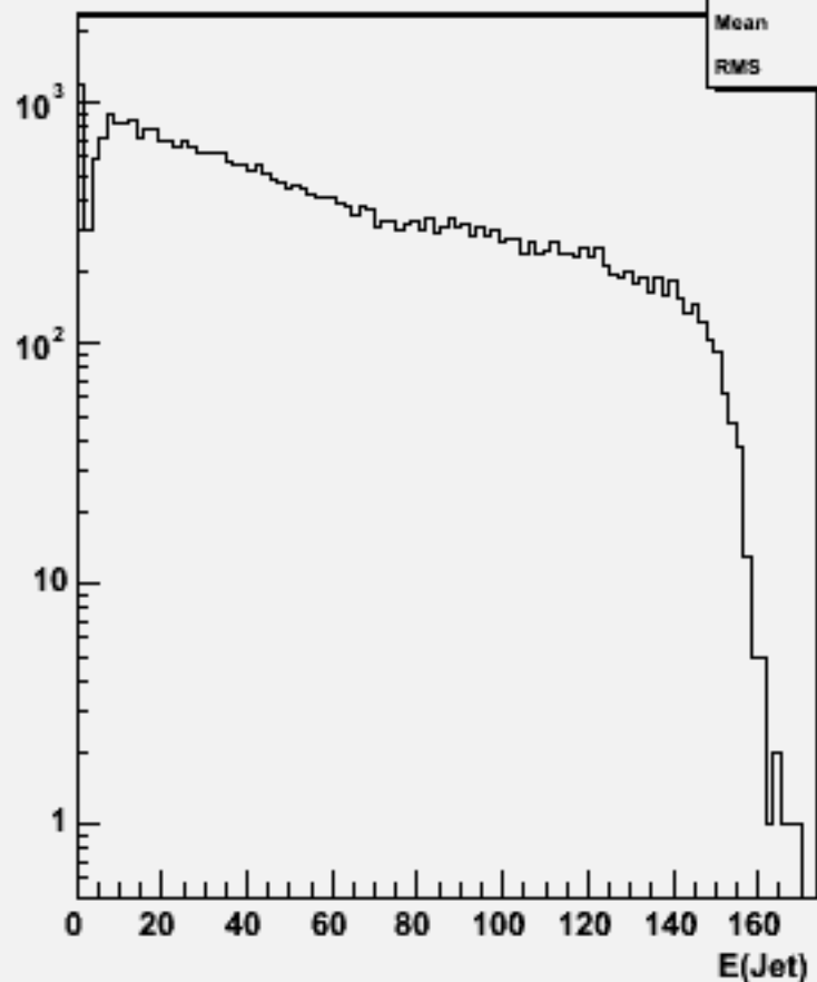
Jet energies(All jets)w103244 e1a_e1n2n2cc_o
