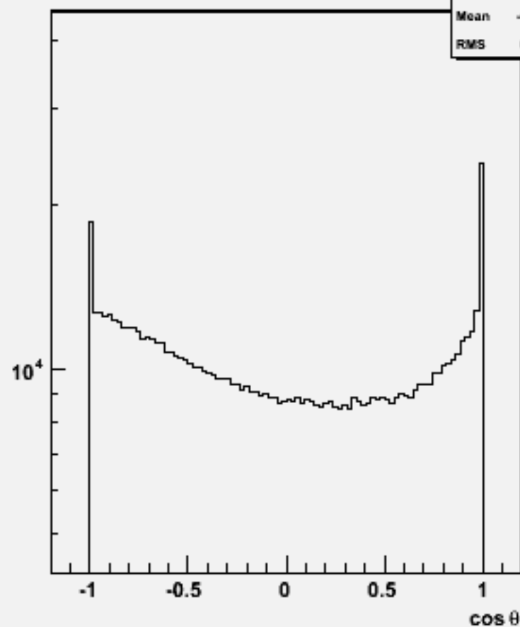
Particle cosθ : w103226 e1a_e1cssc_o
