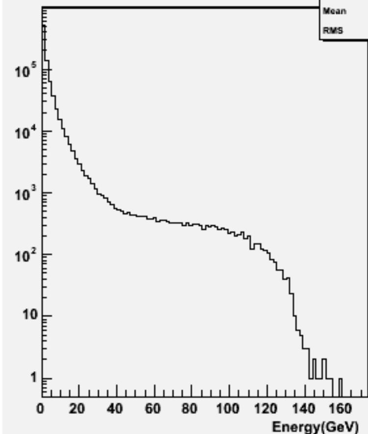
Start point R : w103226 e1a_e1cssc_o
