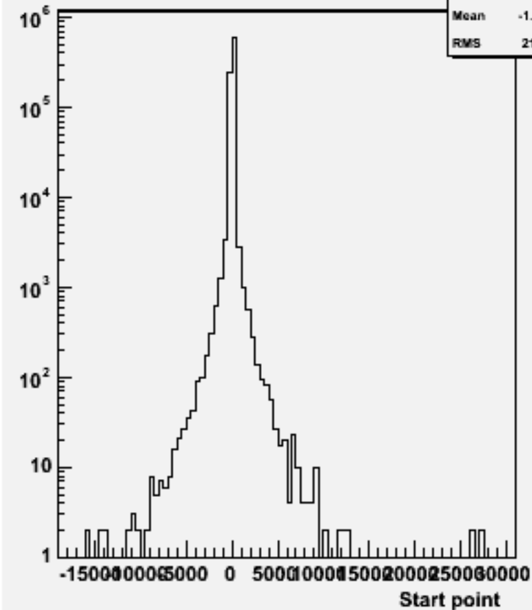
Start point Z : w103226 e1a_e1cssc_o
