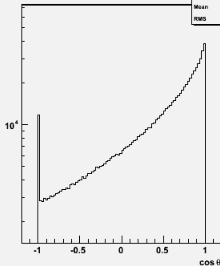
Particle \cos\theta : w103225 e1a_e1csdu_o
