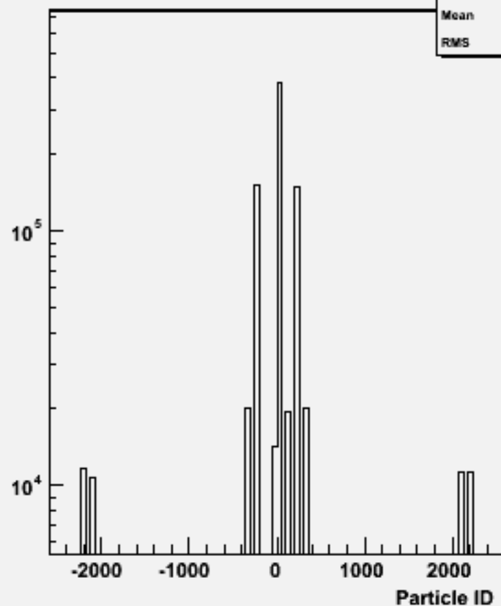
Particle ID : w103225 e1a_e1csdu_o
