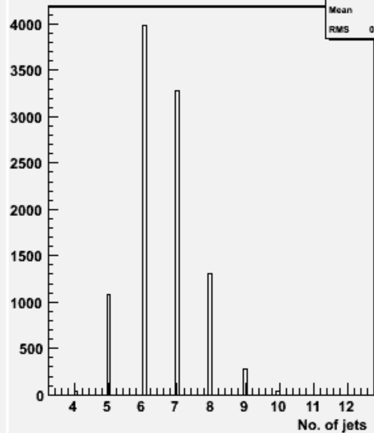
No. jets (ycut=0.001) : w103225 e1a_e1csdu_o
