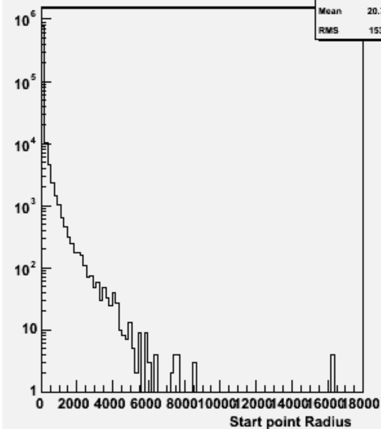
Start point R : w103225 e1a_e1csdu_o
