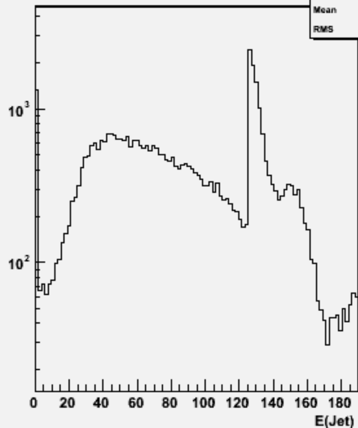
Jet energies(All jets)w103225 e1a_e1csdu_o
