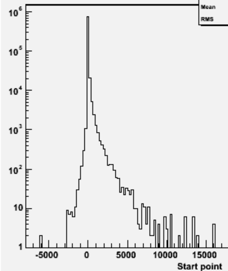
Start point Z : w103225 e1a_e1csdu_o
