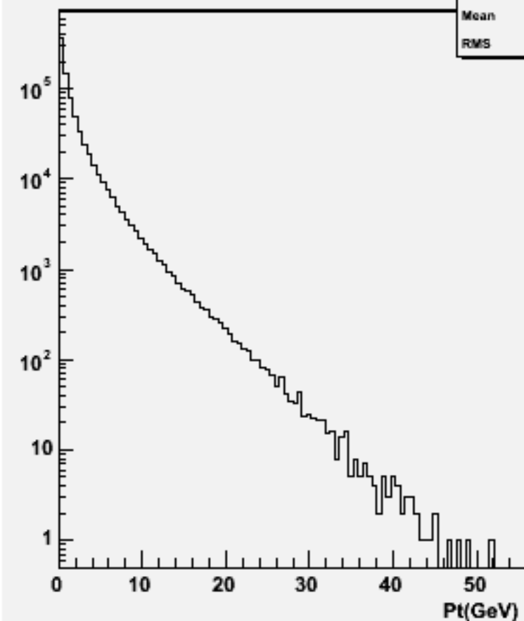
Particle Pt : w103225 e1a_e1csdu_o
