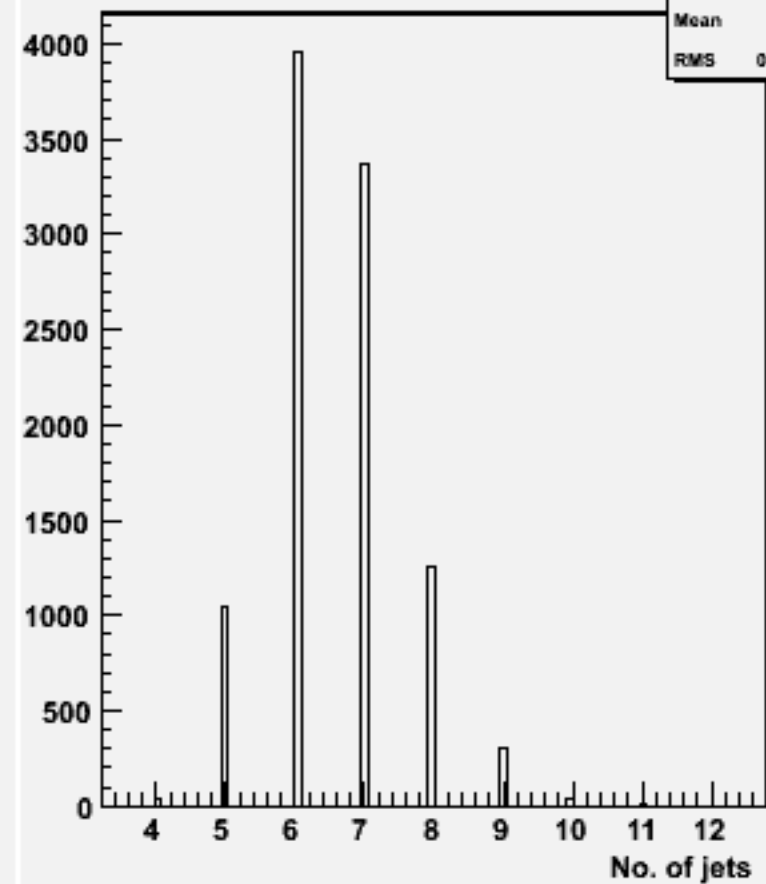
No. jets (ycut=0.001) : w103223 e1a_e1csdu_o
