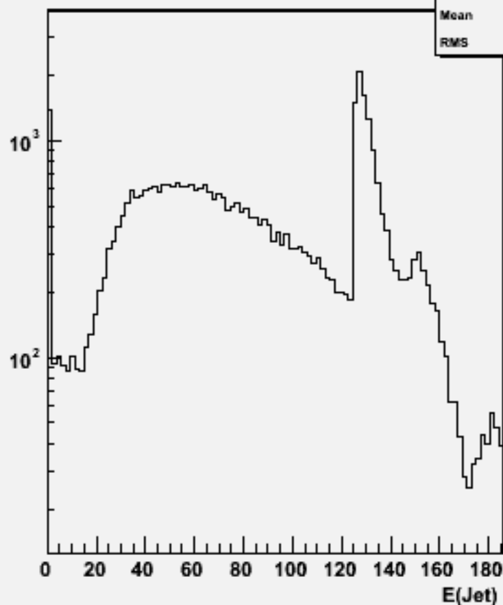
Jet energies(All jets)w103223 e1a_e1csdu_o
