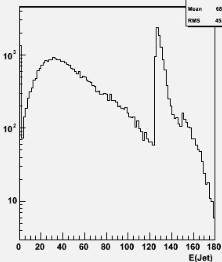
Jet energies(All jets)w103221 e1a_e1cse3n3_o
