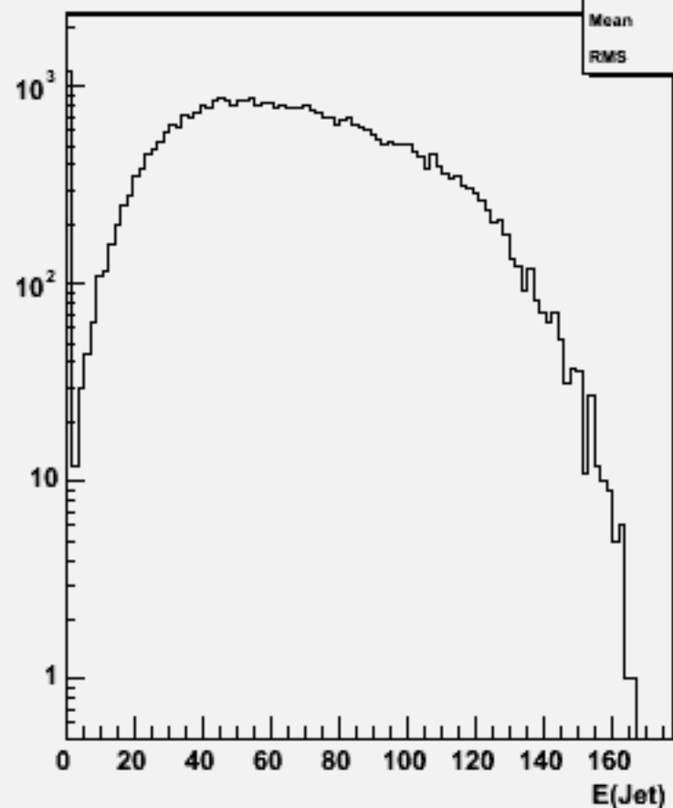
Jet energies(All jets)w103218 e1a_e1cse3n3_o
