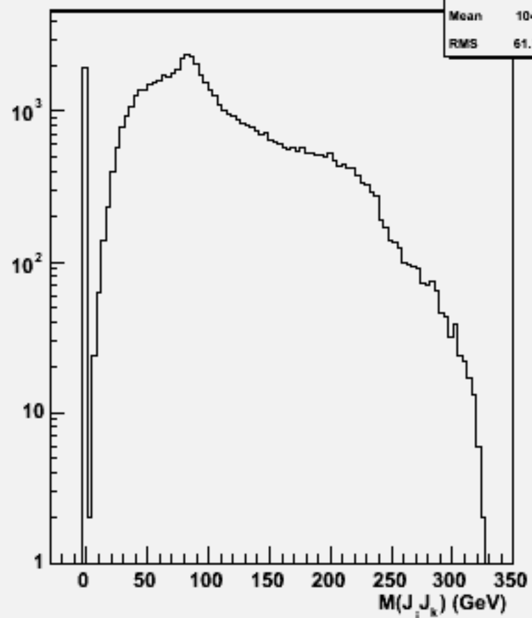
2jets mass(All comb)w103217 e1a_e1cse2n2_o
