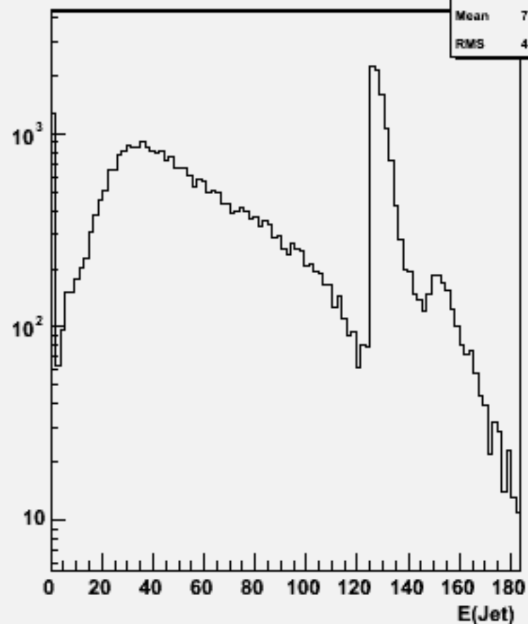
Jet energies(All jets)w103217 e1a_e1cse2n2_o
