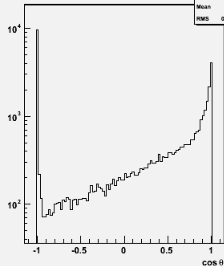
Jet cos \theta (All jets)w103217 e1a_e1cse2n2_o
