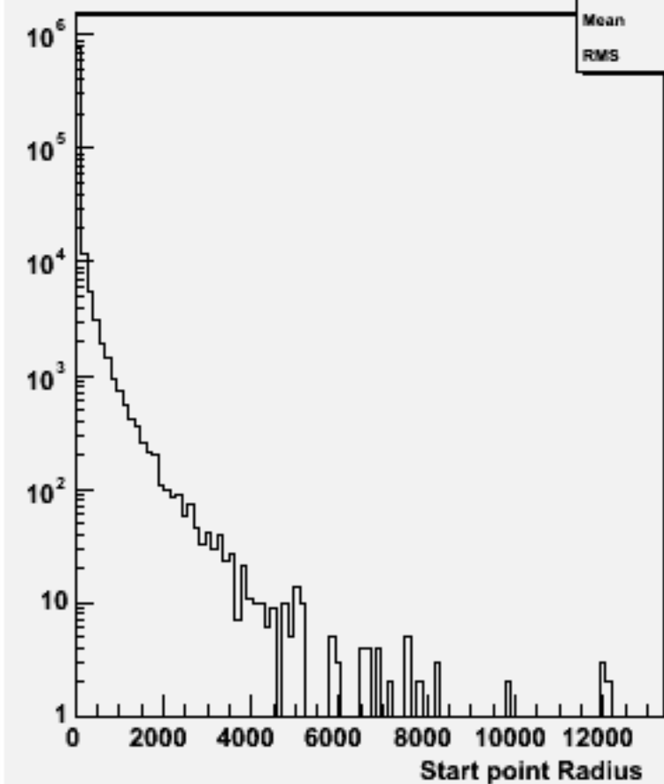
Start point R : w103209 e1a_e1udsc_o
