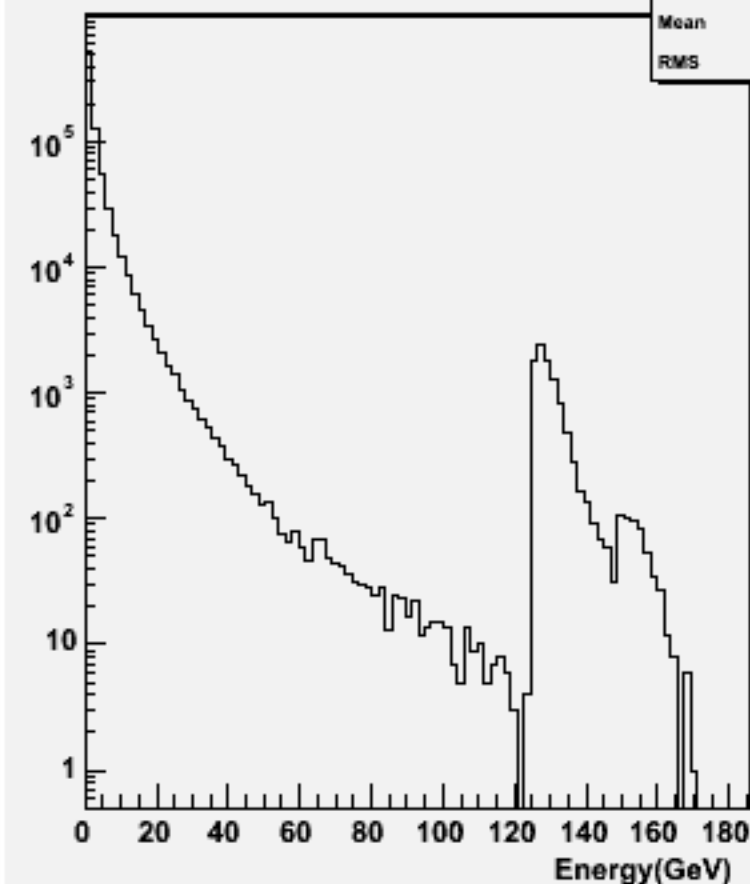
Particle Energy : w103209 e1a_e1udsc_o
