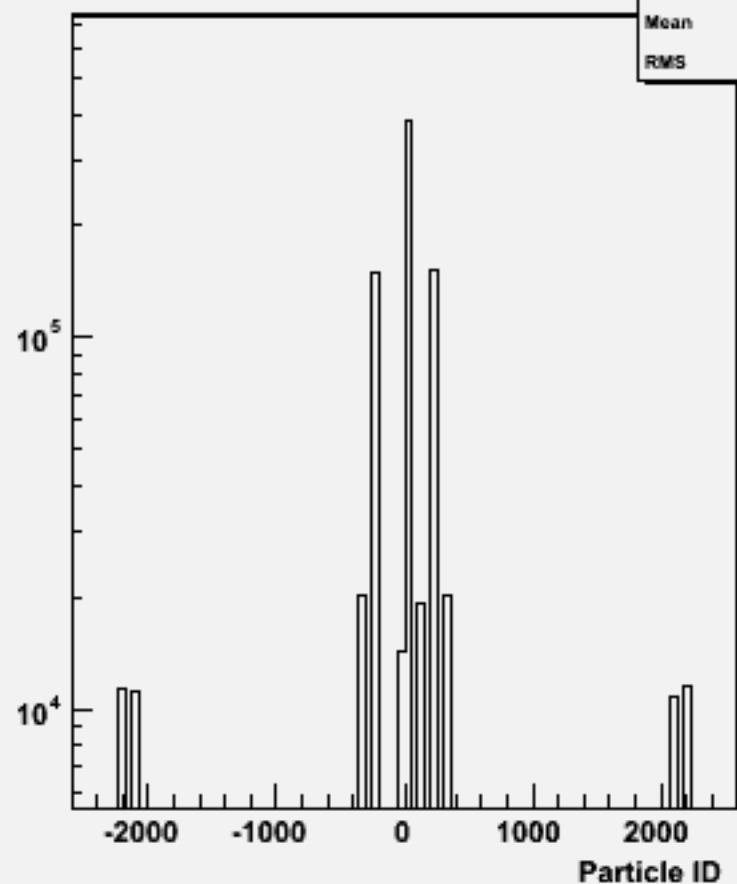
Particle ID : w103209 e1a_e1udsc_o
