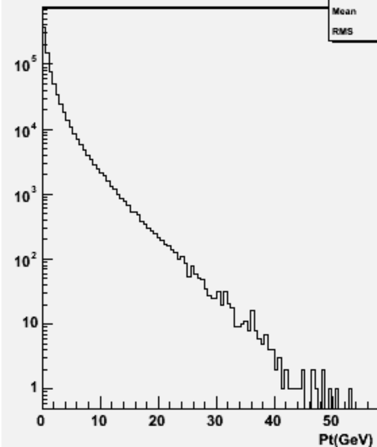
Particle Pt : w103209 e1a_e1udsc_o
