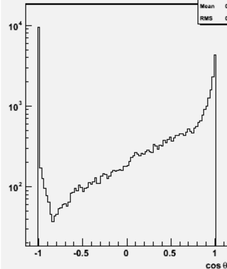
Jet cos \theta (All jets)w103209 e1a_e1udsc_o
