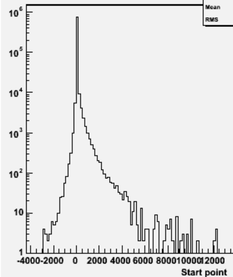
Start point Z : w103209 e1a_e1udsc_o
