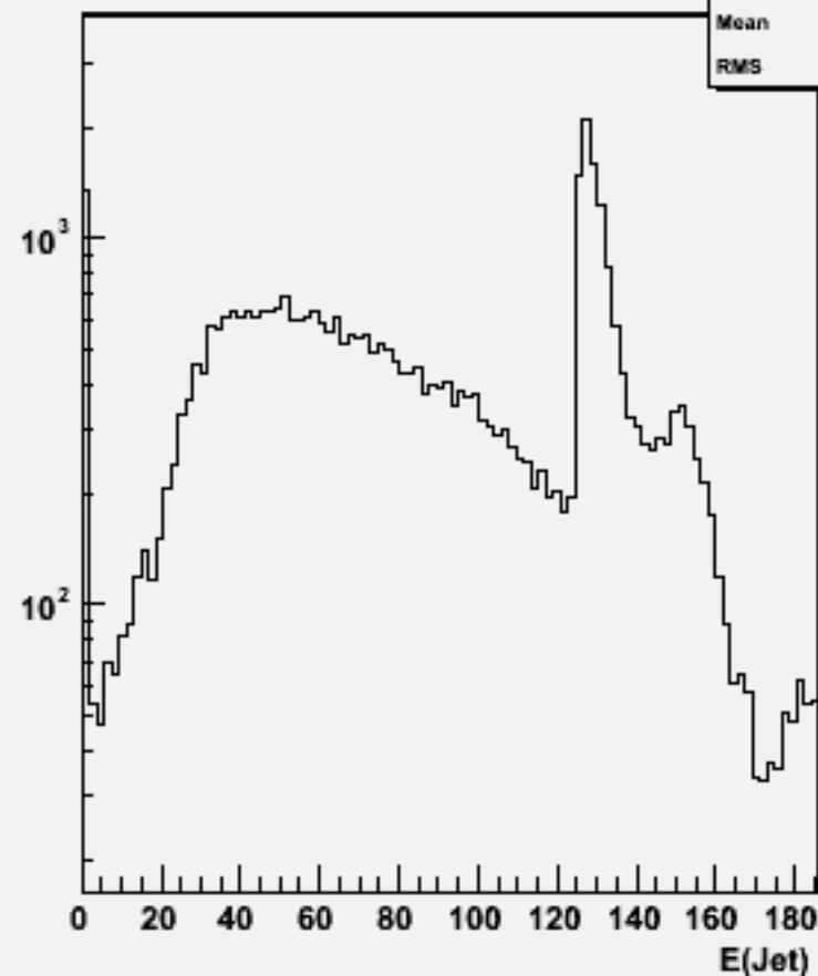
Jet energies(All jets)w103209 e1a_e1udsc_o
