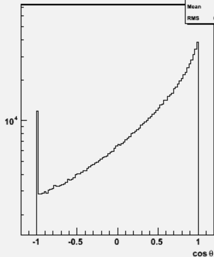
Particle \cos\theta : w103209 e1a_e1udsc_o
