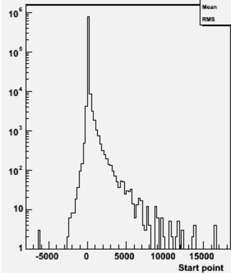
Start point Z : w103207 e1a_e1udsc_o
