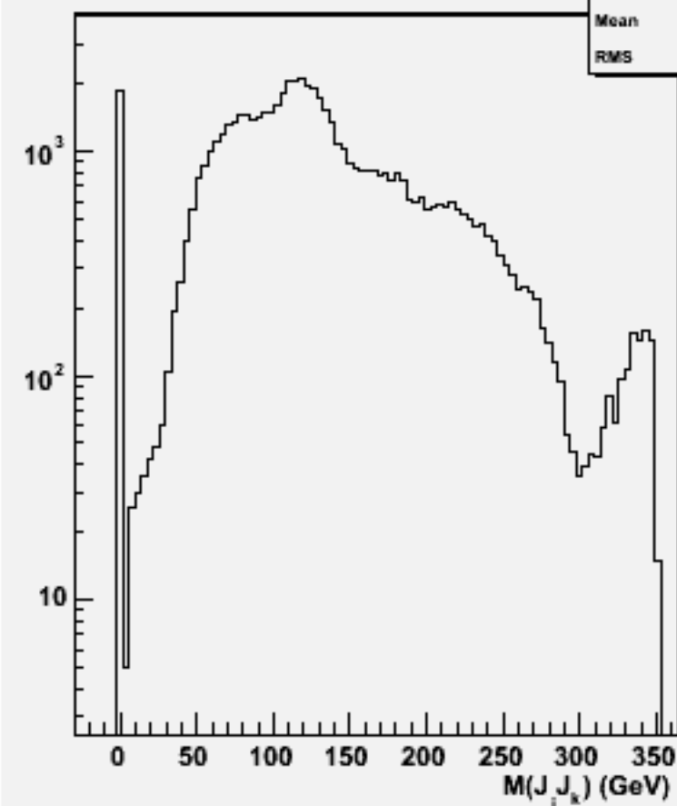
2jets mass(All comb)w103207 e1a_e1udsc_o
