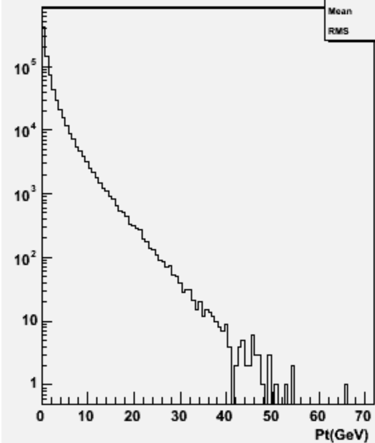
Particle Pt : w103207 e1a_e1udsc_o
