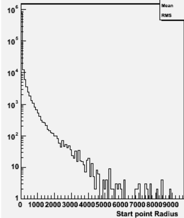
Start point R : w103207 e1a_e1udsc_o
