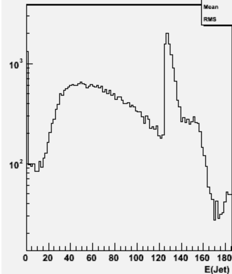
Jet energies(All jets)w103207 e1a_e1udsc_o
