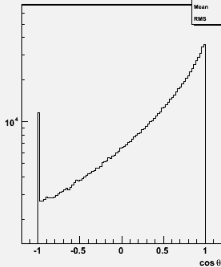
Particle cosθ : w103207 e1a_e1udsc_o
