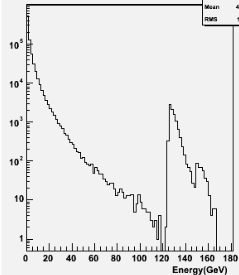
Particle Energy : w103207 e1a_e1udsc_o
