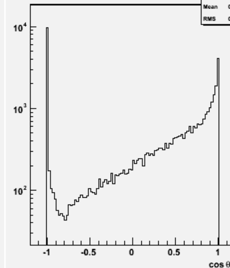
Jet cos \theta (All jets)w103207 e1a_e1udsc_o
