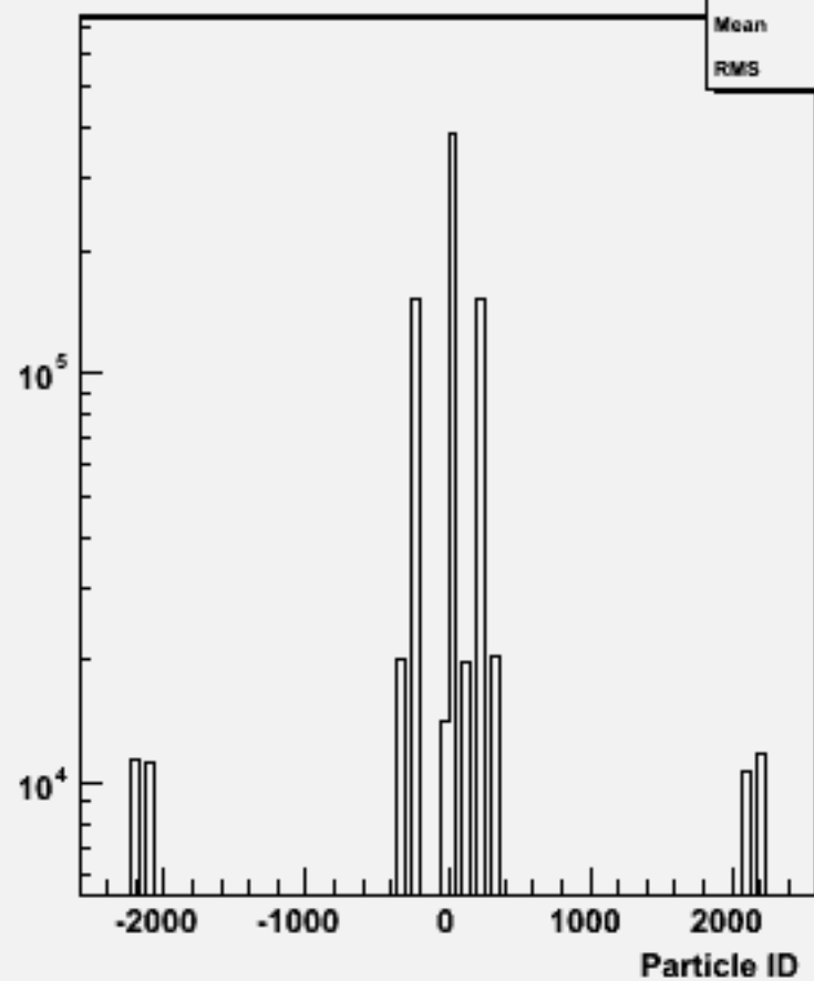
Particle ID : w103207 e1a_e1udsc_o
