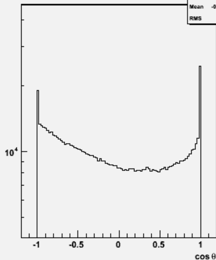
Particle cos \theta : w103204 e1a_e1uddu_o
