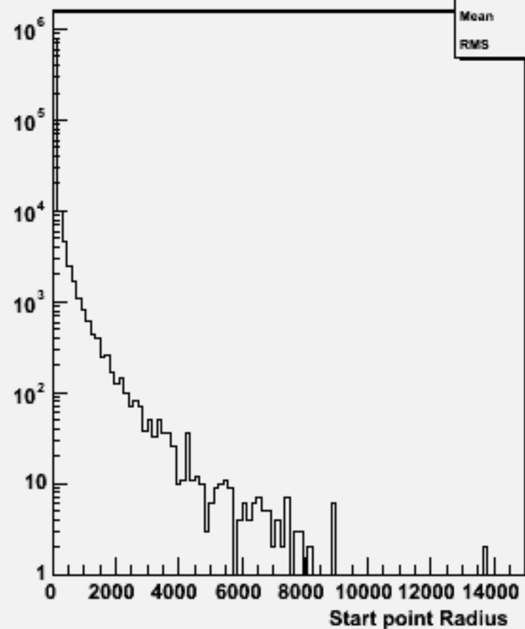
Start point R : w103204 e1a_e1uddu_o
