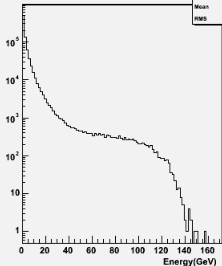
Start point R : w103204 e1a_e1uddu_o
