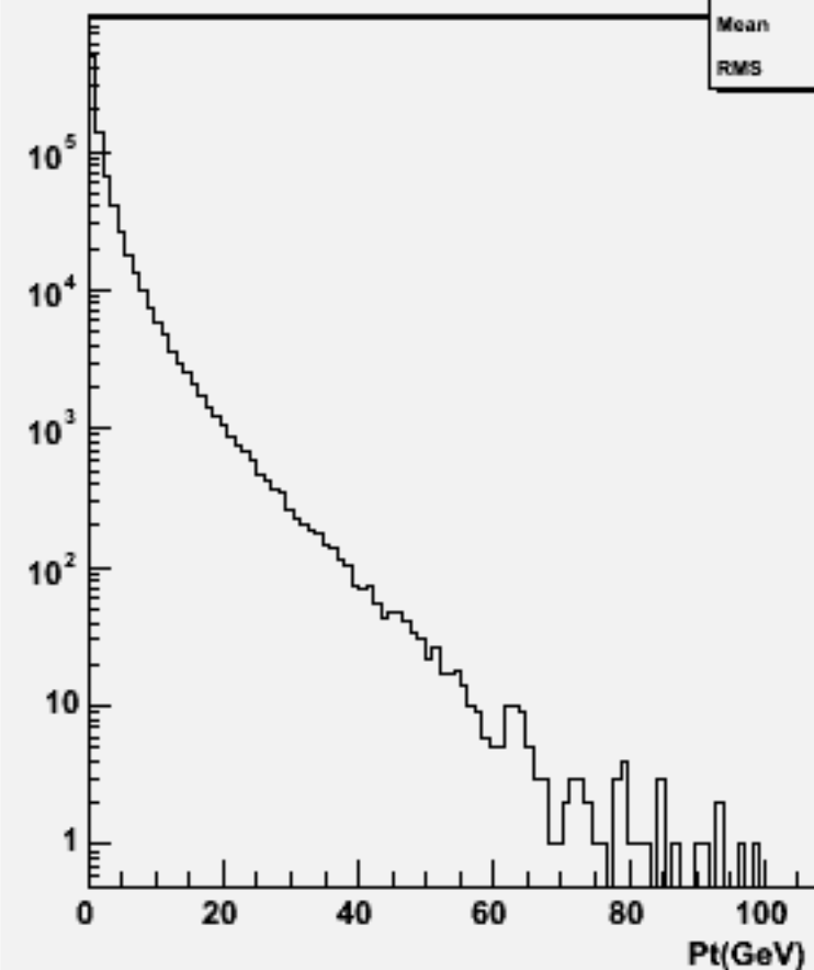
Start point Z : w103204 e1a_e1uddu_o
