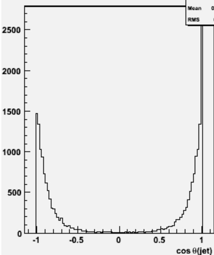
cos \theta for 2-jets :w103204 e1a_e1uddu_o
