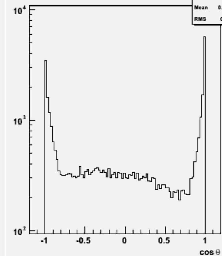
Jet cos \theta (All jets)w103204 e1a_e1uddu_o
