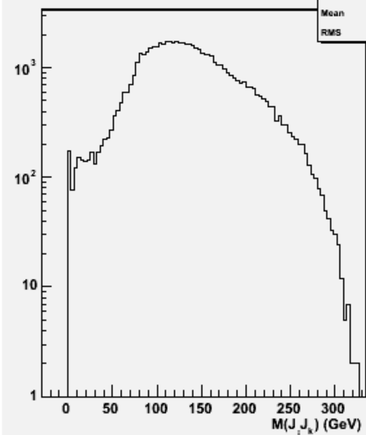
2jets mass(All comb)w103204 e1a_e1uddu_o
