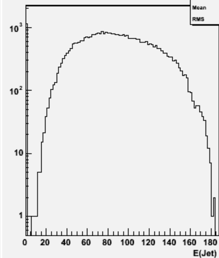
Jet energies(All jets)w103204 e1a_e1uddu_o
