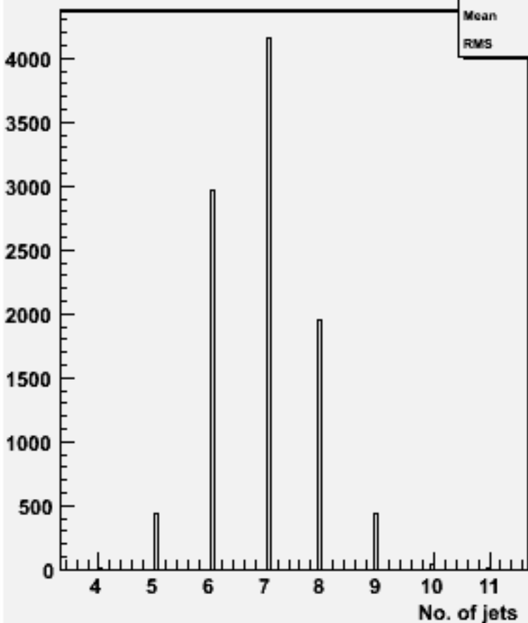
No. jets (ycut=0.001) : w103204 e1a_e1uddu_o
