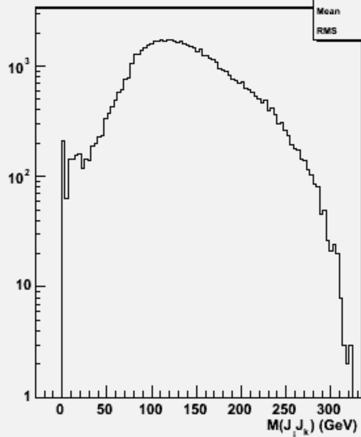
2jets mass(All comb)w103202 e1a_e1uddu_o
