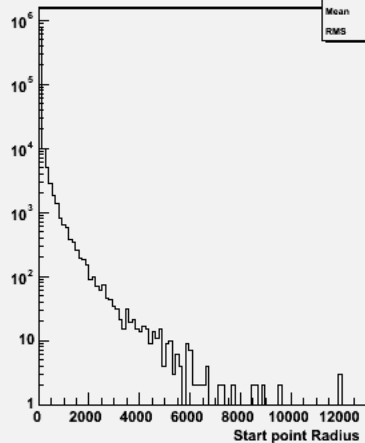
Start point R : w103202 e1a_e1uddu_o
