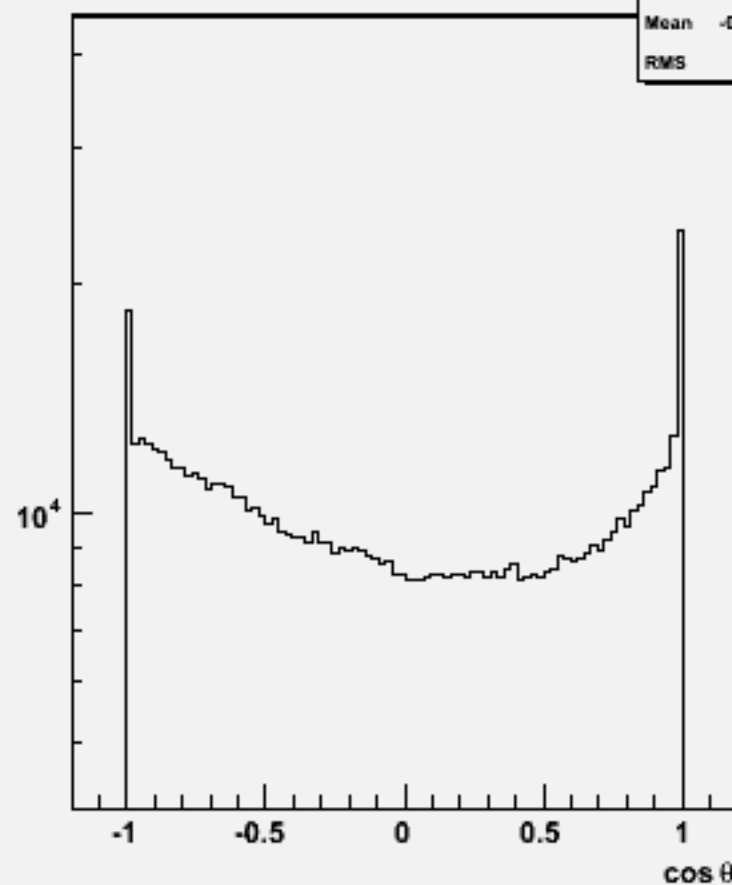
Particle cosθ : w103202 e1a_e1uddu_o
