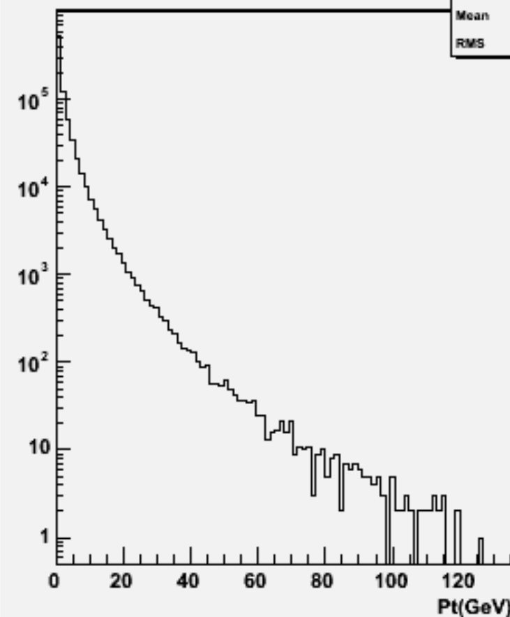
Start point Z : w103202 e1a_e1uddu_o
