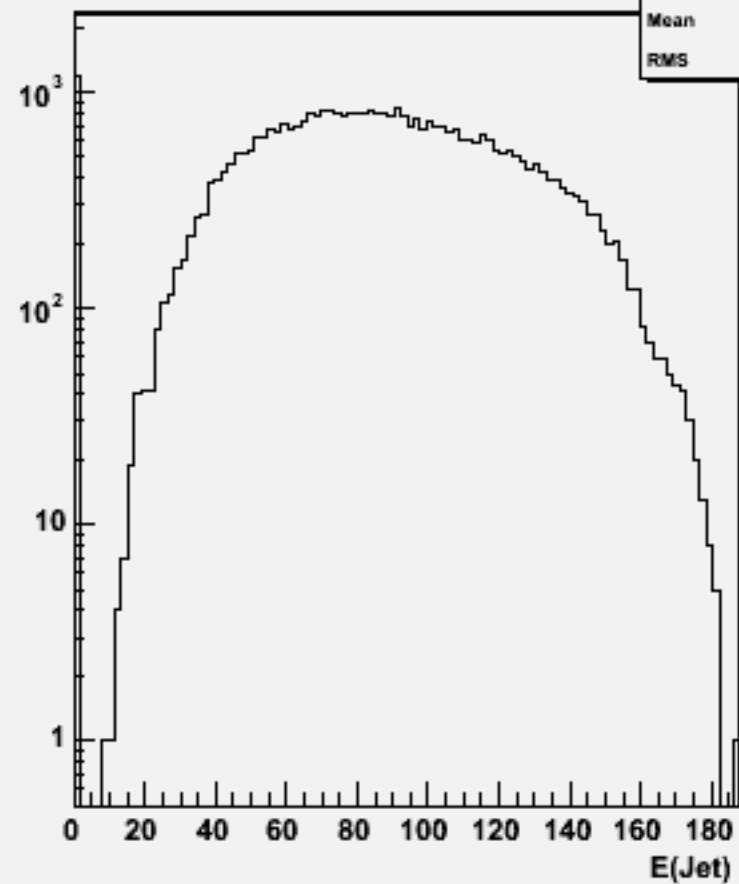
Jet energies(All jets)w103202 e1a_e1uddu_o
