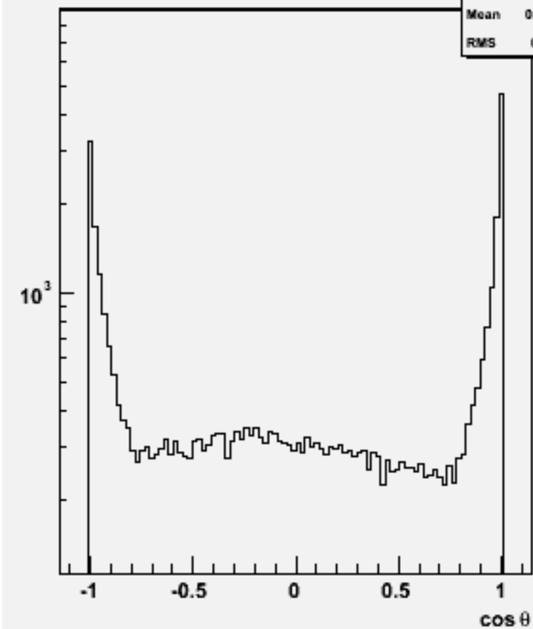
Jet cos \theta (All jets)w103202 e1a_e1uddu_o
