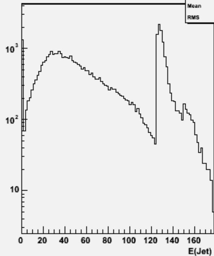
Jet energies(All jets)w103189 e1a_e1n3e3sc_o
