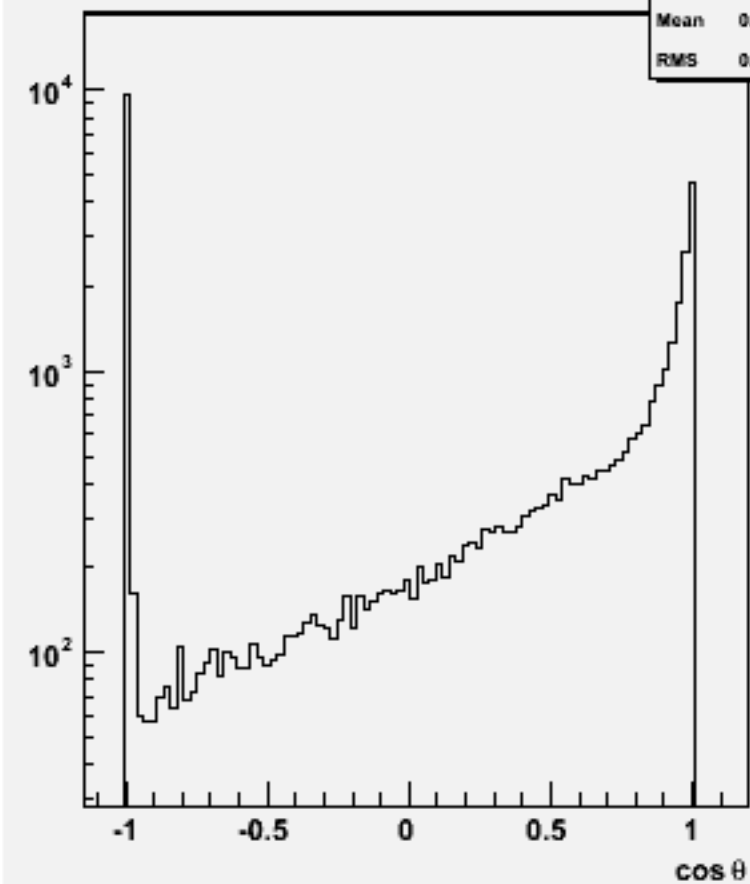
Jet cos \theta (All jets)w103189 e1a_e1n3e3sc_o
