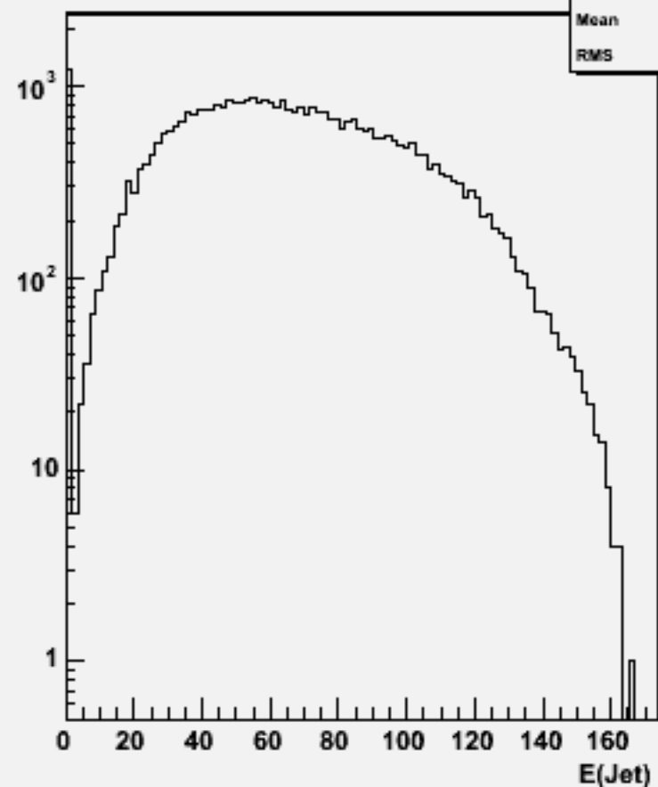
Jet energies(All jets)w103188 e1a_e1n3e3sc_o
