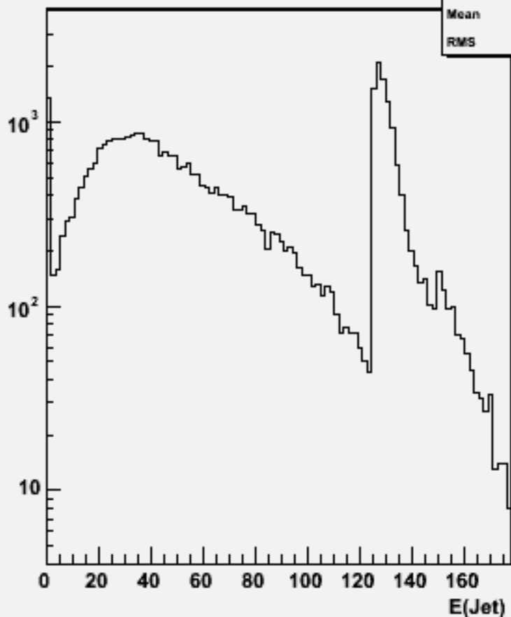
Jet energies(All jets)w103187 e1a_e1n3e3sc_o
