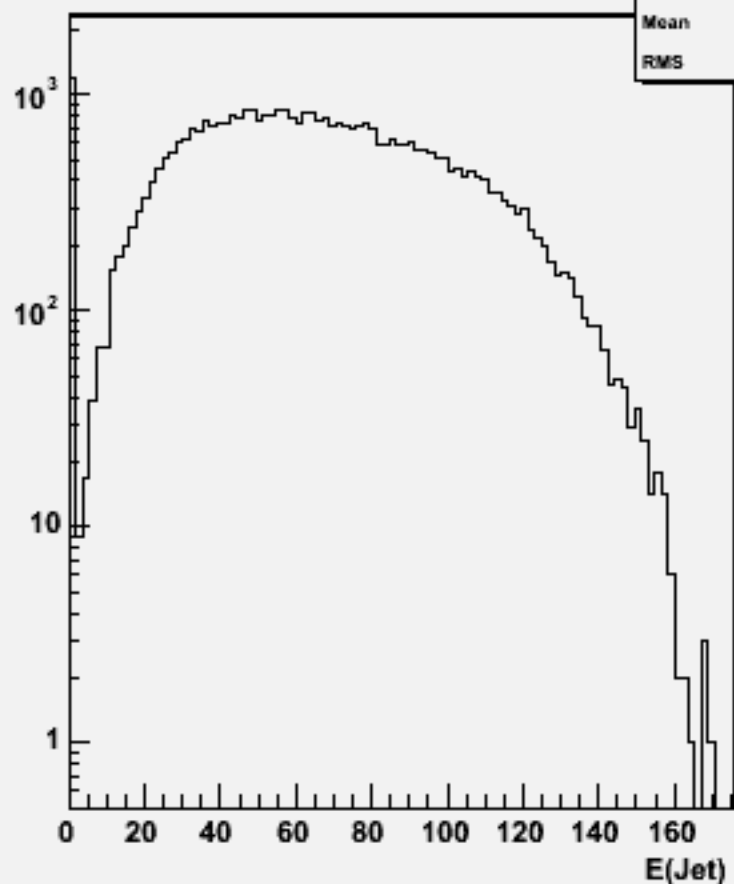
Jet energies(All jets)w103186 e1a_e1n3e3sc_o
