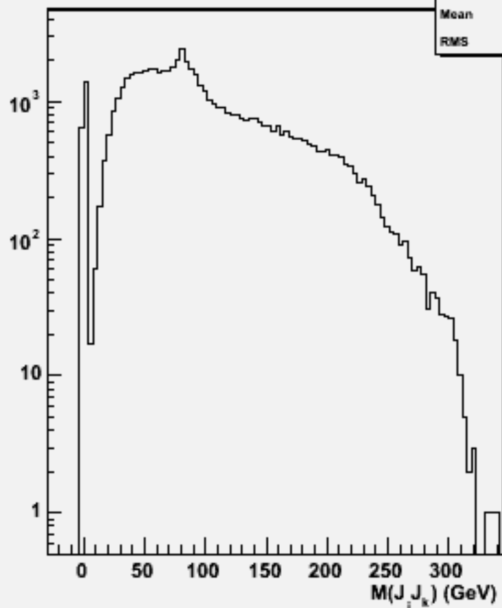
2jets mass(All comb)w103185 e1a_e1n3e3du_o
