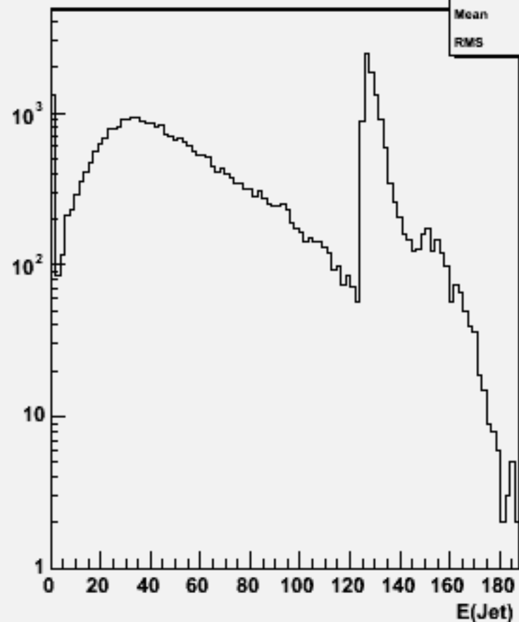
Jet energies(All jets)w103185 e1a_e1n3e3du_o
