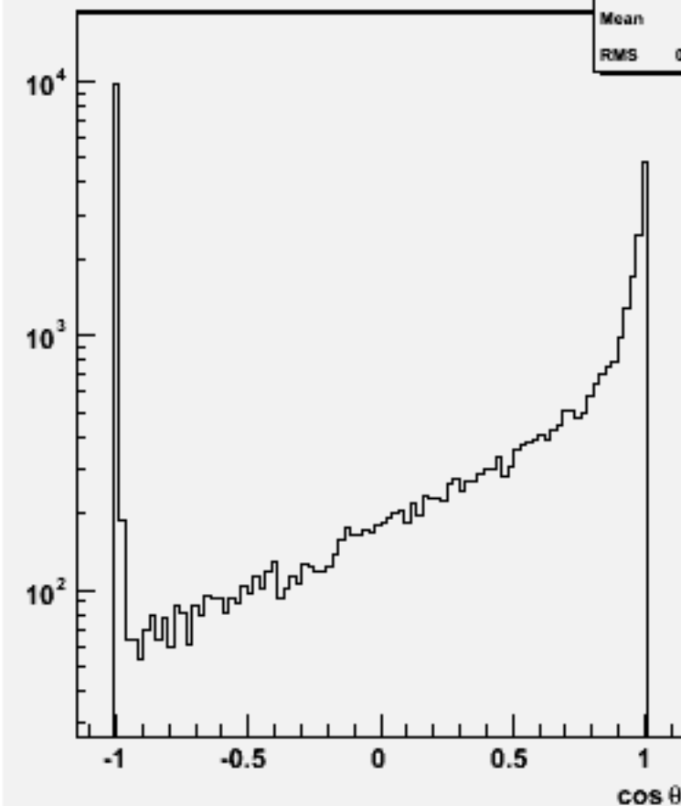
Jet cos \theta (All jets)w103185 e1a_e1n3e3du_o
