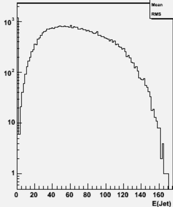
Jet energies(All jets)w103182 e1a_e1n3e3du_o
