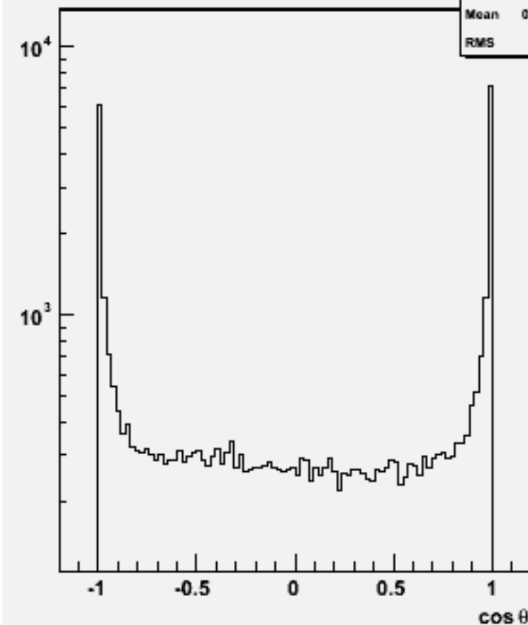
Jet cos \theta (All jets)w103182 e1a_e1n3e3du_o
