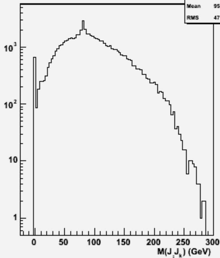
2jets mass(All comb)w103182 e1a_e1n3e3du_o
