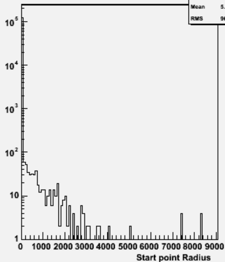
Start point R : w103180 e1a_e1n3e3e3n3_o
