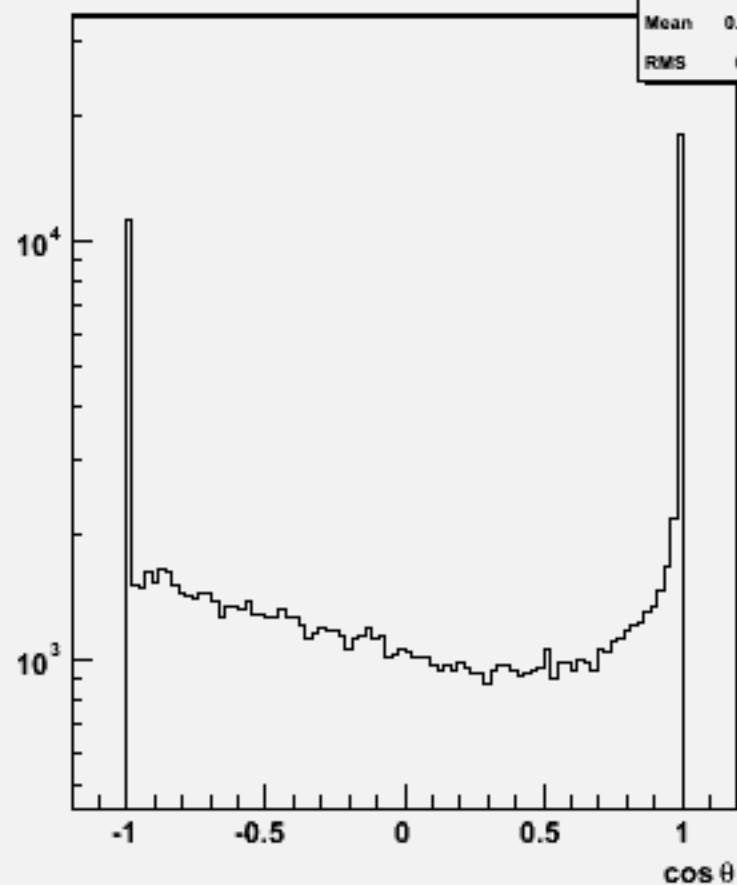
Particle cos \theta : w103180 e1a_e1n3e3e3n3_o
