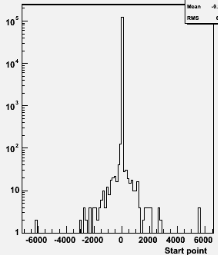
Start point Z : w103180 e1a_e1n3e3e3n3_o
