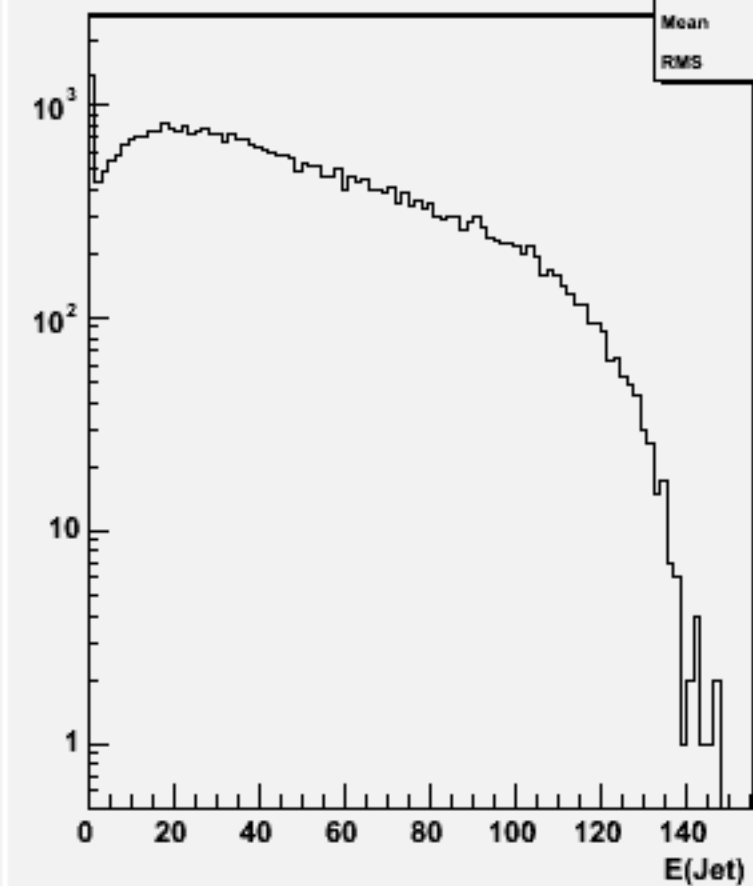
Jet energies(All jets)w103180 e1a_e1n3e3e3n3_o
