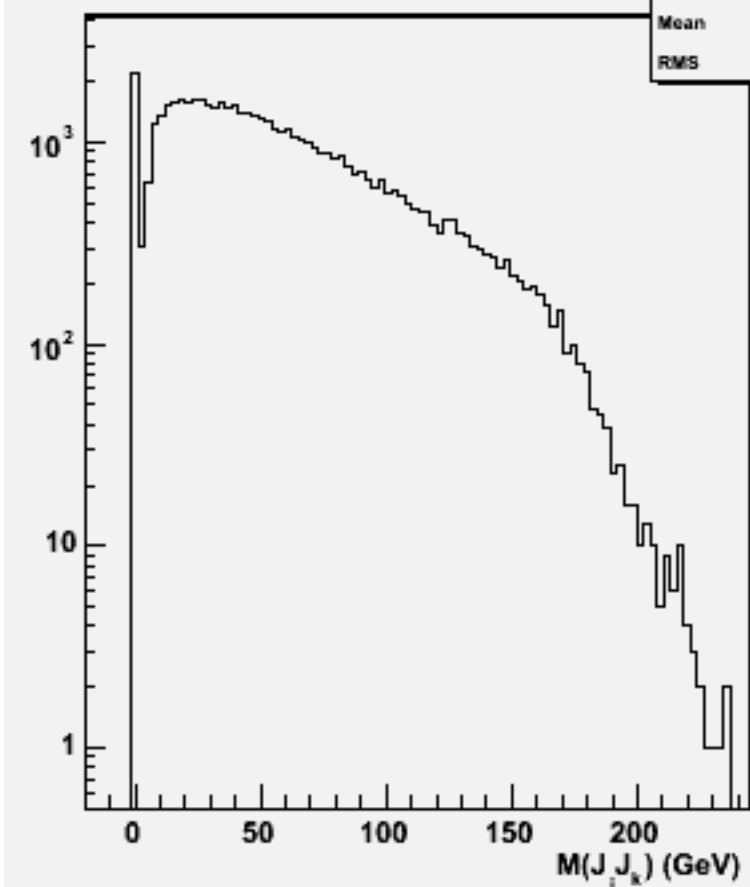
2jets mass(All comb)w103180 e1a_e1n3e3e3n3_o
