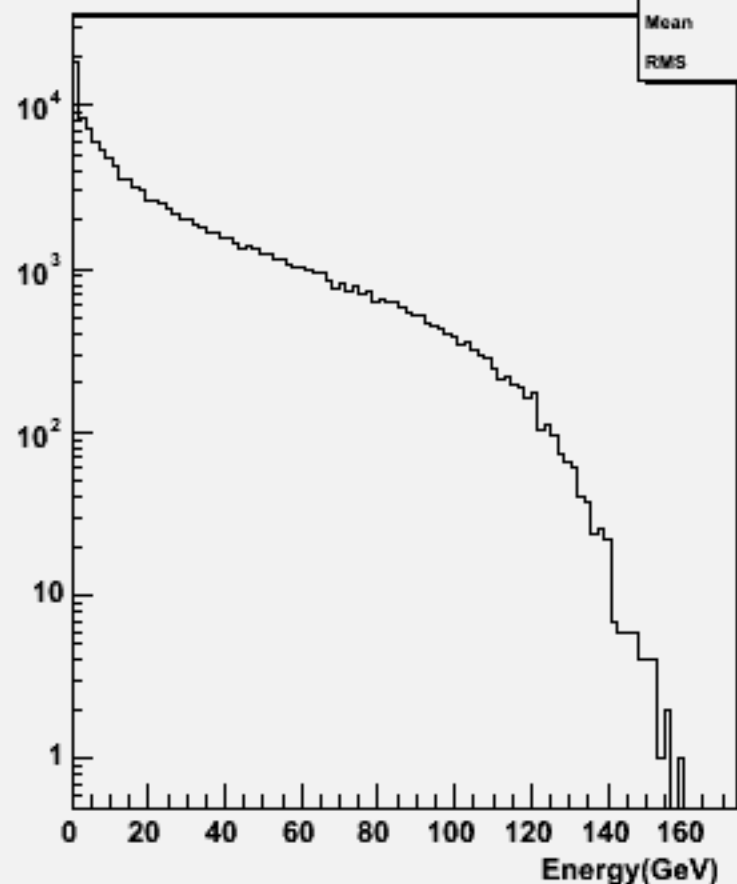
Start point R : w103180 e1a_e1n3e3e3n3_o
