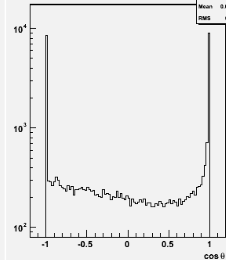
Jet cos \theta (All jets)w103180 e1a_e1n3e3e3n3_o
