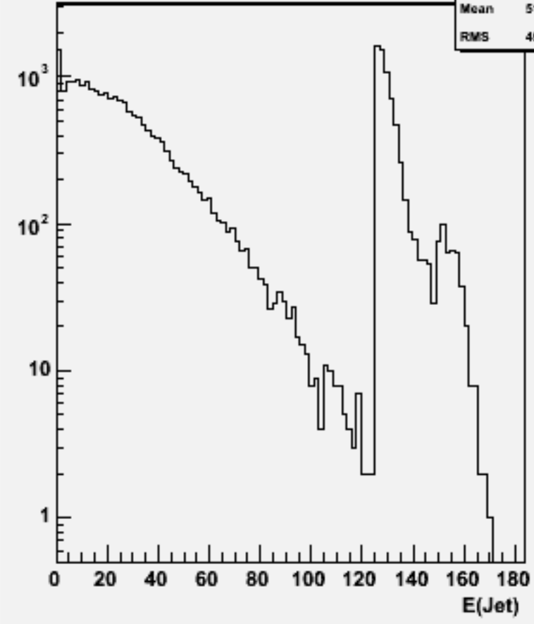
Jet energies(All jets)w103179 e1a_e1n3e3e3n3_o
