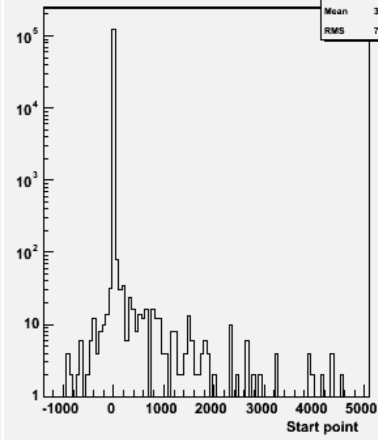
Start point Z : w103179 e1a_e1n3e3e3n3_o
