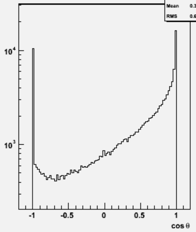
Particle cos θ : w103179 e1a_e1n3e3e3n3_o
