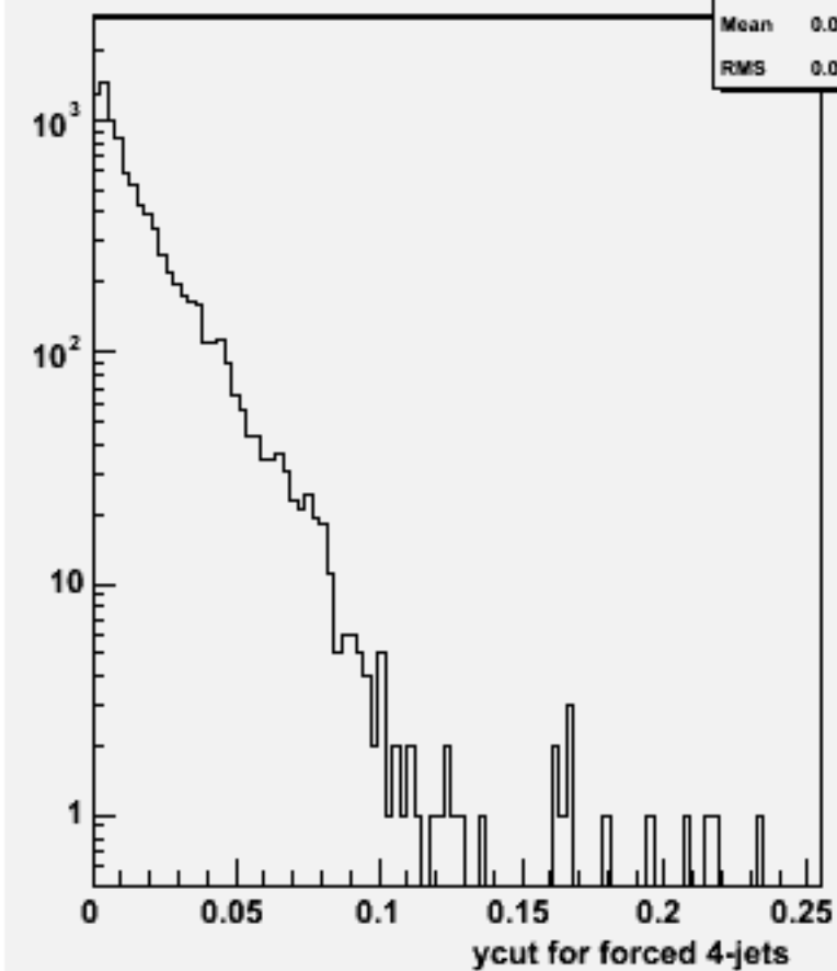
Ycut for 4-jets :w103178 e1a_e1n3e3e3n3_o
