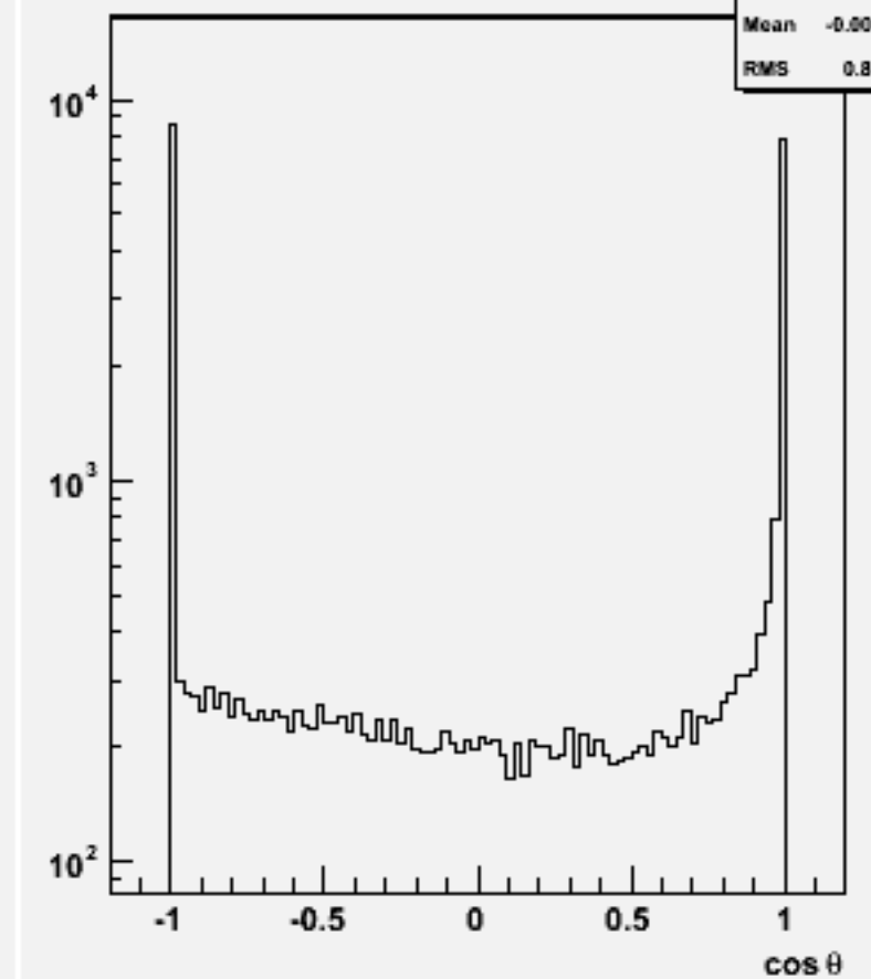
Jet cos \theta (All jets)w103178 e1a_e1n3e3e3n3_o
