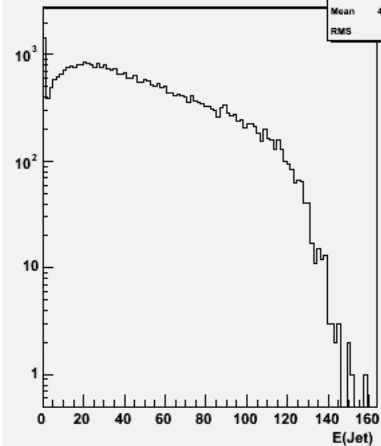
Jet energies(All jets)w103178 e1a_e1n3e3e3n3_o
