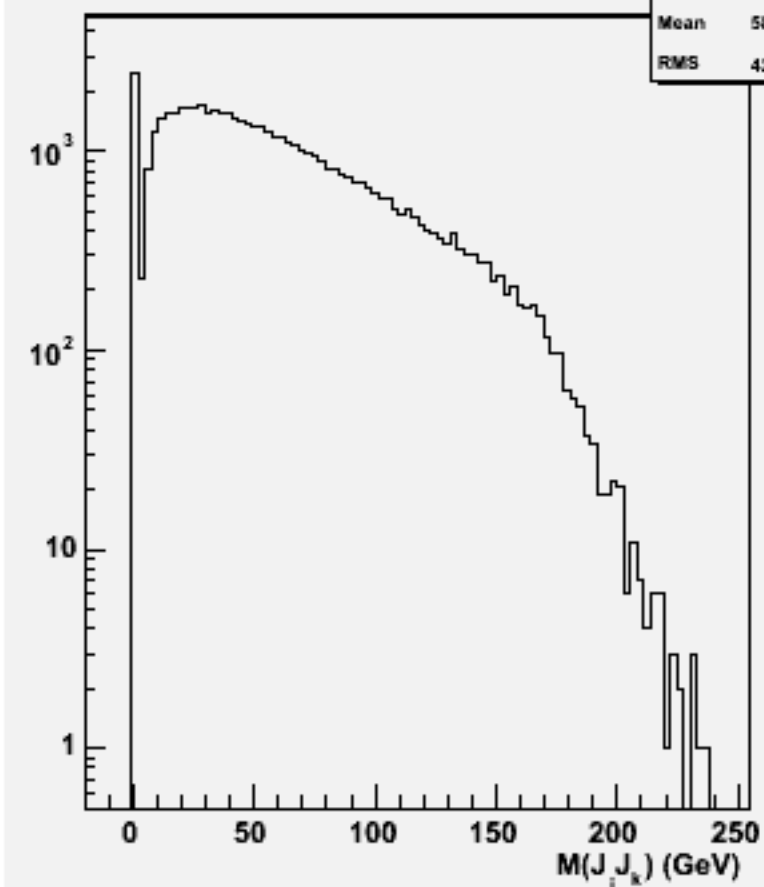
2jets mass(All comb)w103178 e1a_e1n3e3e3n3_o
