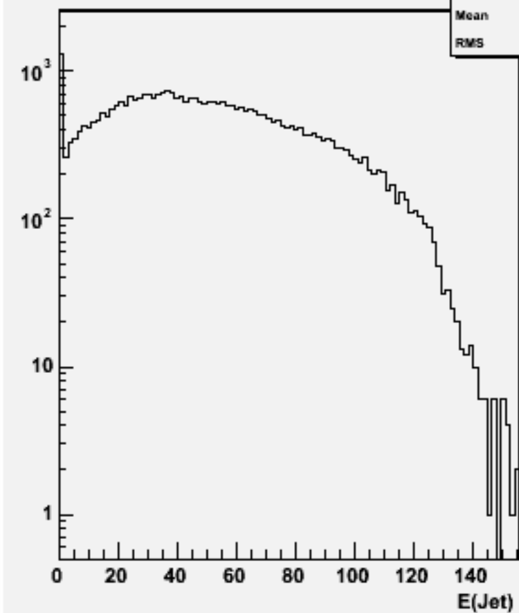
Jet energies(All jets)w103176 e1a_e1n3e3e2n2_o
