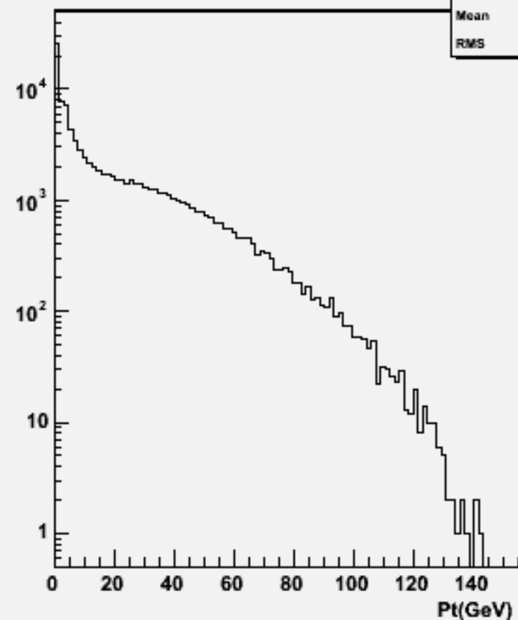
Start point Z : w103176 e1a_e1n3e3e2n2_o
