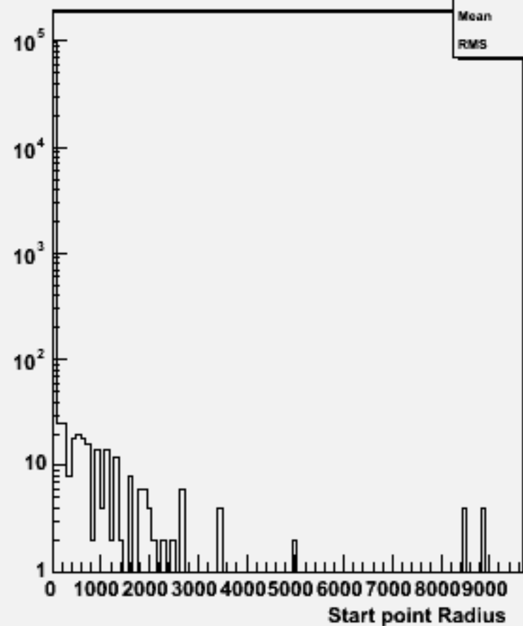
Start point R : w103176 e1a_e1n3e3e2n2_o
