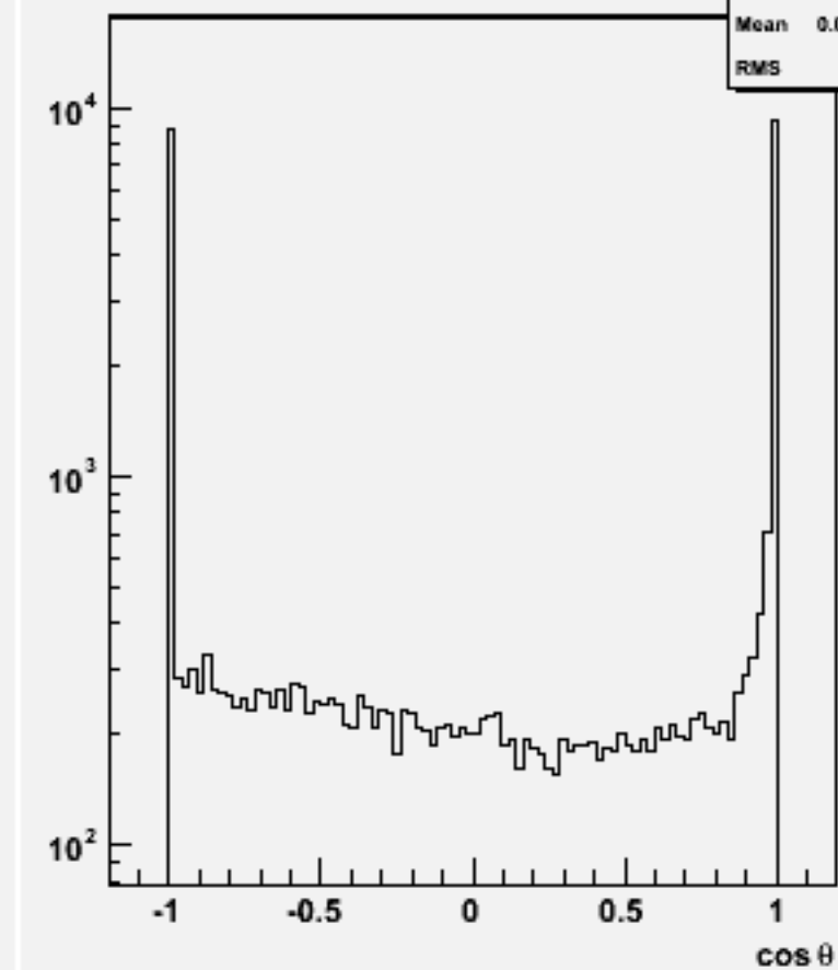
Jet cos \theta (All jets)w103176 e1a_e1n3e3e2n2_o
