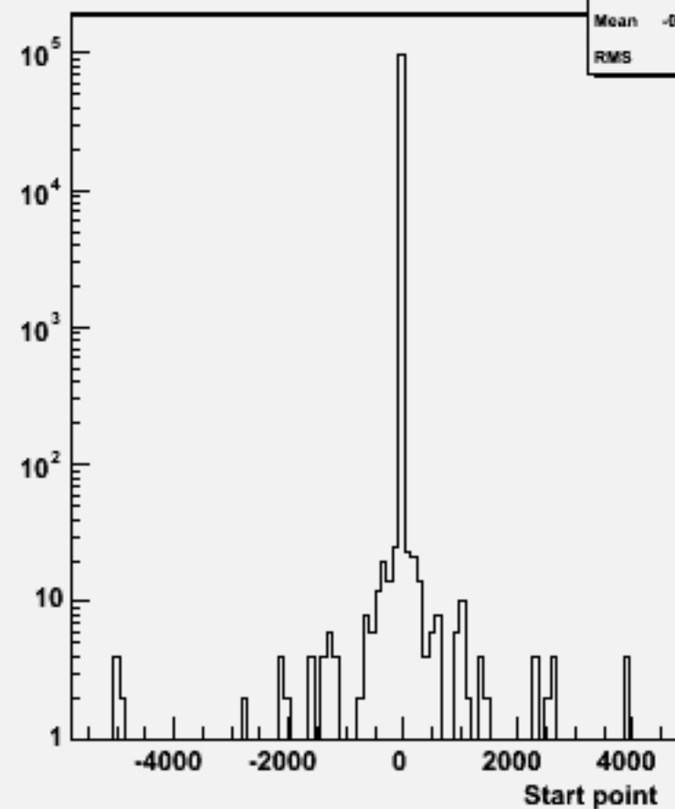
Start point Z : w103176 e1a_e1n3e3e2n2_o
