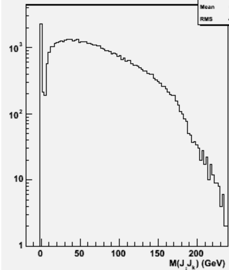
2jets mass(All comb)w103176 e1a_e1n3e3e2n2_o
