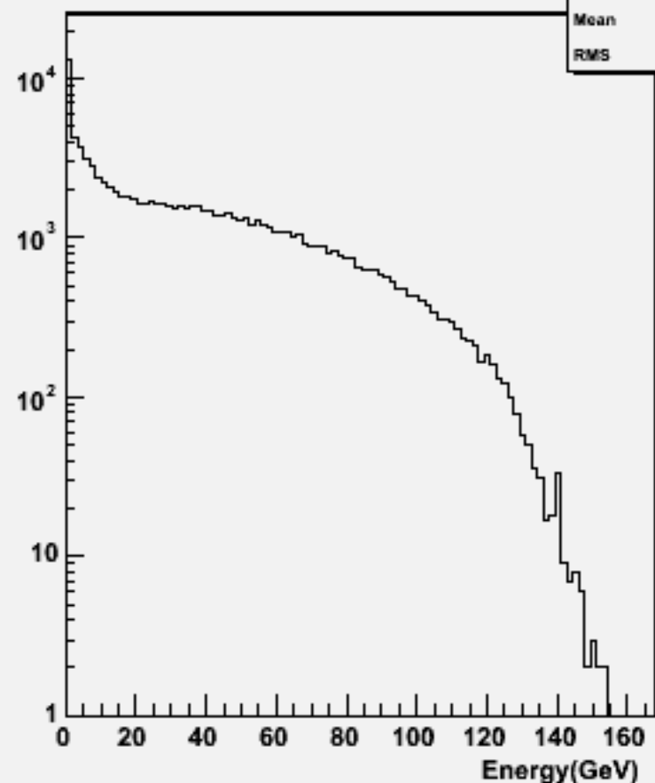
Start point R : w103176 e1a_e1n3e3e2n2_o
