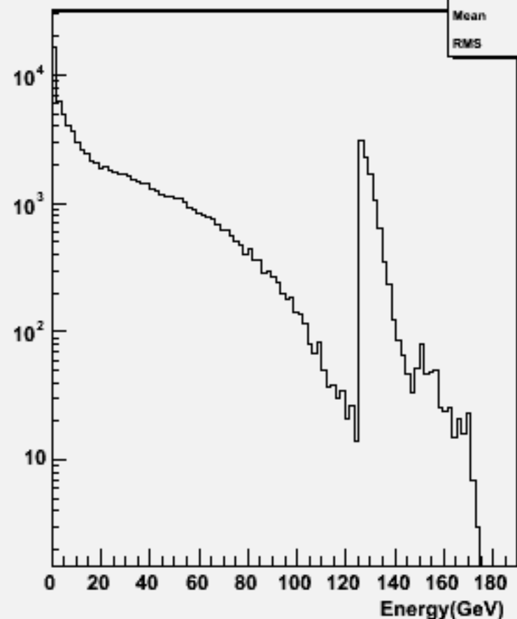
Start point R : w103175 e1a_e1n3e3e2n2_o
