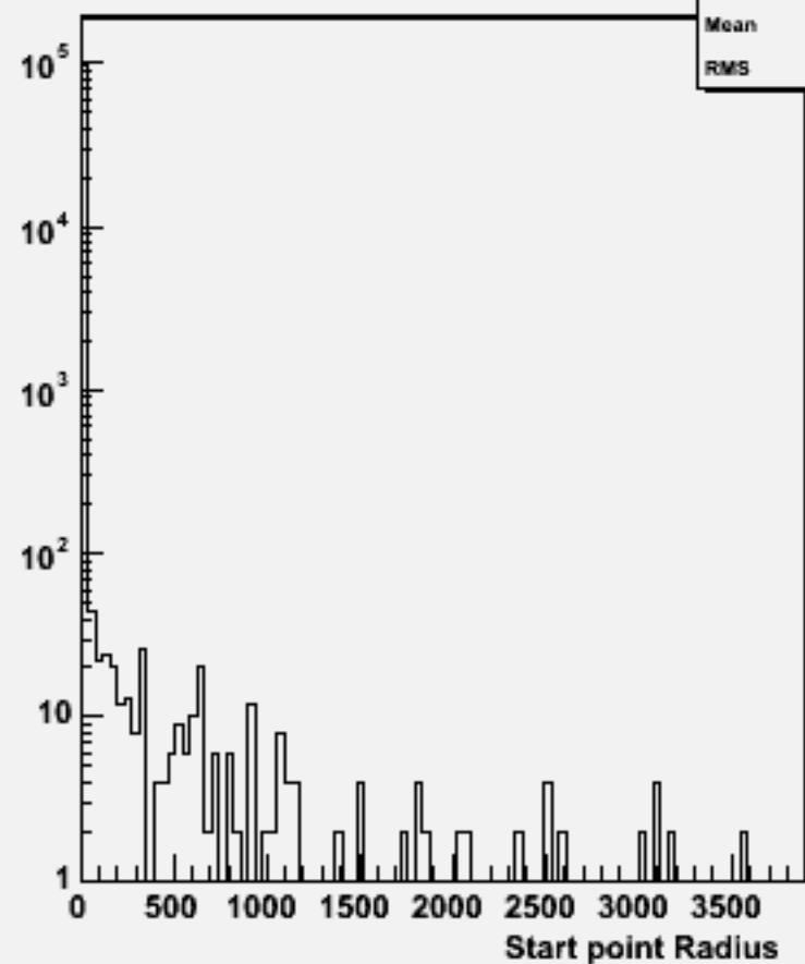
Start point R : w103175 e1a_e1n3e3e2n2_o
