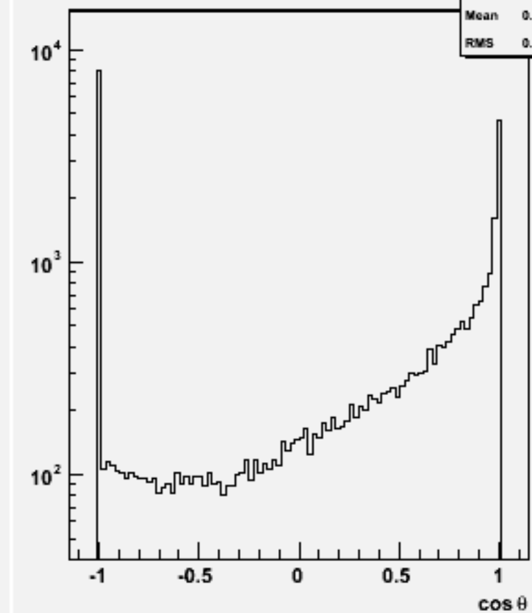
Jet cos \theta (All jets)w103175 e1a_e1n3e3e2n2_o
