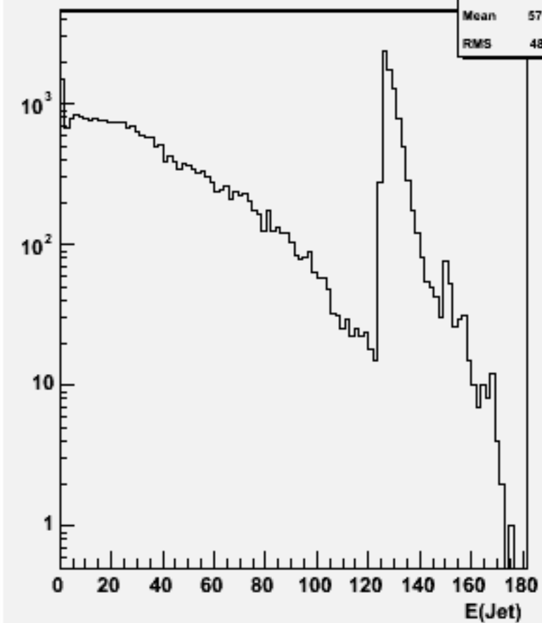
Jet energies(All jets)w103175 e1a_e1n3e3e2n2_o
