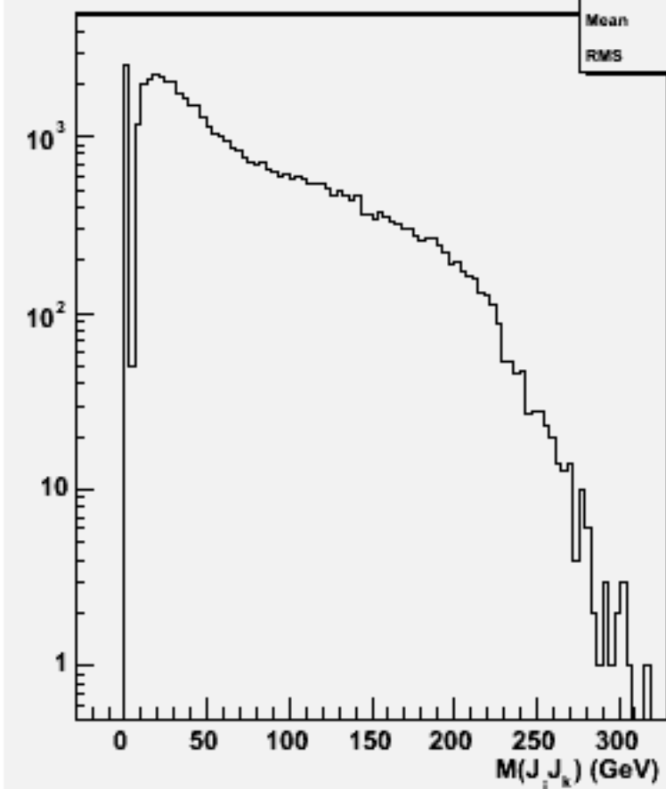
2jets mass(All comb)w103175 e1a_e1n3e3e2n2_o
