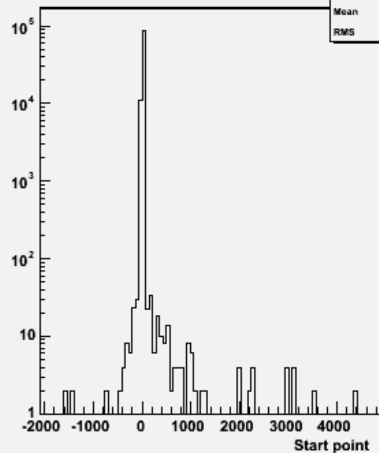
Start point Z : w103175 e1a_e1n3e3e2n2_o
