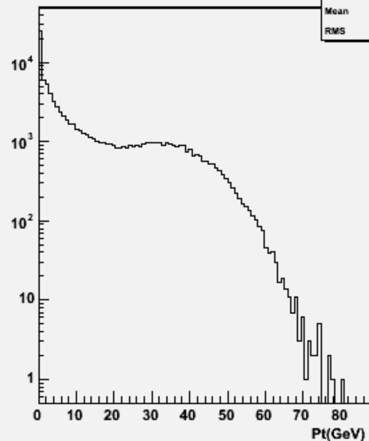
Start point Z : w103175 e1a_e1n3e3e2n2_o
