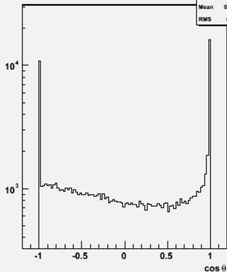
Particle cos \theta : w103174 e1a_e1n3e3e2n2_o
