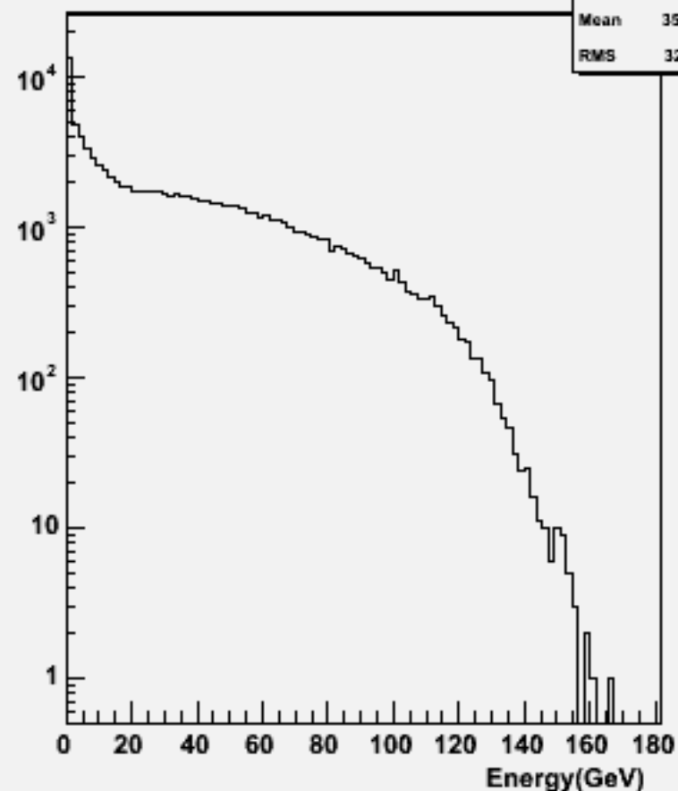
Start point R : w103174 e1a_e1n3e3e2n2_o
