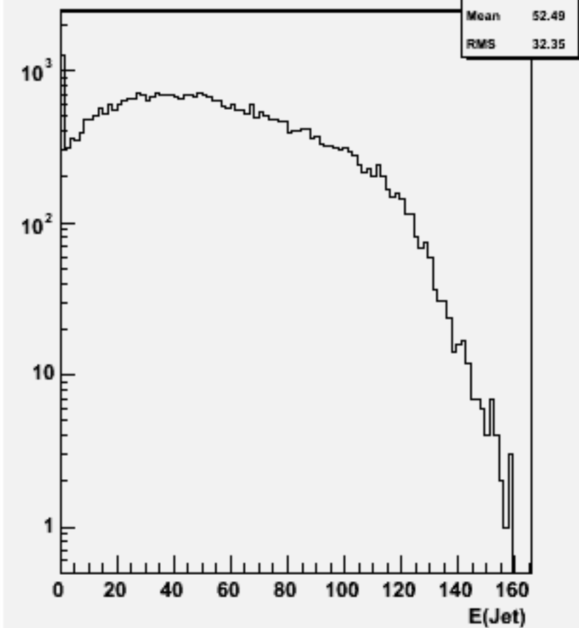
Jet energies(All jets)w103174 e1a_e1n3e3e2n2_o
