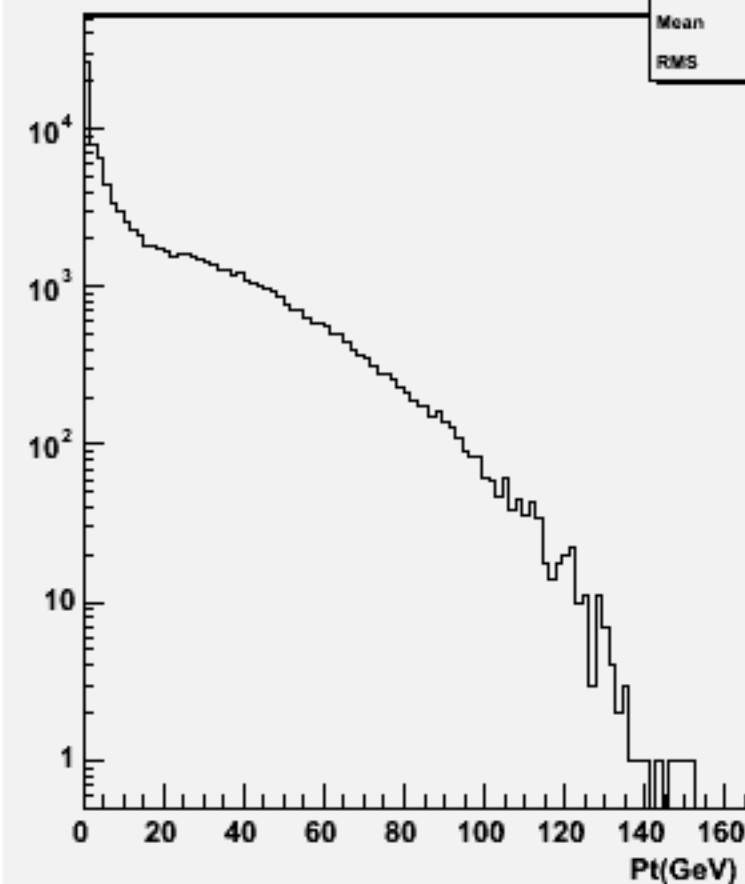
Start point Z : w103174 e1a_e1n3e3e2n2_o
