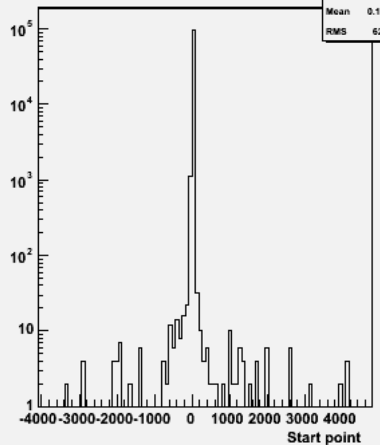
Start point Z : w103172 e1a_e1n3e3e1n1_o
