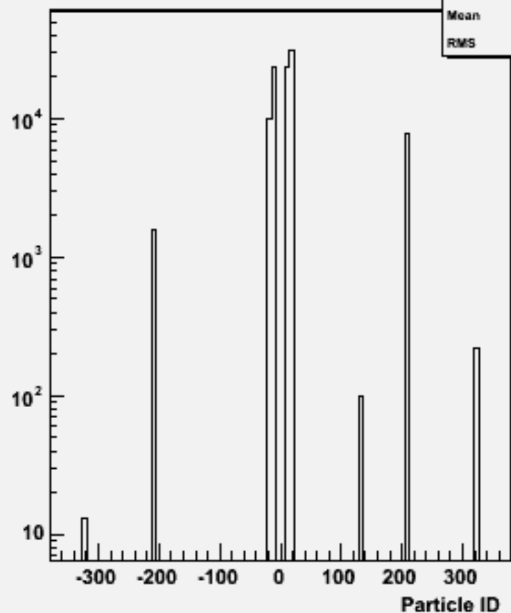
Particle ID : w103172 e1a_e1n3e3e1n1_o
