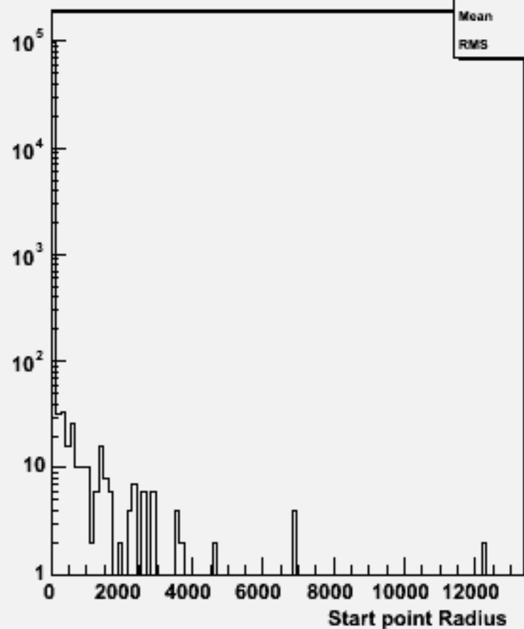
Start point R : w103172 e1a_e1n3e3e1n1_o
