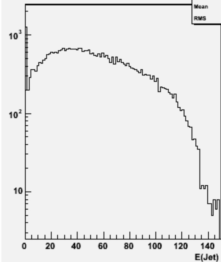
Jet energies(All jets)w103172 e1a_e1n3e3e1n1_o
