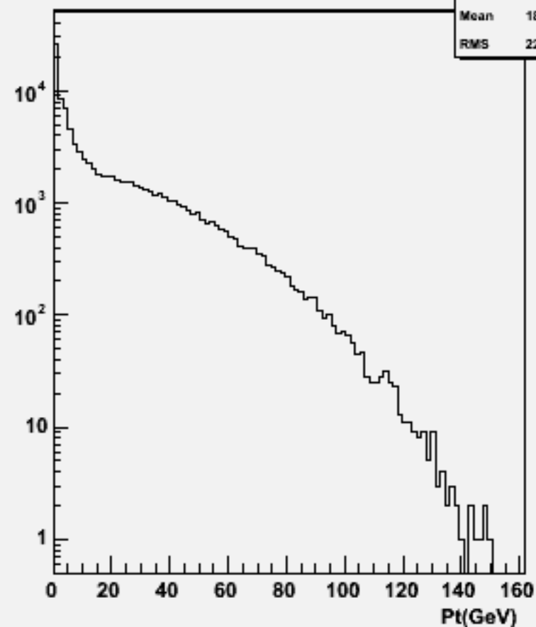
Particle Pt : w103172 e1a_e1n3e3e1n1_o
