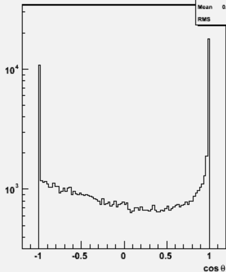
Particle cos \theta : w103172 e1a_e1n3e3e1n1_o
