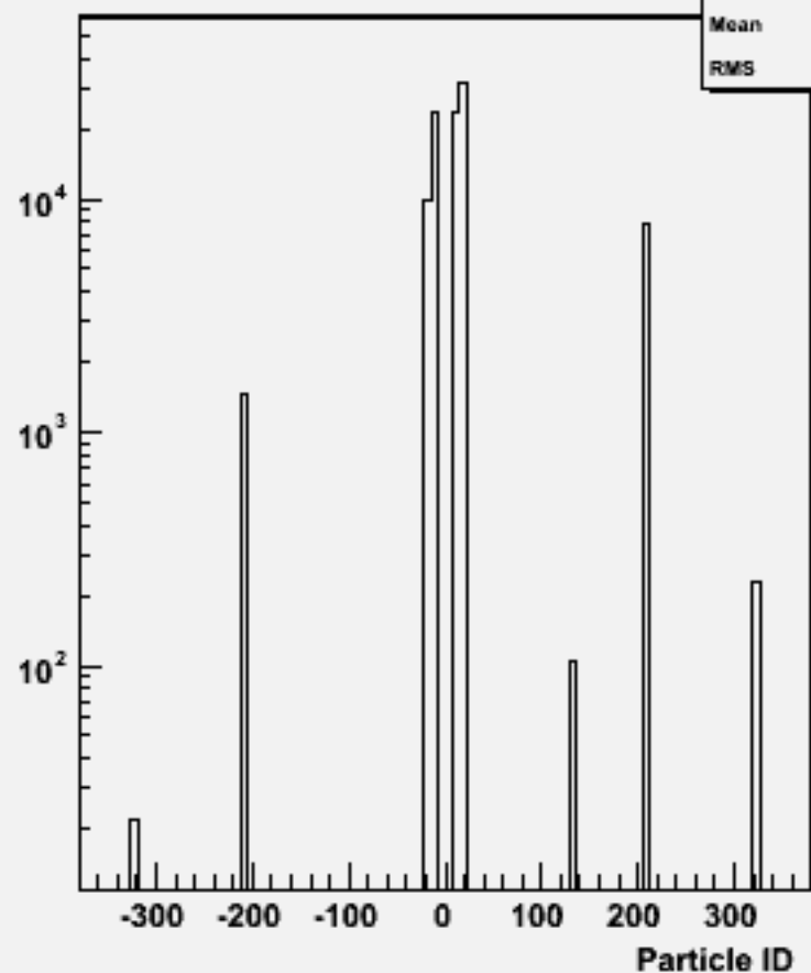
Particle ID : w103170 e1a_e1n3e3e1n1_o
