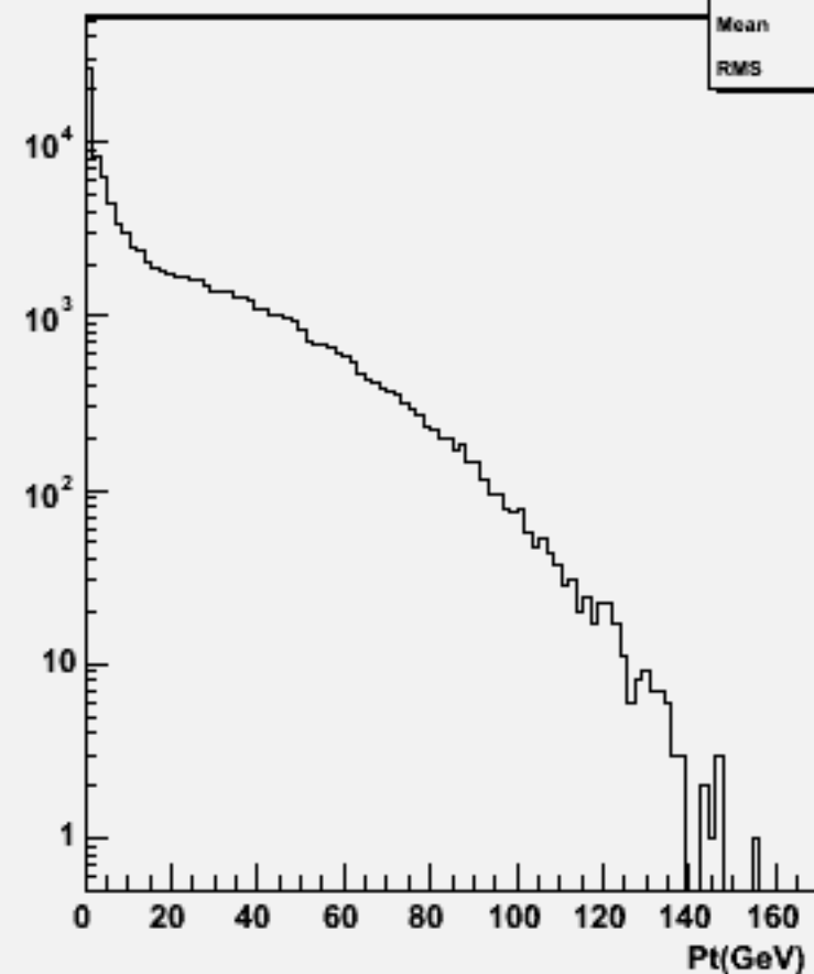
Particle Pt : w103170 e1a_e1n3e3e1n1_o
