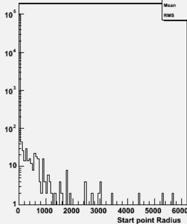
Start point R : w103170 e1a_e1n3e3e1n1_o
