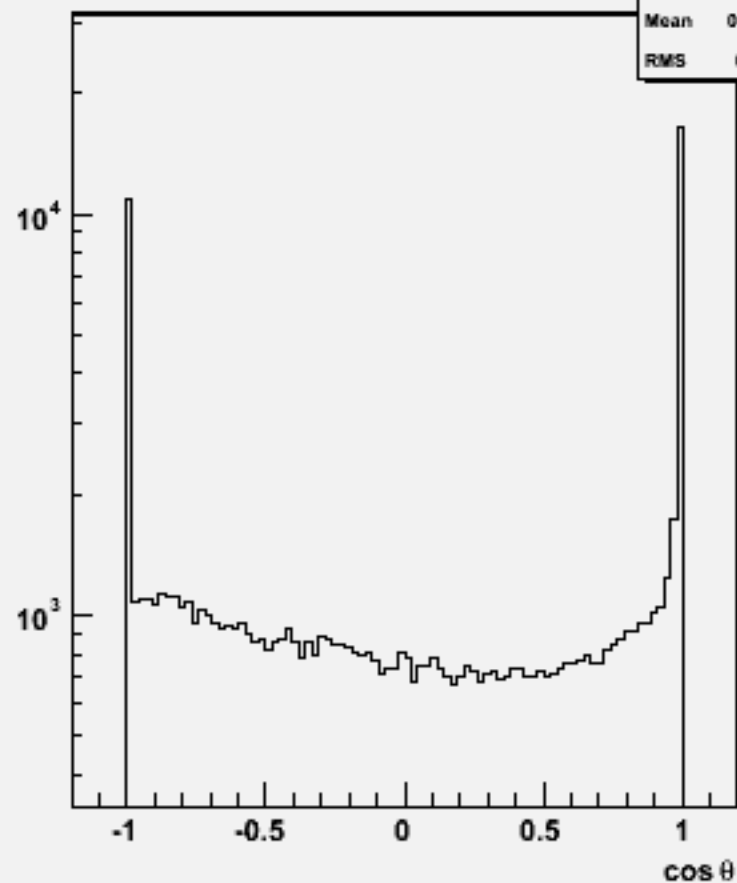
Particle cos \theta : w103170 e1a_e1n3e3e1n1_o
