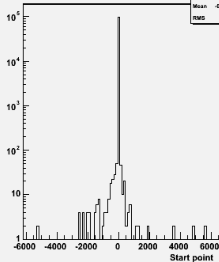
Start point Z : w103170 e1a_e1n3e3e1n1_o
