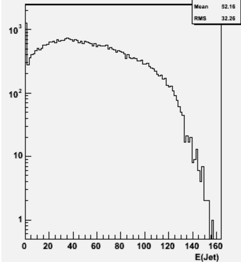
Jet energies(All jets)w103170 e1a_e1n3e3e1n1_o
