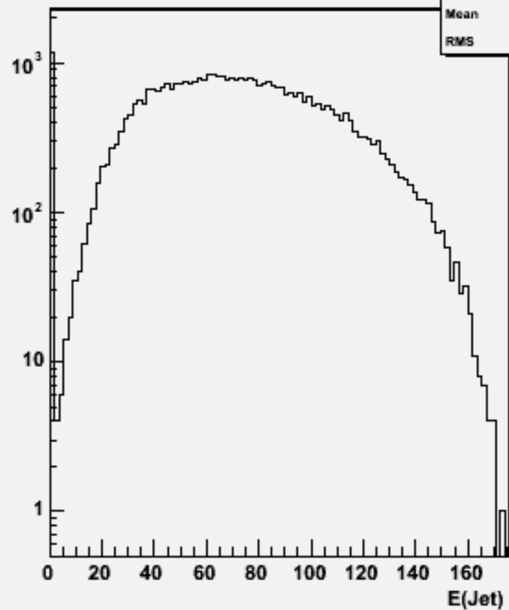
Jet energies(All jets)w103168 e1a_e1n2e2sc_o
