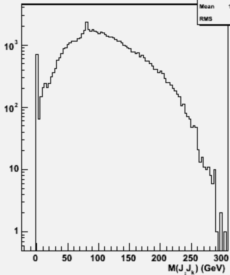
2jets mass(All comb)w103168 e1a_e1n2e2sc_o
