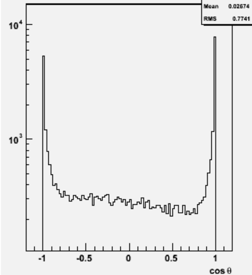
Jet cos theta (All jets)w103168 e1a_e1n2e2sc_o
