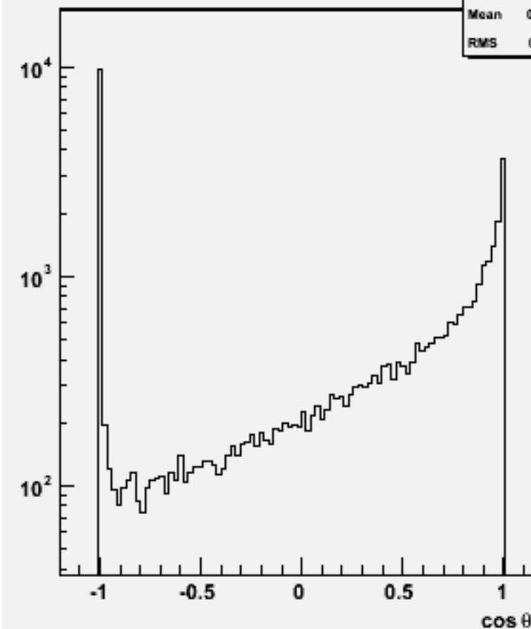
Jet cos \theta (All jets)w103163 e1a_e1n2e2du_o
