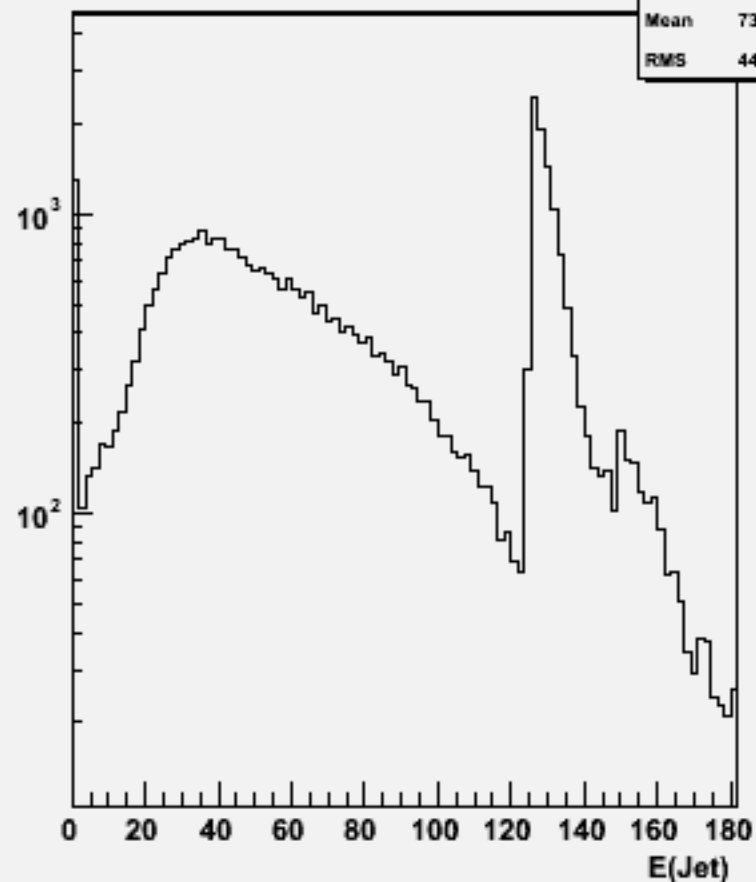
Jet energies(All jets)w103163 e1a_e1n2e2du_o
