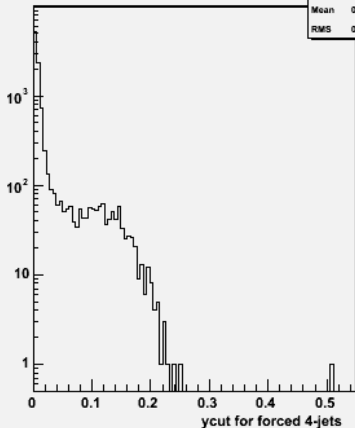
Ycut for 4-jets :w103163 e1a_e1n2e2du_o
