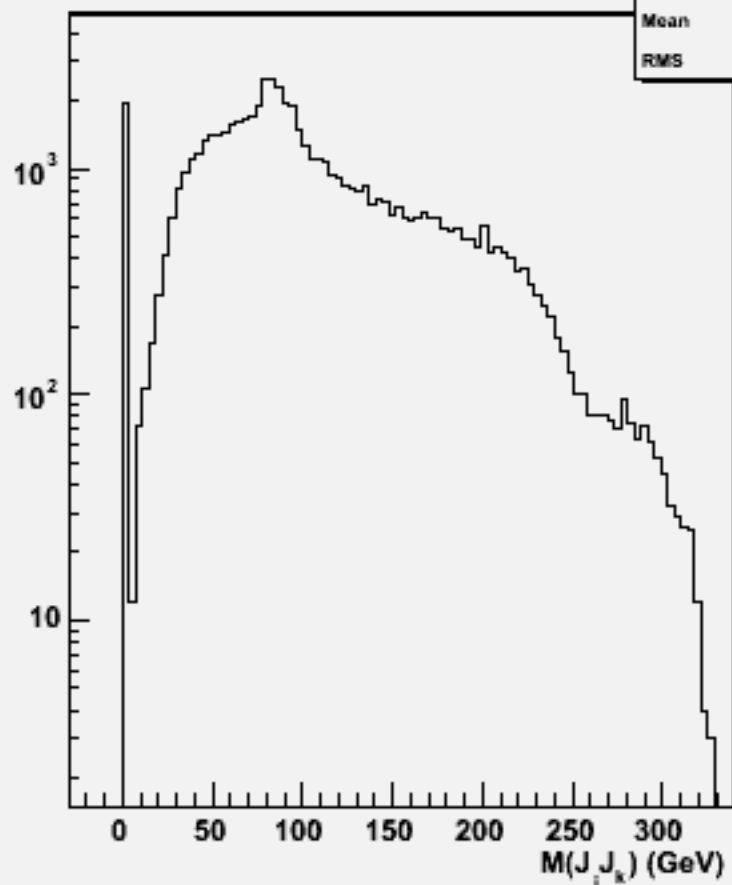
2jets mass(All comb)w103163 e1a_e1n2e2du_o
