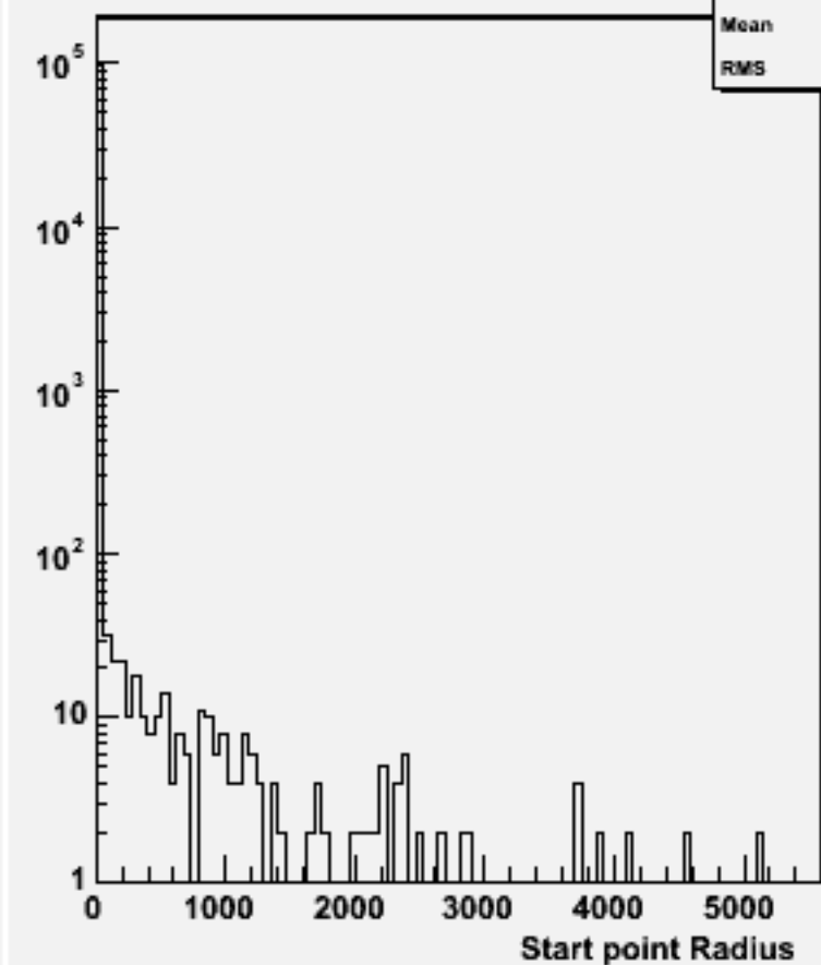
Start point R : w103160 e1a_e1n2e2e3n3_o
