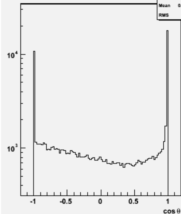
Particle cos \theta : w103160 e1a_e1n2e2e3n3_o
