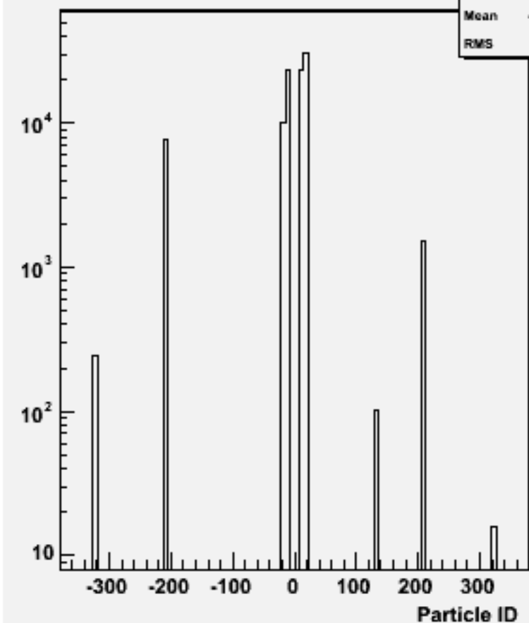
Particle ID : w103160 e1a_e1n2e2e3n3_o
