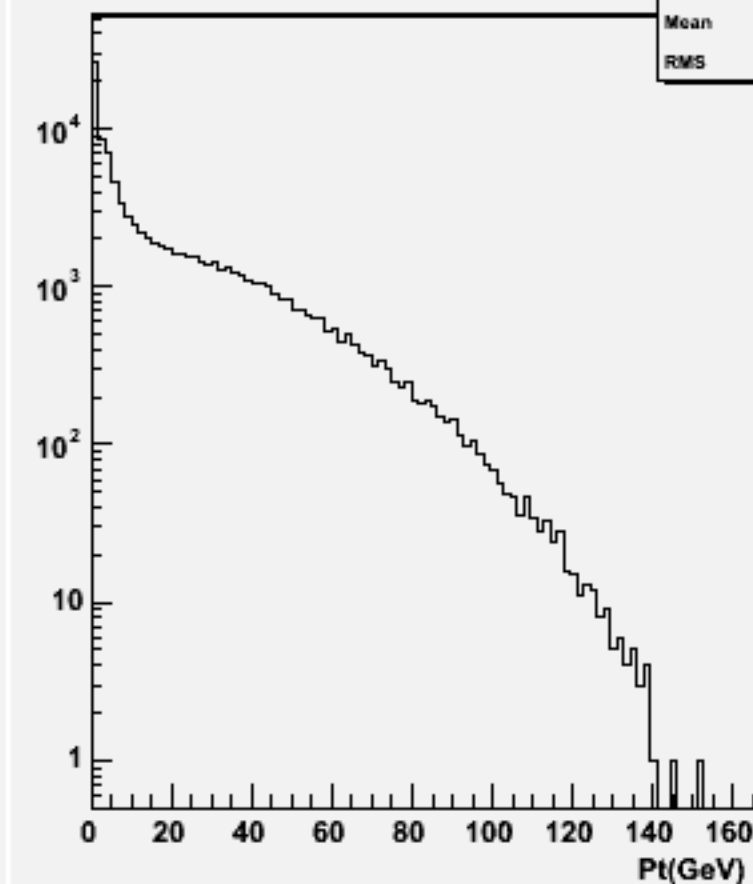
Particle Pt : w103160 e1a_e1n2e2e3n3_o
