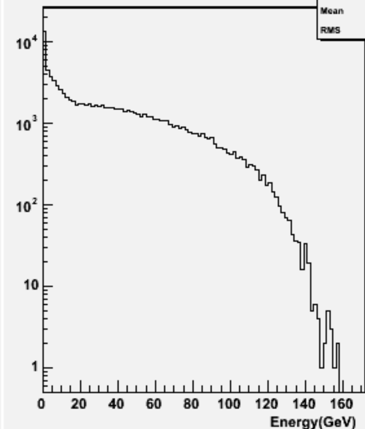
Particle Energy : w103160 e1a_e1n2e2e3n3_o
