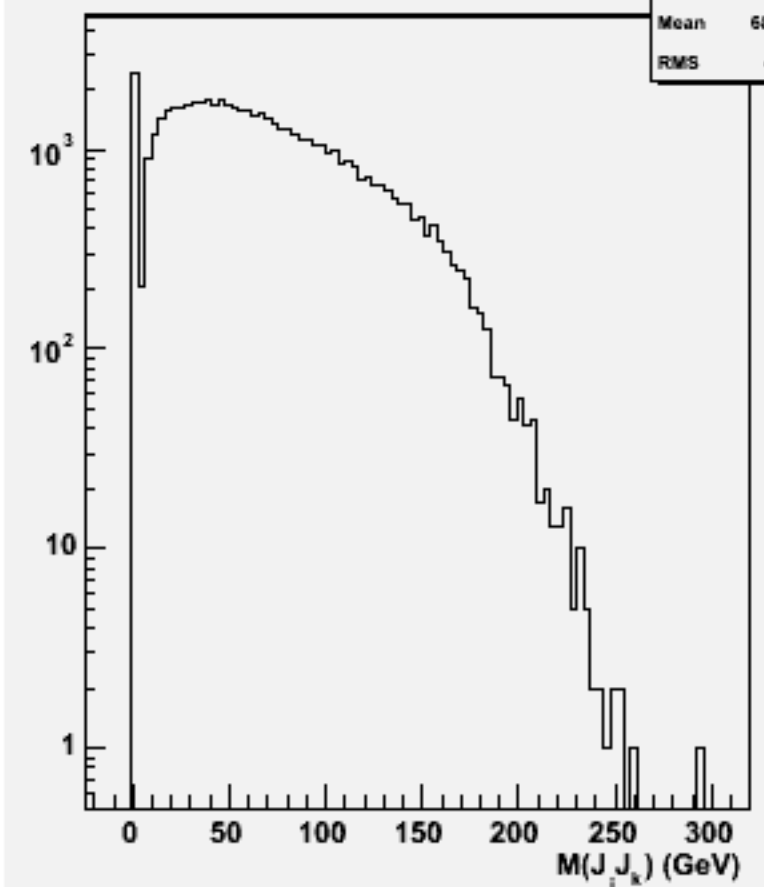
2jets mass(All comb)w103160 e1a_e1n2e2e3n3_o
