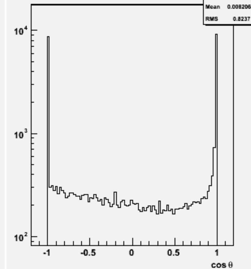
Jet cos \theta (All jets)w103160 e1a_e1n2e2e3n3_o
