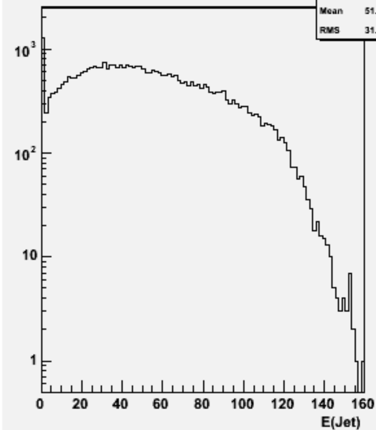
Jet energies(All jets)w103160 e1a_e1n2e2e3n3_o
