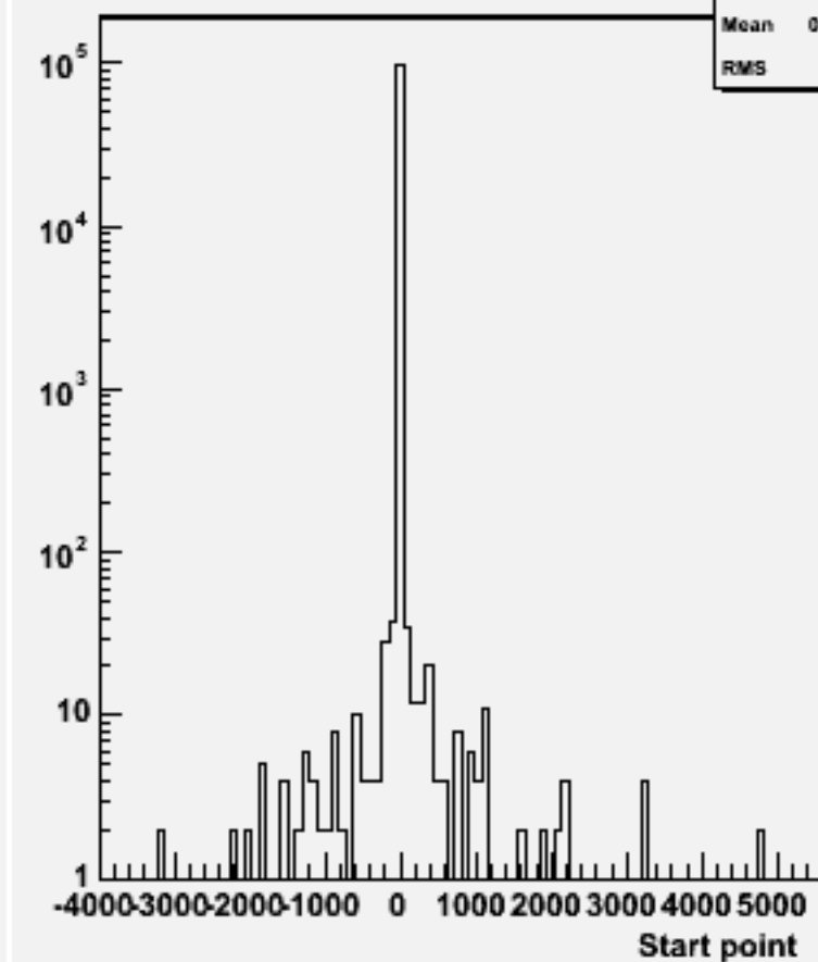
Start point Z : w103160 e1a_e1n2e2e3n3_o
