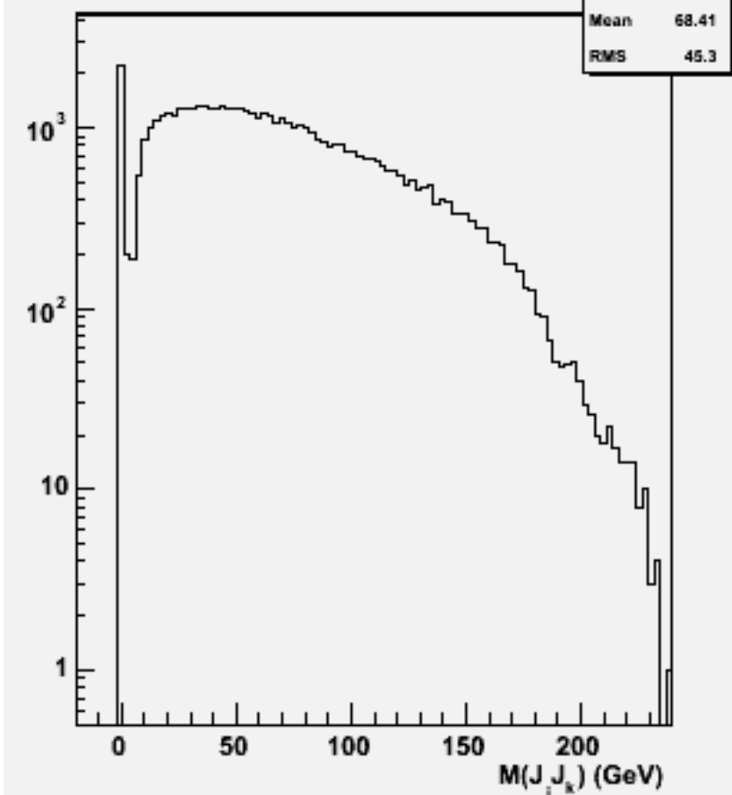
2jets mass(All comb)w103158 e1a_e1n2e2e3n3_o
