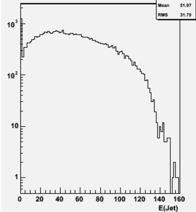
Jet energies(All jets)w103158 e1a_e1n2e2e3n3_o
