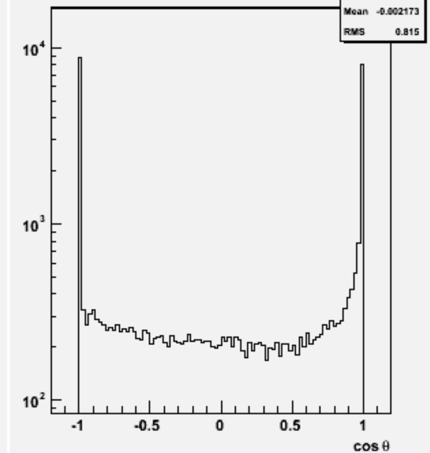
Jet cos \theta (All jets)w103158 e1a_e1n2e2e3n3_o
