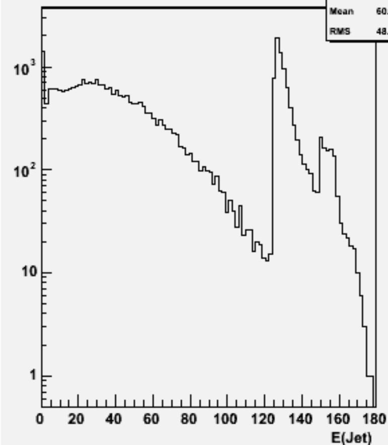
Jet energies(All jets)w103157 e1a_e1n2e2e2n2_o
