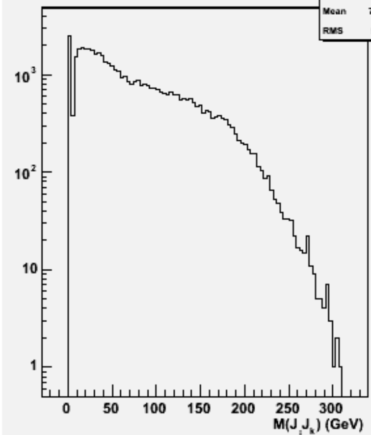
2jets mass(All comb)w103157 e1a_e1n2e2e2n2_o
