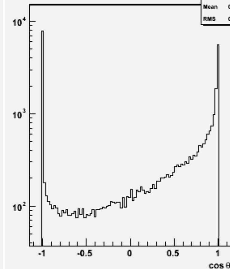
Jet cos \theta (All jets)w103157 e1a_e1n2e2e2n2_o
